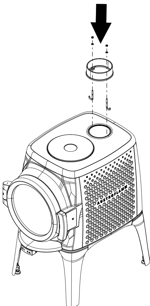
Fig. 6: Montaggio della presa della canna fumaria
