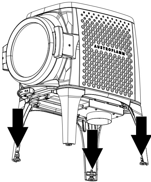
Fig. 11: Allineamento della stufa
