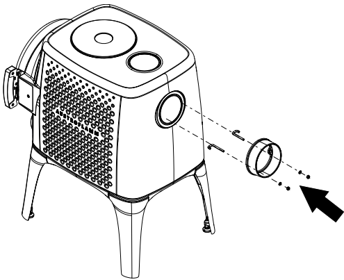
Fig. 8: Montaggio della presa della canna fumaria posteriore
