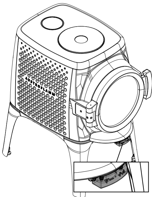
Fig. 2: Regolatore dell'aria
