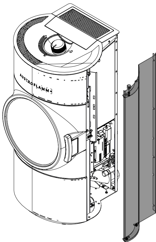
Fig. 23: Déposer l'habillage latéral
