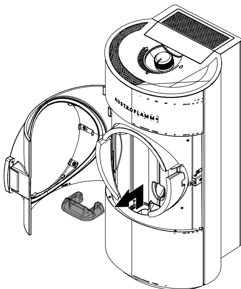
Fig. 26: Enlever la pierre en Keramott
