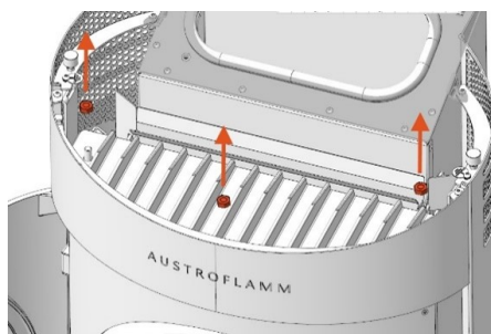
Fig. 31: Dévisser les vis de fixation
