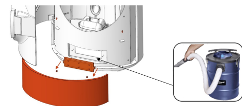
Fig. 33: Aspirer la zone des fumées
