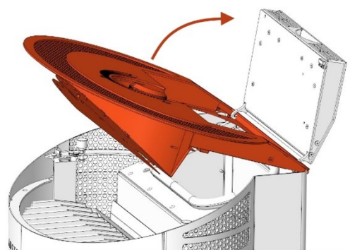
Fig. 30: Relever le couvercle de révision
