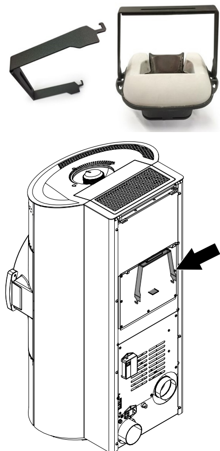
Fig. 25: Outil de levage
