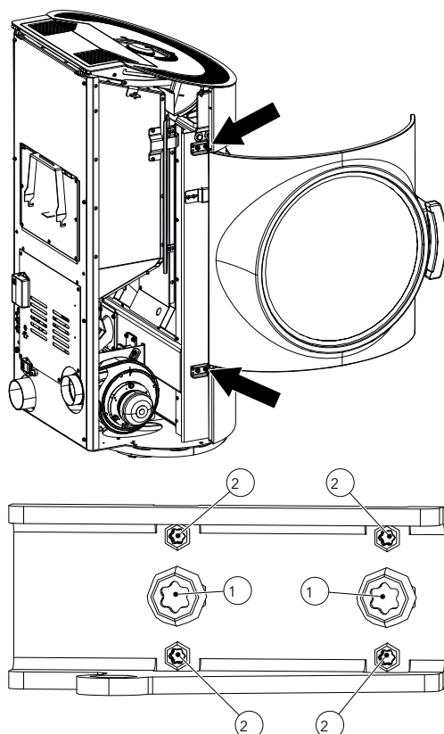
Fig. 18: Vis de réglage de la porte
