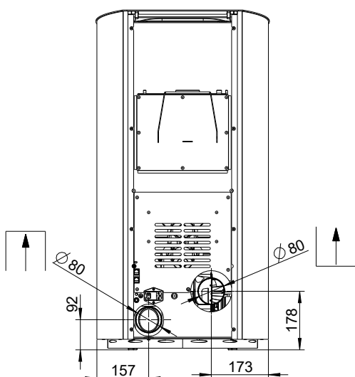
Fig. 9: Raccord par l'arrière
