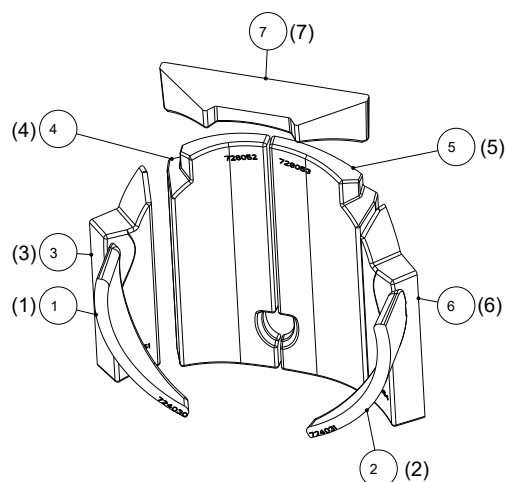
Fig. 8: Installer la Keramott
