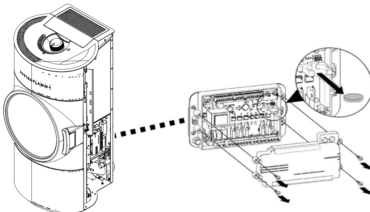
Fig. 24: Remplacer la pile mémoire
