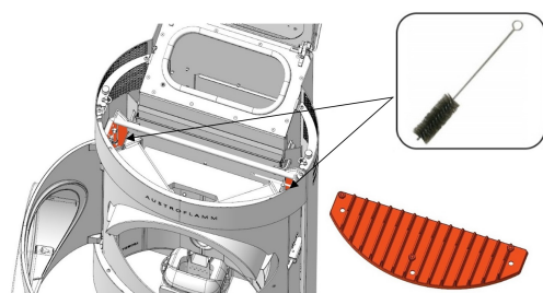
Fig. 32: Brosser le circuit de fumées
