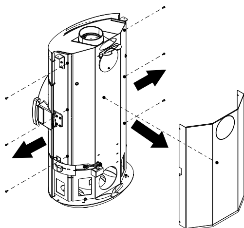
Fig. 17: Démonter le recouvrement
