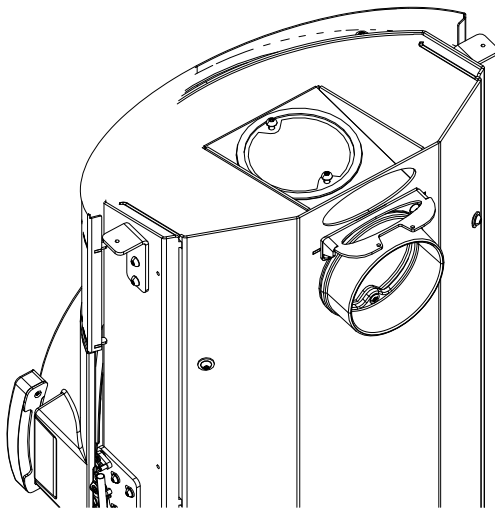
Fig. 20: Recouvrement et tubulure échangés
