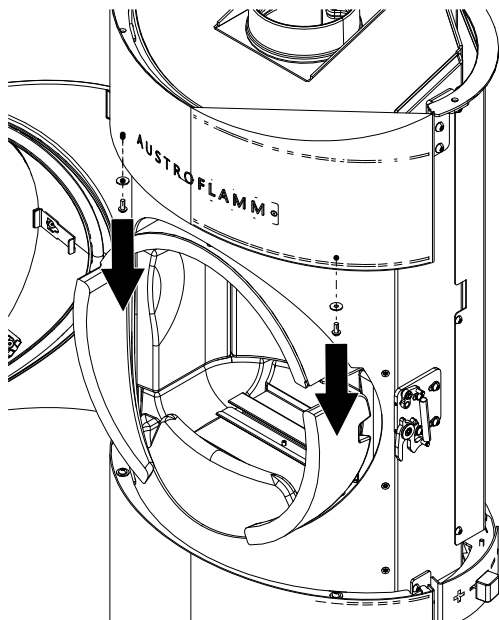
Fig. 12: Dévisser les vis
