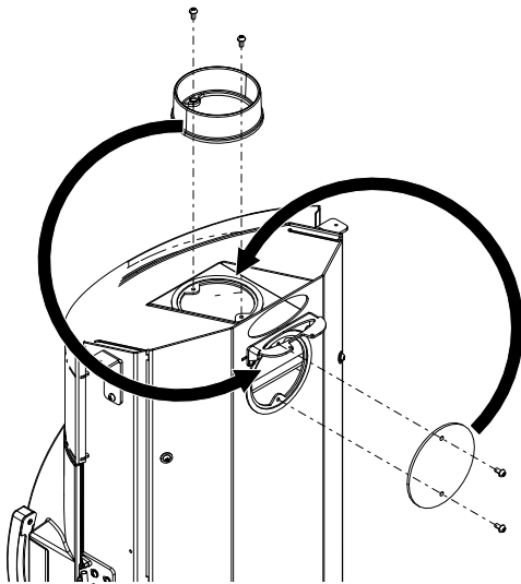
Fig. 19: Échanger le recouvrement et la tubulure
