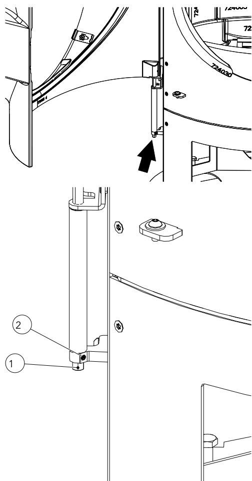
Fig. 32: Régler la force de fermeture de la porte
