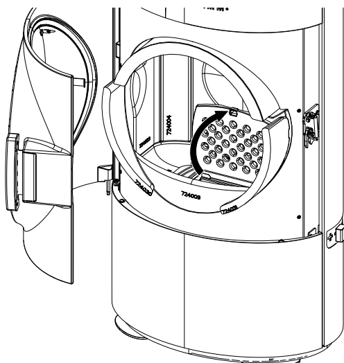
Fig. 37: Relever la grille
