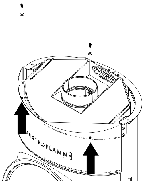
Fig. 11: Dévisser les vis de l'habillage avant supérieur.
