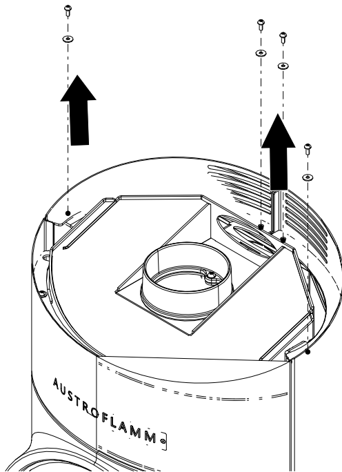
Fig. 9: Dévisser les vis
