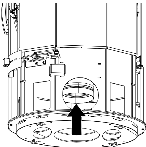
Fig. 23: Fixer le tuyau flexible en alu
