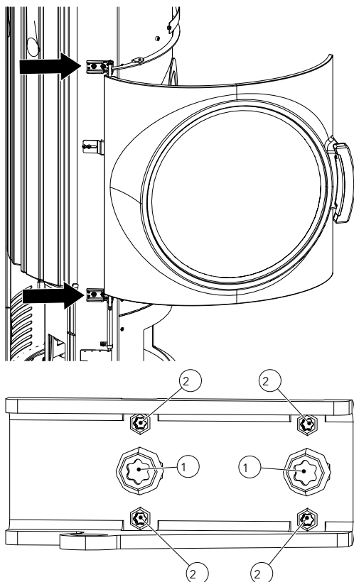
Fig. 29: Vis de réglage de la porte
