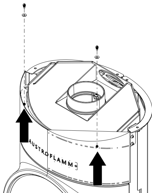
Fig. 26: Dévisser les vis
