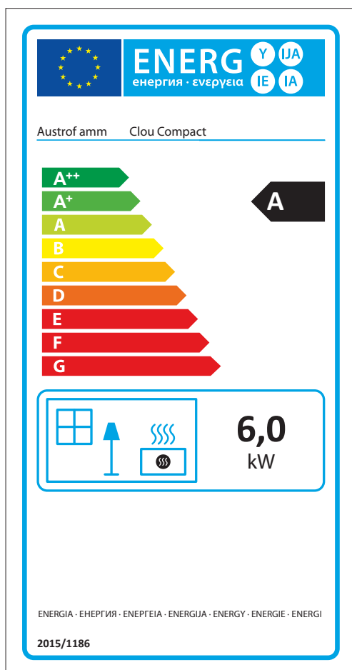
Fig. 4: Label énergétique
