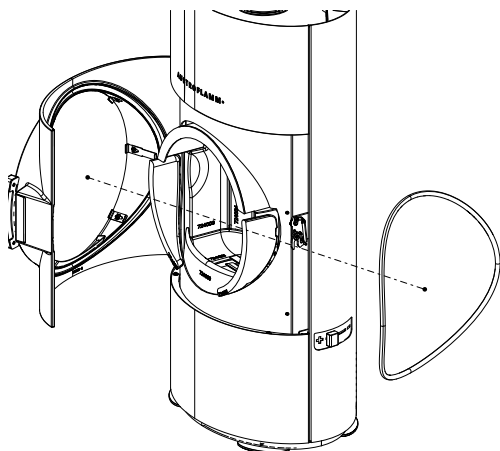
Fig. 36: Remplacer le joint
