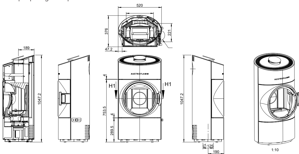
Fig. 1: Dimensions
