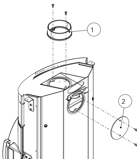
Fig. 18: Démonter la tubulure de fumées et le recouvrement
