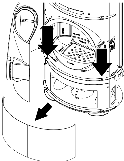
Fig. 31: Déposer l'habillage avant inférieur
