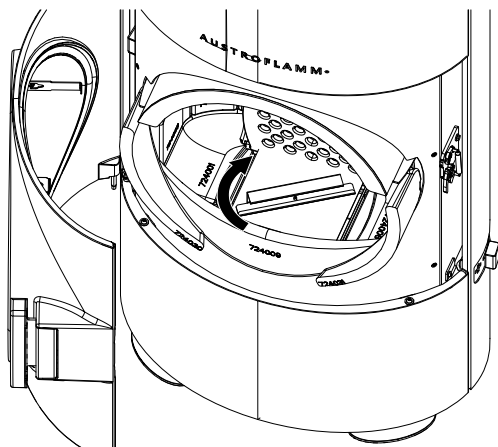
Fig. 38: Mettre le couvercle sur le bac à cendres
