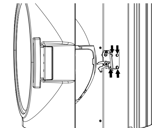
Fig. 30: Régler la serrure de la porte
