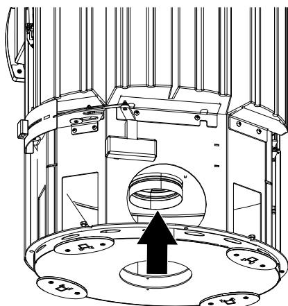
Fig. 12: Fixer le tuyau flexible en alu
