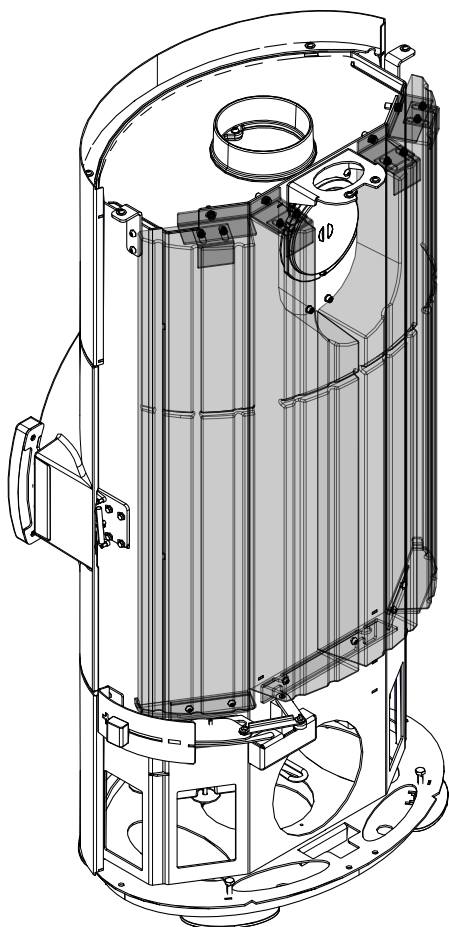
Fig. 13: Installer l'HMS
