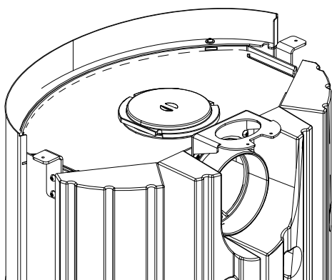
Fig. 9: Recouvrement et tubulure échangés
