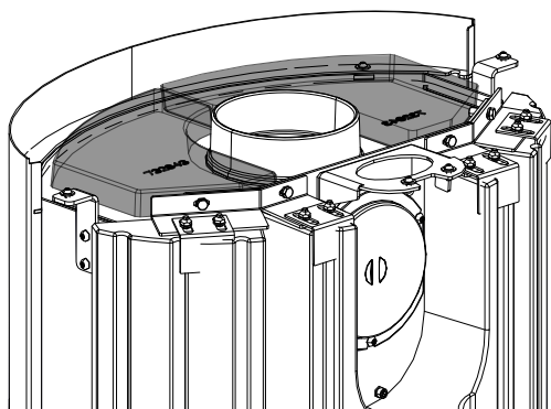
Fig. 15: Fixer les pierres HMS en haut.
