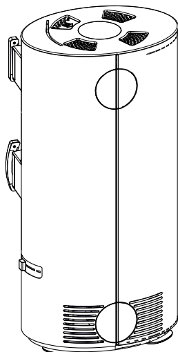
Fig. 16: Remettre l'habillage latéral et le couvercle en place
