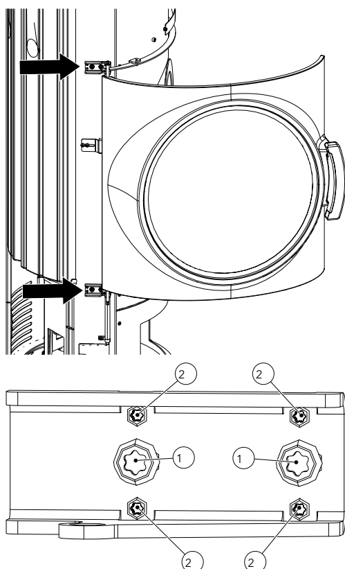
Fig. 22: Vis de réglage de la porte
