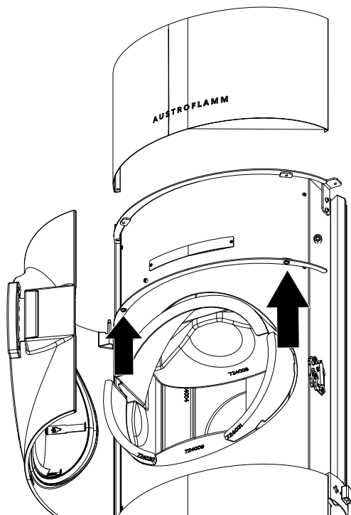
Fig. 20: Déposer l'habillage avant supérieur
