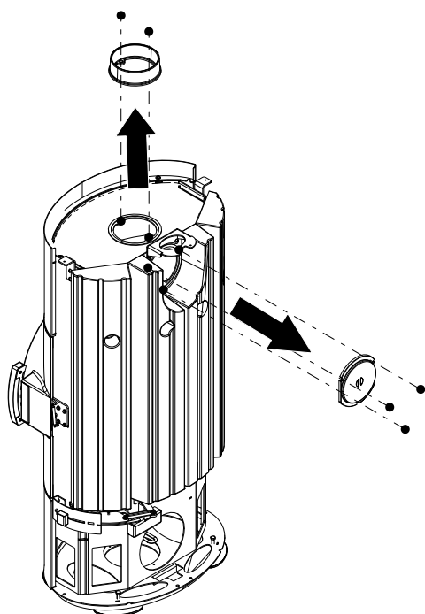
Fig. 7: Démonter le recouvrement et la tubulure de fumées
