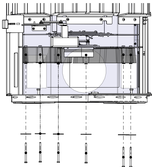
Fig. 14: Monter les pierres HMS en bas
