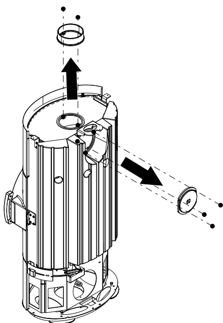
Fig. 7: Smontaggio del coperchio e della presa della canna fumaria
