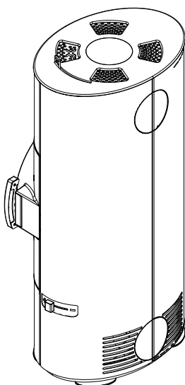
Fig. 10: Montaggio del rivestimento laterale e posizionamento del coperchio
