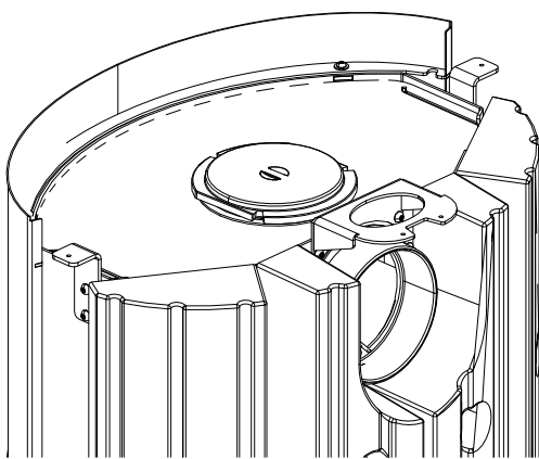
Fig. 9: Copertura e pezzo di collegamento sostituiti
