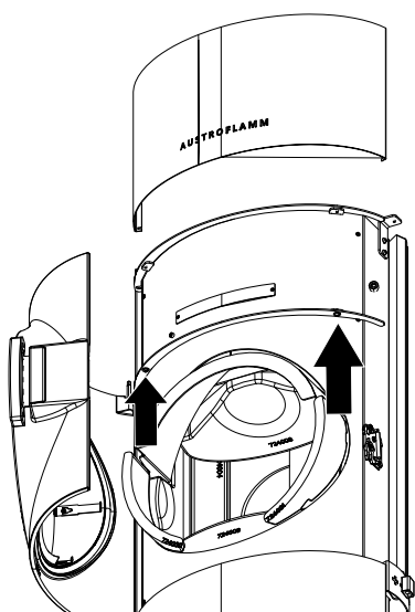
Fig. 20: Smontaggio del rivestimento anteriore superiore
