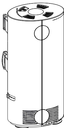
Fig. 16: Collocazione del rivestimento laterale e del coperchio
