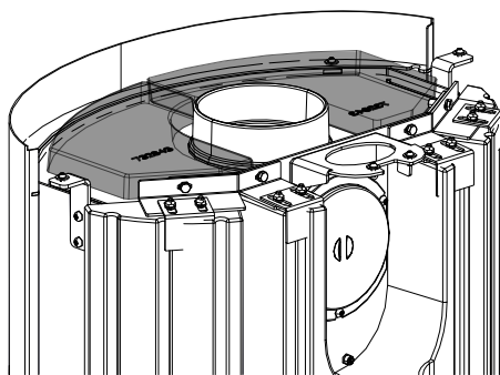
Fig. 15: Attaccare le pietre HMS in alto.
