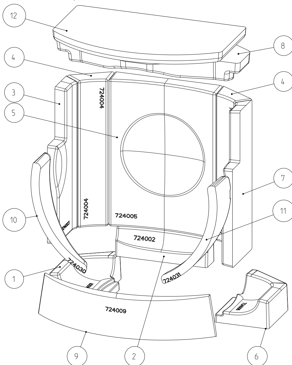
Fig. 17: Keramott
