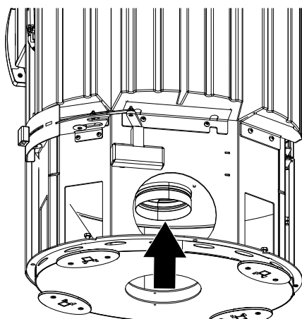
Fig. 12: Fissaggio del tubo Aluflex
