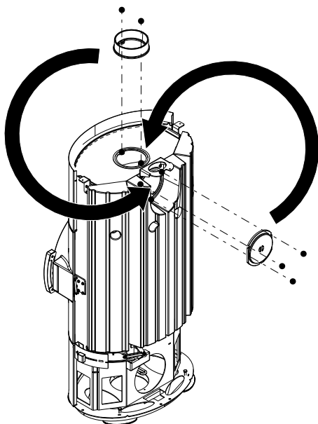
Fig. 8: Sostituzione della copertura e del pezzo di collegamento
