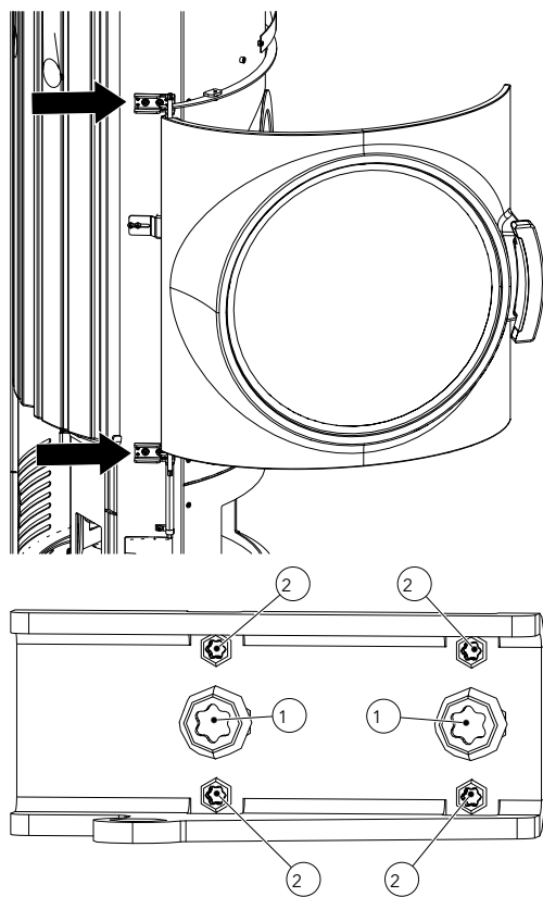
Fig. 22: Viti di registro dello sportello
