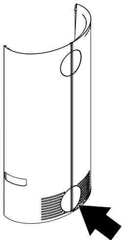
Fig. 11: Rimozione della parte perforata
