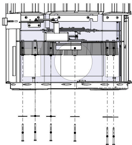
Fig. 14: Montare le pietre HMS in basso
