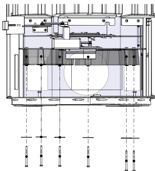
Fig. 42: Montare le pietre HMS in basso
