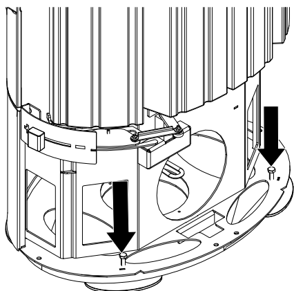
Fig. 18: Allineamento della stufa
