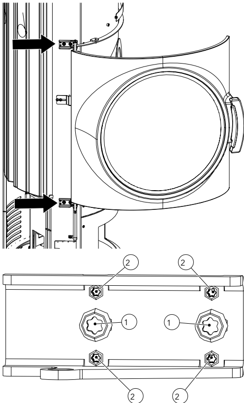
Fig. 19: Vis de réglage de la porte
