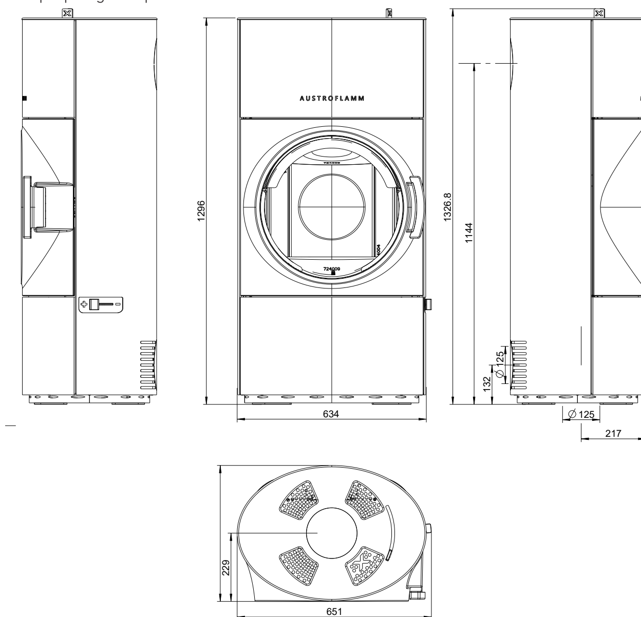
Fig. 1: Dimensions de l'appareil de base
