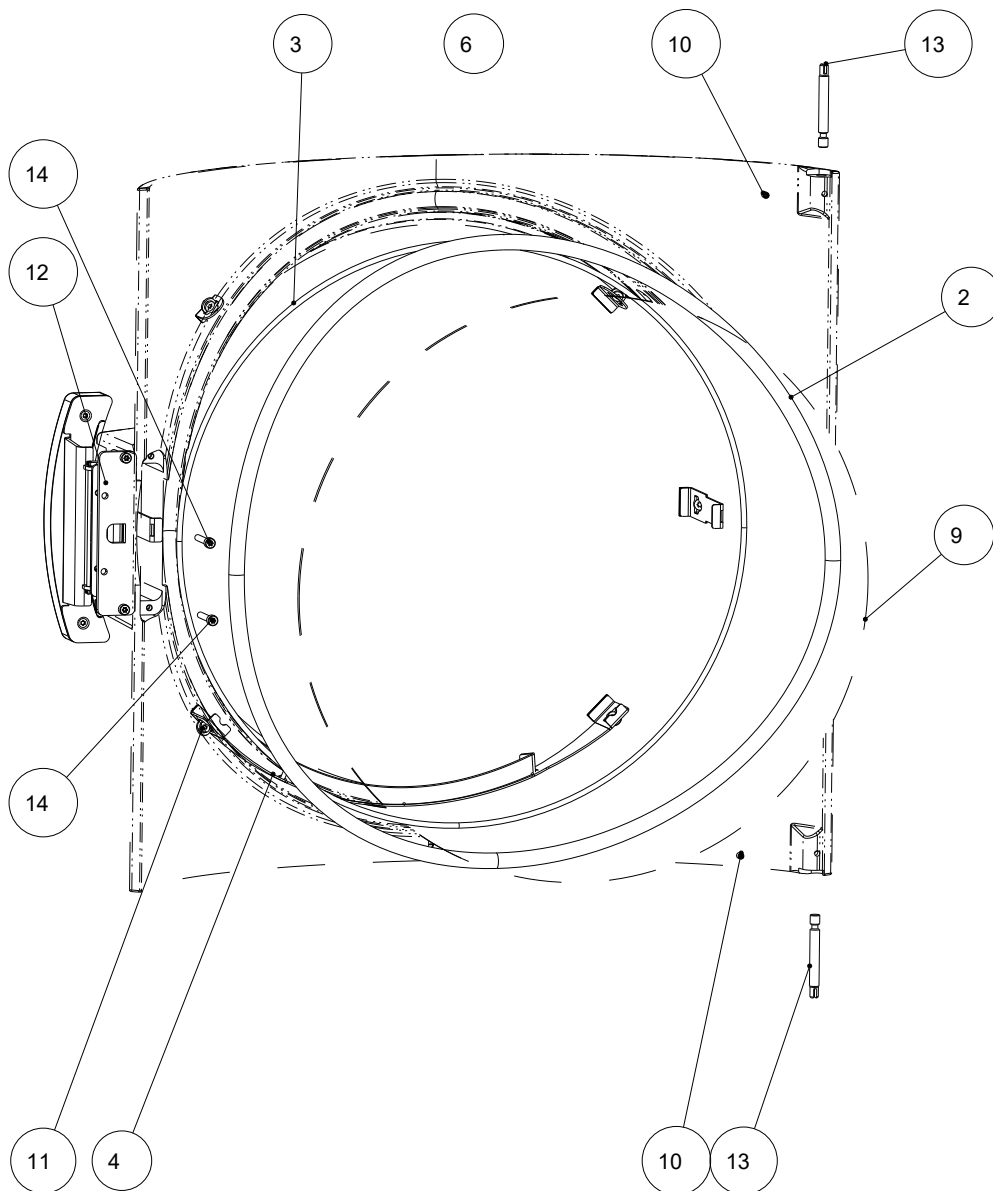
Fig. 38: Porte de la chambre de combustion
