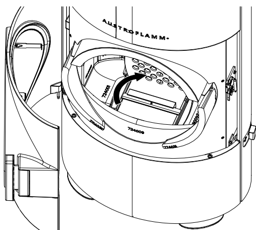
Fig. 31: Fermer le couvercle
