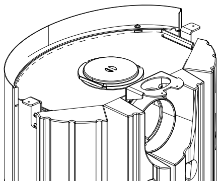
Fig. 11: Recouvrement et tubulure échangés
