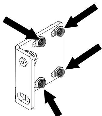
Fig. 22: Régler la serrure de la porte
