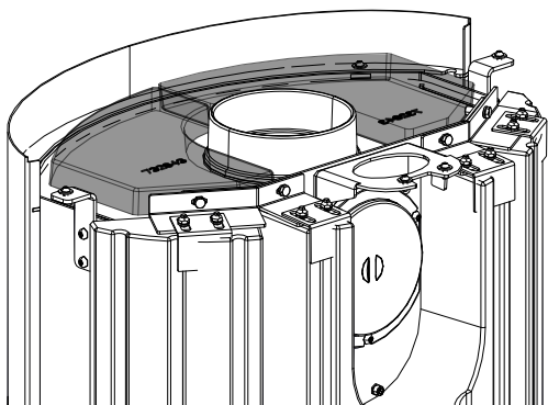
Fig. 6: Fixer les pierres HMS en haut.
