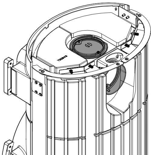
Fig. 12: Recouvrement et tubulure échangés
