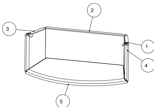
Fig. 17: Installer le compartiment cuisson en Keramott
