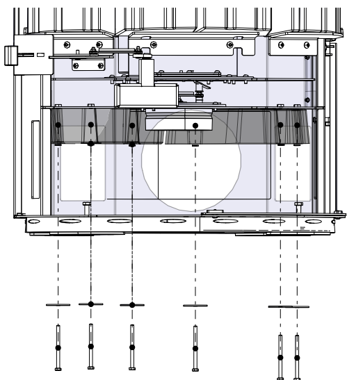
Fig. 7: Monter les pierres HMS en bas
