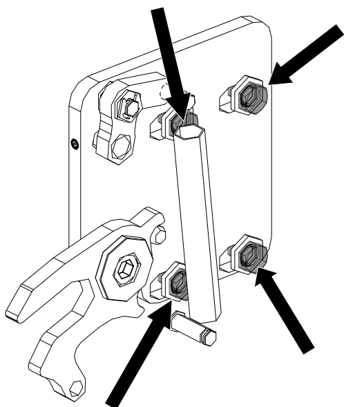
Fig. 20: Régler la serrure de la porte
