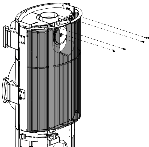
Fig. 5: Installer l'HMS
