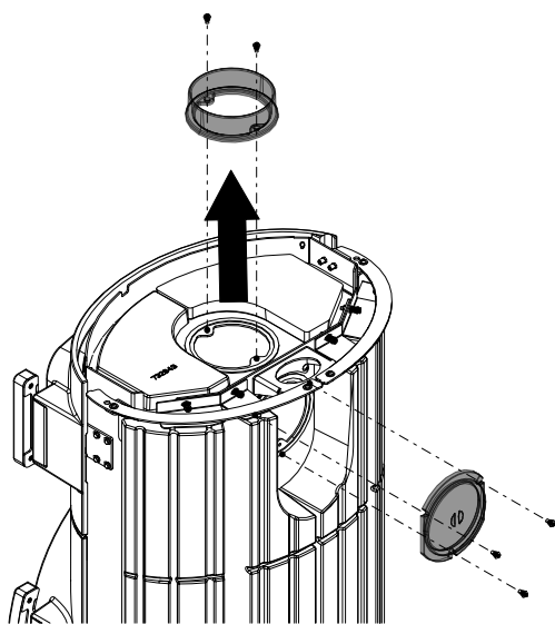
Fig. 10: Démontez le recouvrement et la tubulure de fumées
