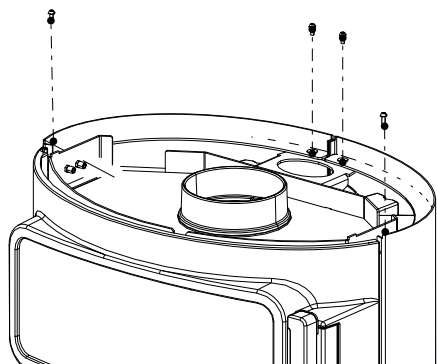
Fig. 38: Dévisser les vis
