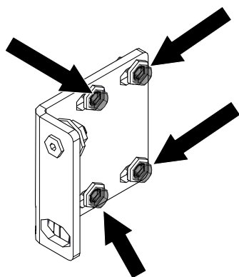
Fig. 22: Regolazione della serratura dello sportello
