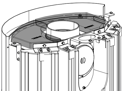
Fig. 6: Attaccare le pietre HMS in alto.
