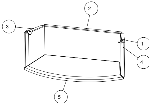
Fig. 17: Montaggio dello scomparto di cottura in Keramott
