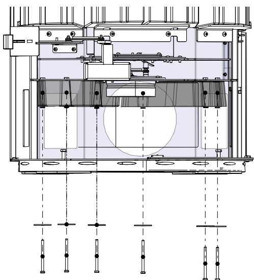
Fig. 7: Montare le pietre HMS in basso
