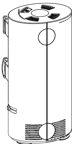
Fig. 8: Collocazione del rivestimento laterale e del coperchio
