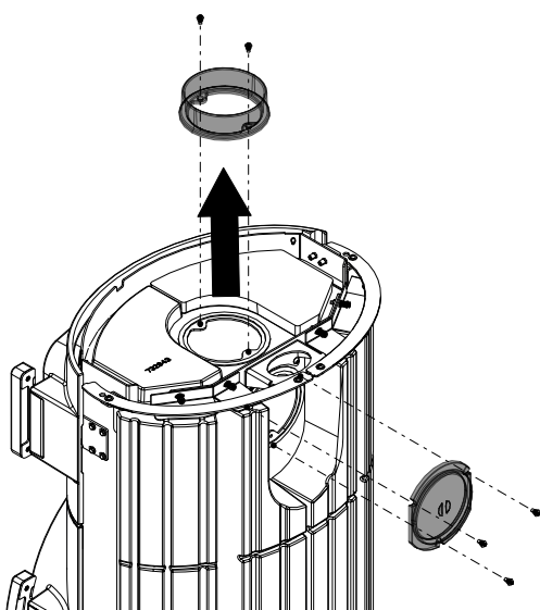
Fig. 10: Smontaggio del coperchio e della presa della canna fumaria
