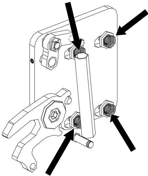
Fig. 20: Regolazione della serratura dello sportello
