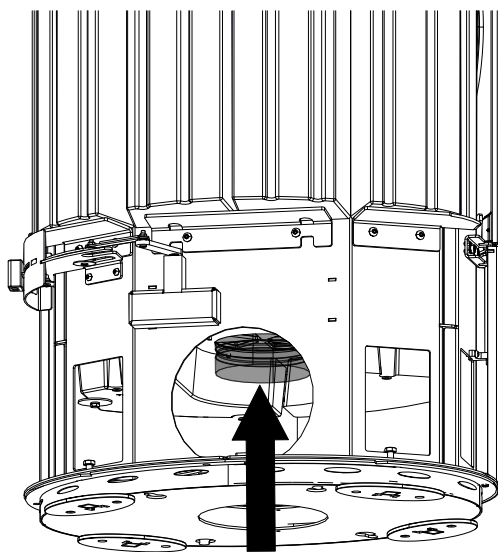
Fig. 15: Fissaggio del tubo Aluflex
