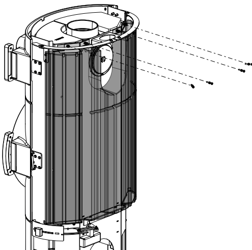
Fig. 8: Montaggio dell'HMS
