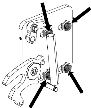
Fig. 22: Regolazione della serratura dello sportello
