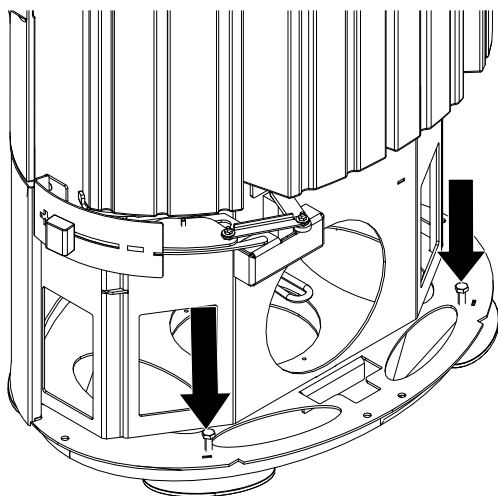
Fig. 19: Allineamento della stufa
