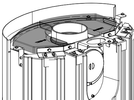
Fig. 41: Rimozione delle pietre HMS
