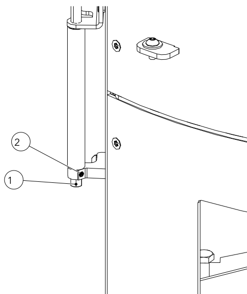
Fig. 28: Regolazione della forza di chiusura dello sportello
