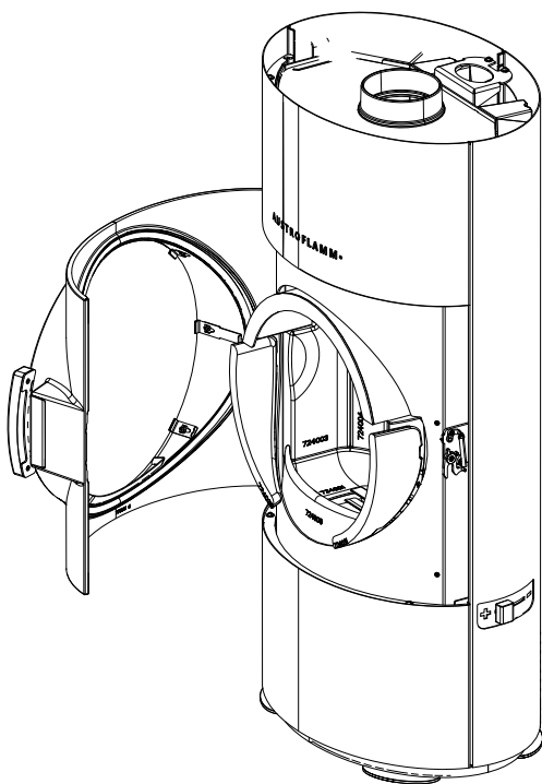
Fig. 26: Apertura dello sportello
