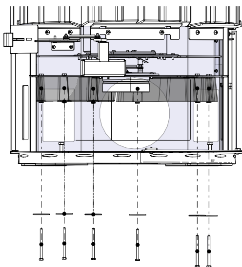
Fig. 43: Montare le pietre HMS in basso
