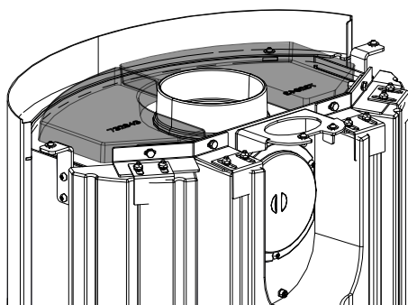
Fig. 9: Attaccare le pietre HMS in alto.
