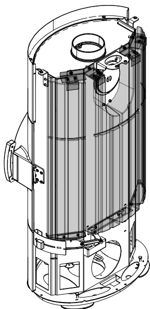
Fig. 7: Montaggio dell'HMS
