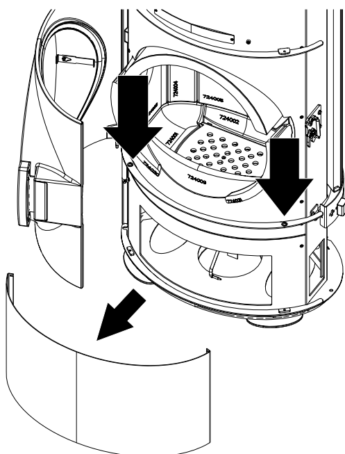
Fig. 22: Smontaggio del rivestimento anteriore inferiore
