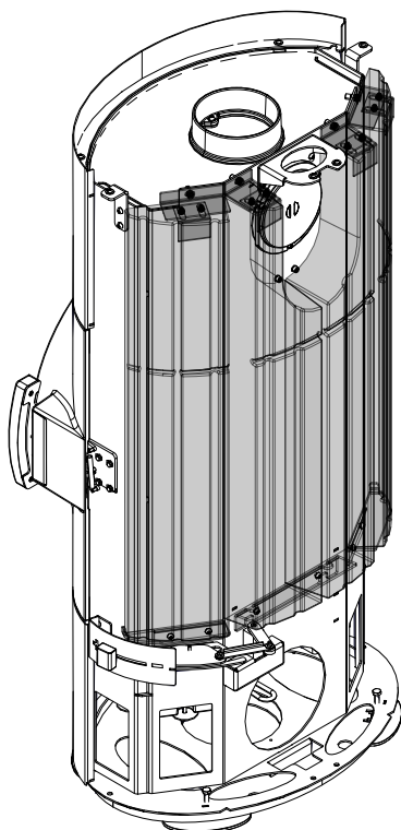
Fig. 42: Svitamento delle viti e smontaggio dell'HMS
