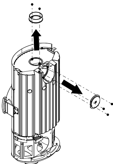
Fig. 12: Smontaggio del coperchio e della presa della canna fumaria
