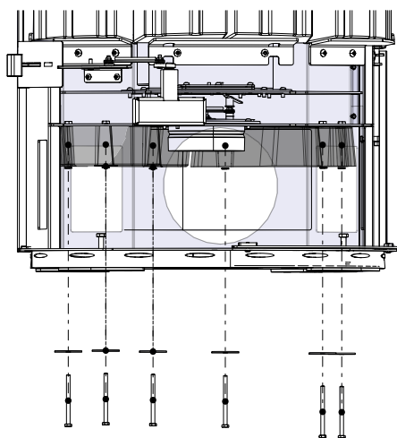
Fig. 8: Montaggio delle pietre HMS dal basso
