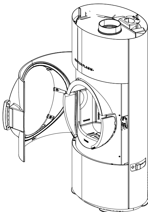
Fig. 24: Apertura dello sportello
