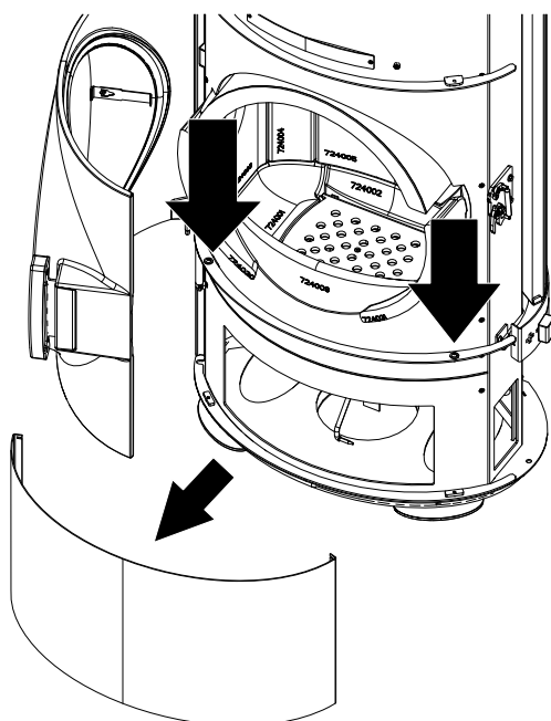
Fig. 27: Smontaggio del rivestimento anteriore inferiore
