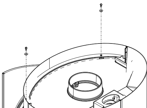
Fig. 20: Smontaggio del rivestimento anteriore superiore
