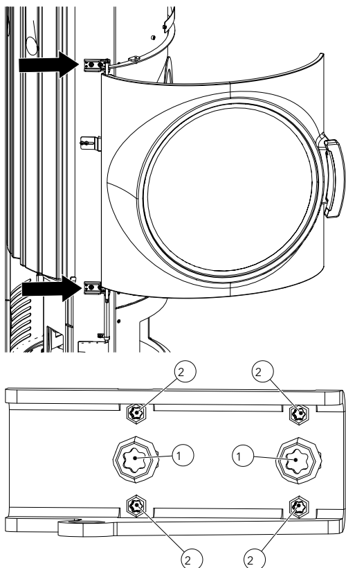
Fig. 23: Viti di registro dello sportello
