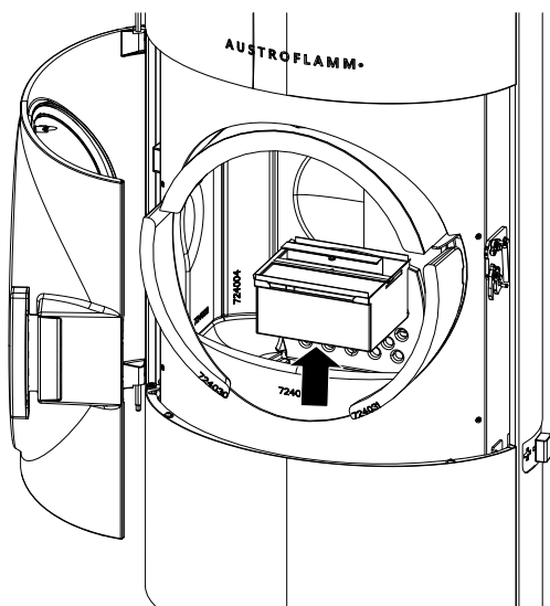
Fig. 31: Rimozione e svuotamento del box cenere
