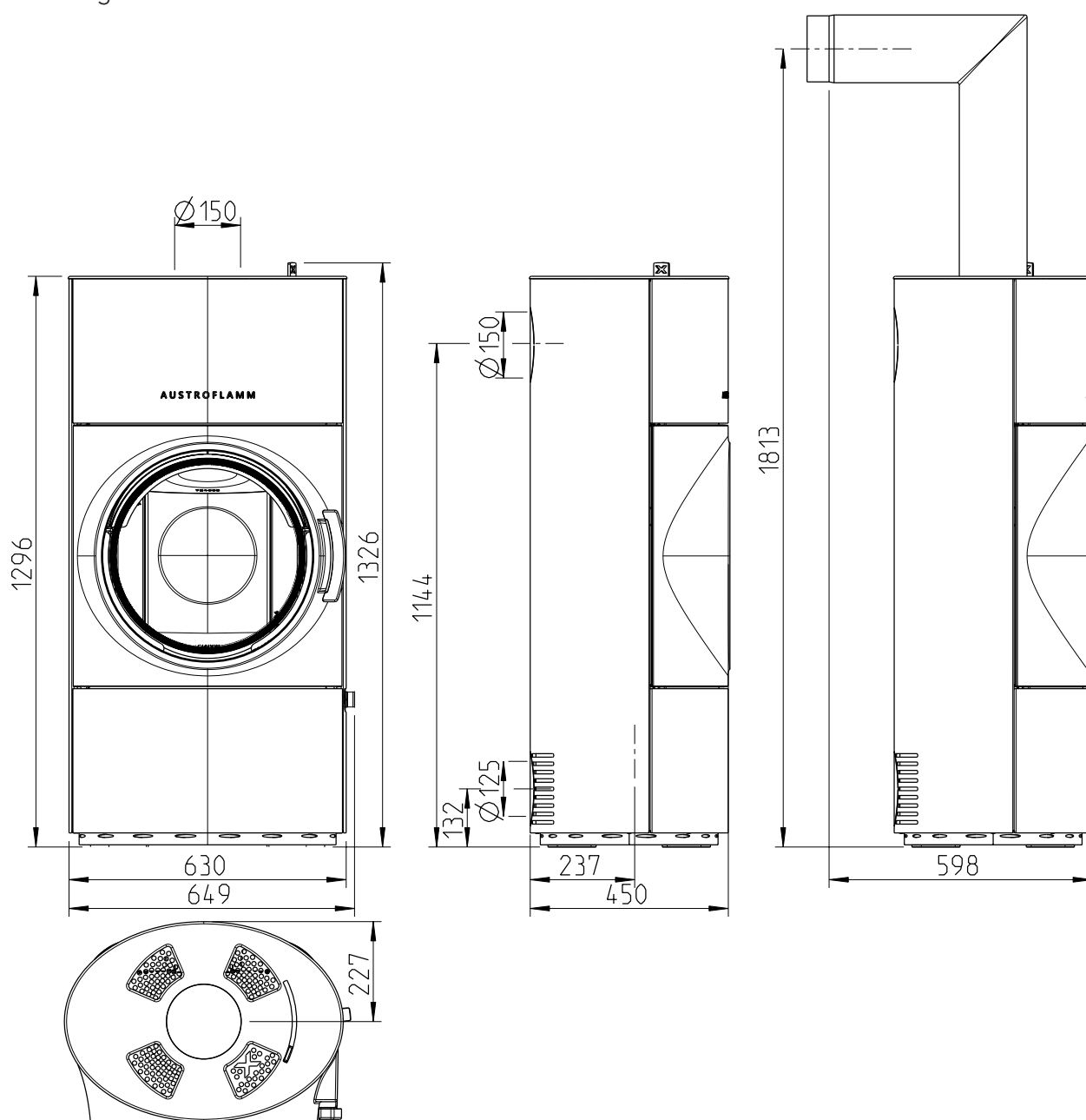
Fig. 1: Dimensioni dell'apparecchio di base
