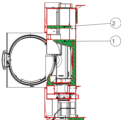
Fig. 38: Rimozione del Keramott e del deflettore
