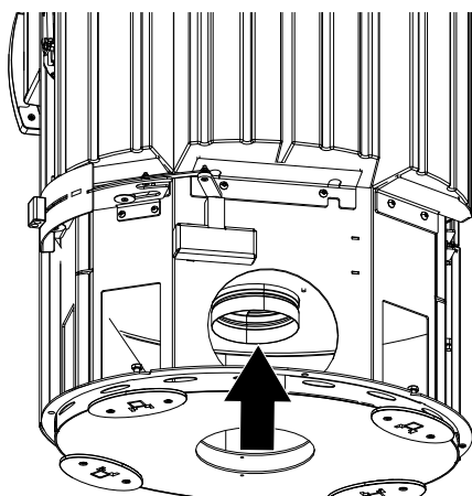
Fig. 14: Fissaggio del tubo Aluflex
