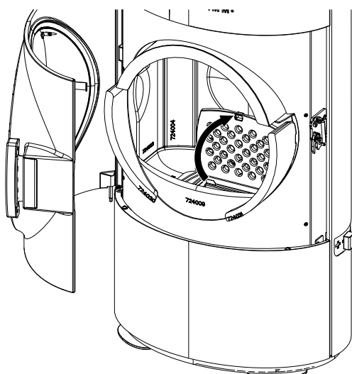
Fig. 28: Sollevamento della griglia
