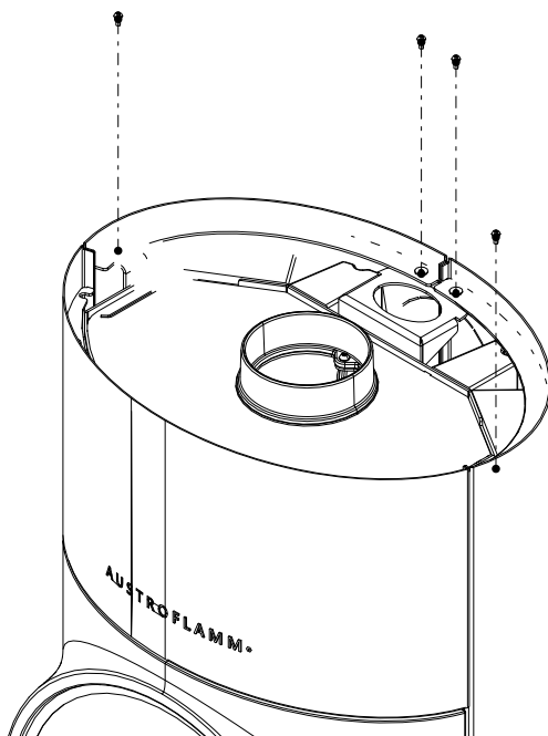
Fig. 36: Svitamento delle viti
