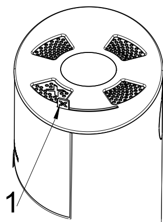
Fig. 32: Regolatore della convezione dell'aria
