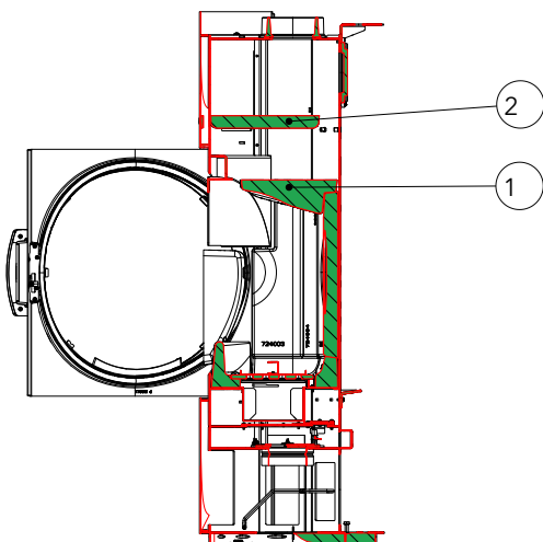
Abb. 39: Keramik und Umlenkplatte herausnehmen
