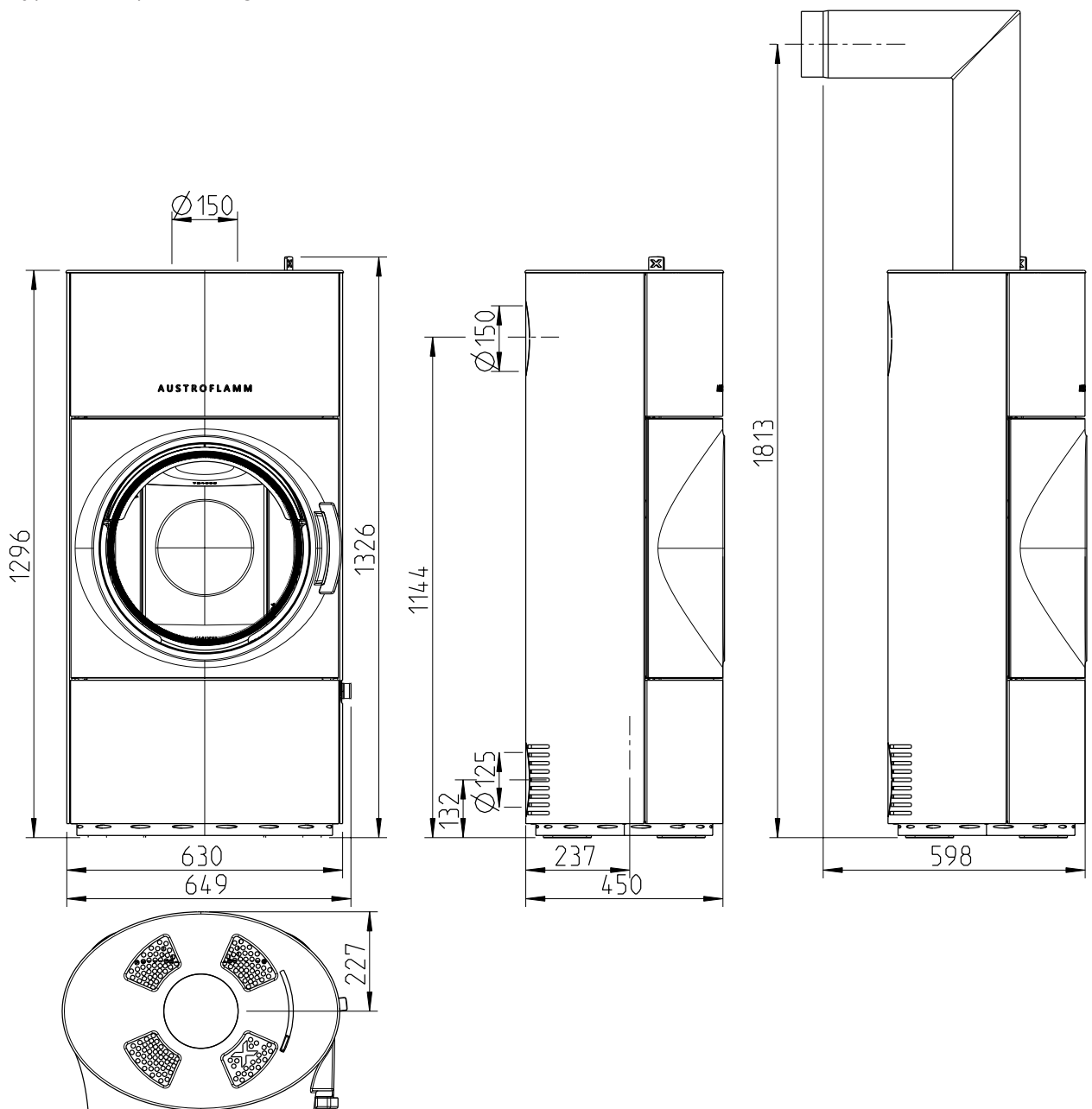
Abb. 2: Abmessungen Grundgerät
