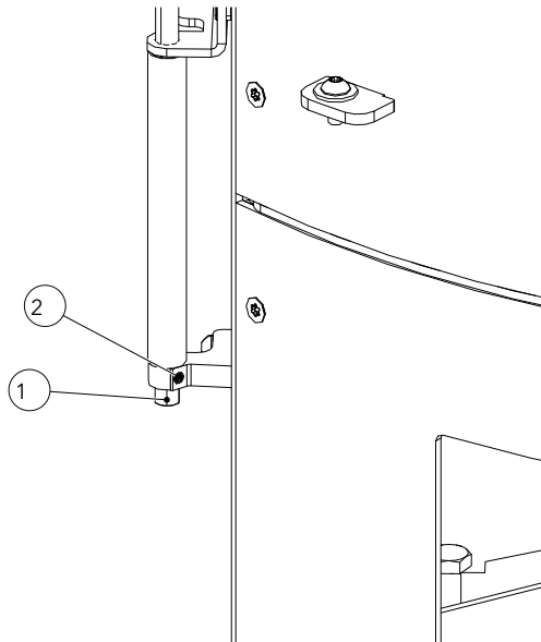
Abb. 25: Türschließkraft einstellen
