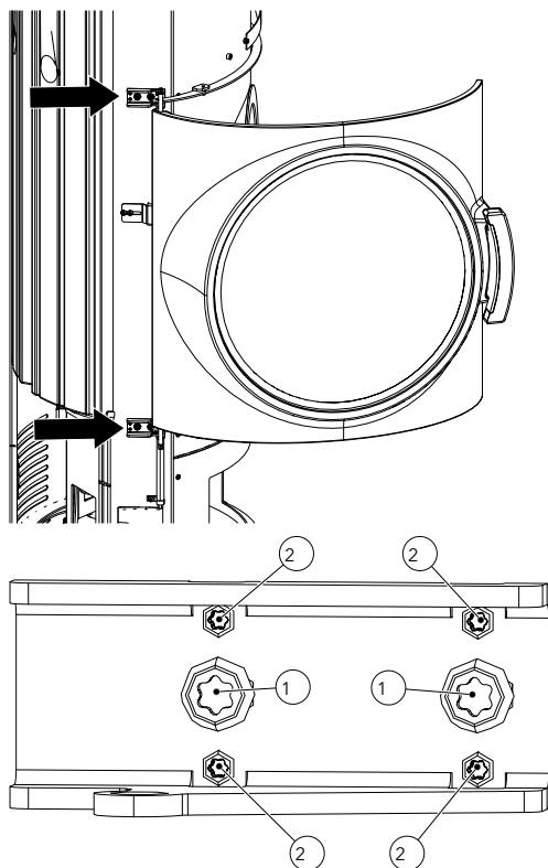
Abb. 20: Türeinsteilschrauben
