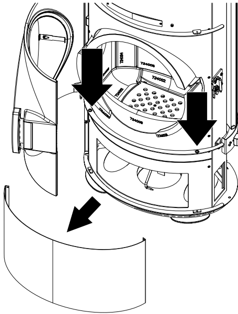
Abb. 24: unten vordere Verkleidung demonstrieren
