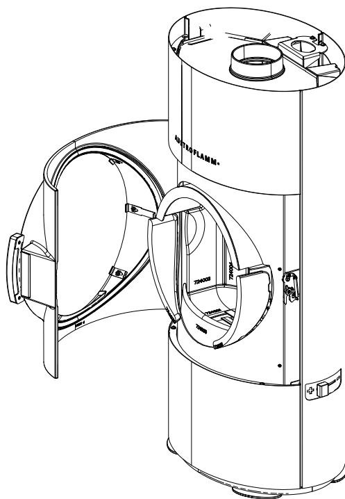
Abb. 21: Tür öffnen
