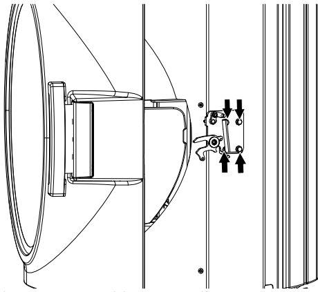
Abb. 22: Türverschluss einstellen
