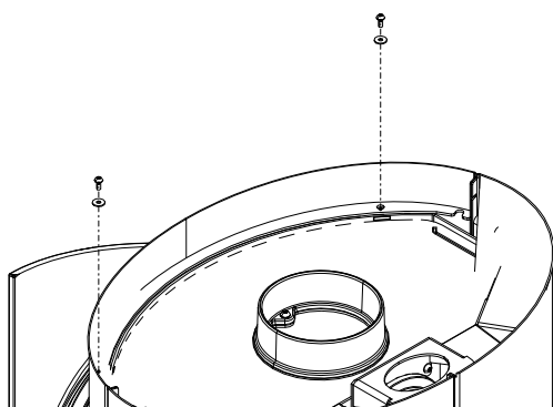
Abb. 17: vordere Verkleidung oben demonstrieren
