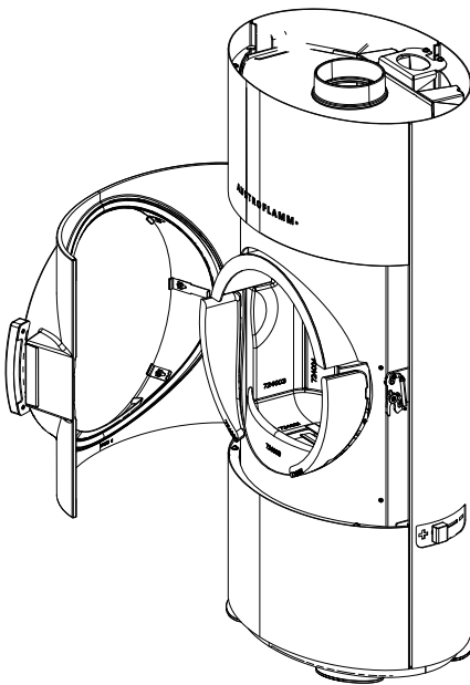
Abb. 23: Tür öffnen
