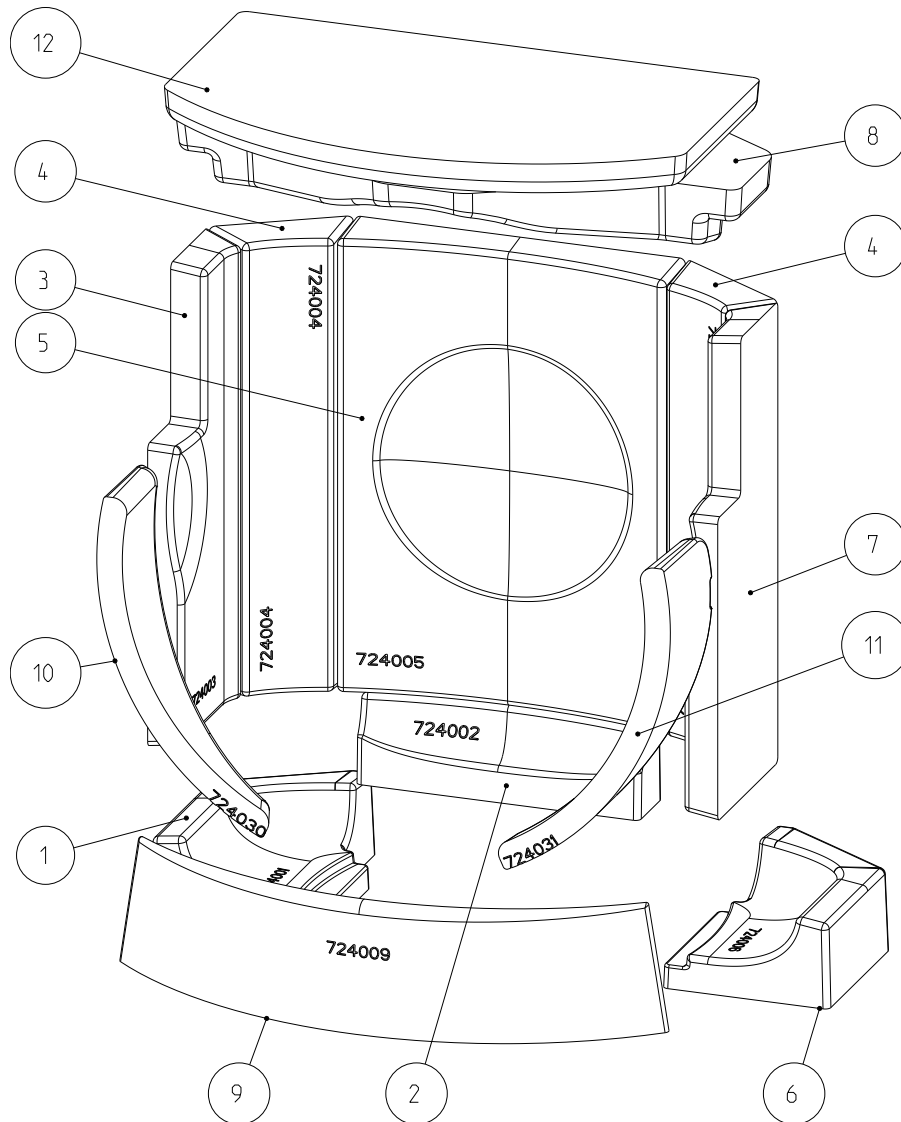
Abb. 35: Keramott
