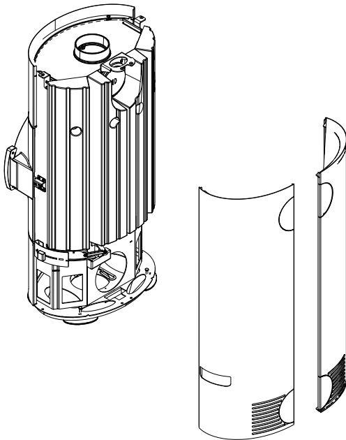
Abb. 38: Seitenverkleidung abnehmen
