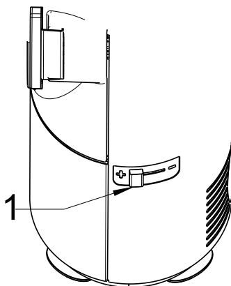
Abb. 26: Primär-Sekundärluftregler
