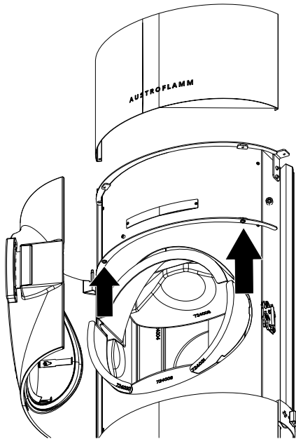
Abb. 18: obere vordere Verkleidung demon- tieren
