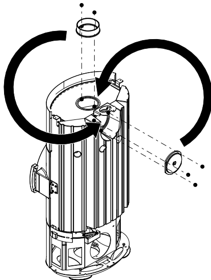
Abb. 11: Abdeckung und Stutzen tauschen
