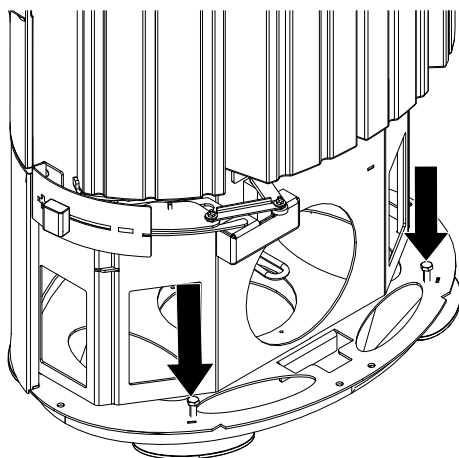
Abb. 16: Kaminofen ausrichten
