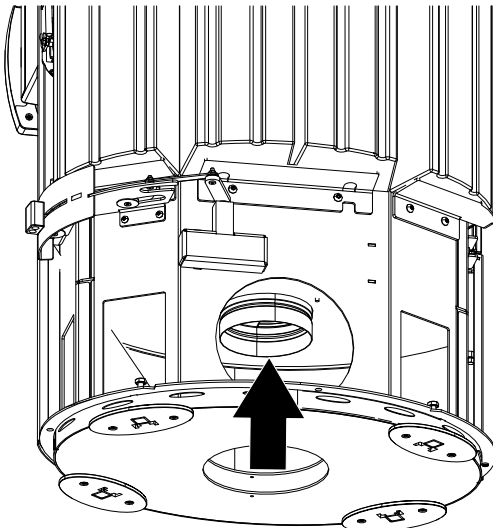
Abb. 15: Aluflexschlauch befestigen
