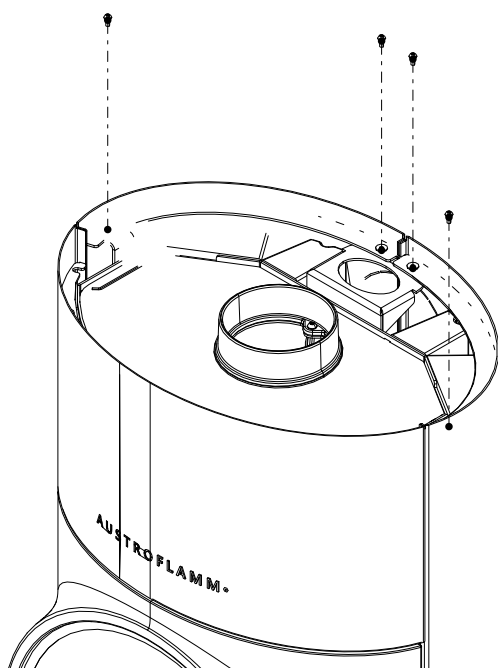
Abb. 37: Schrauben lösen
