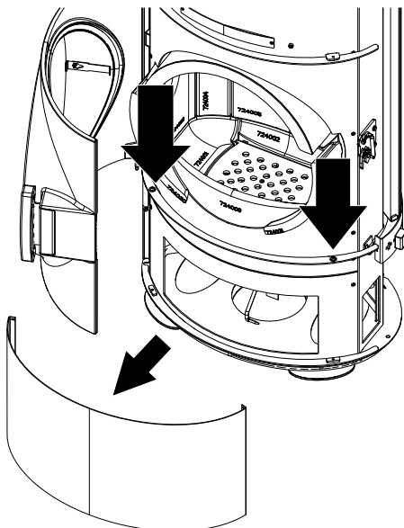
Abb. 19: unten vordere Verkleidung demon- tieren
