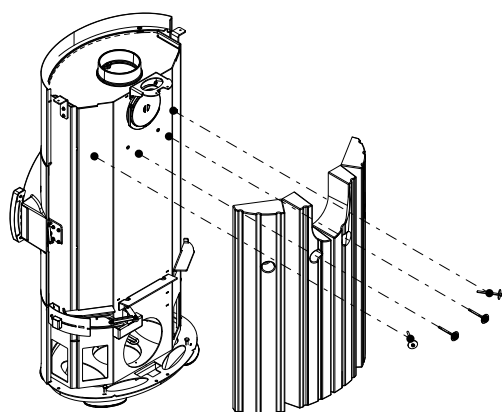
Abb. 40: Schrauben lösen und HSM demontieren
