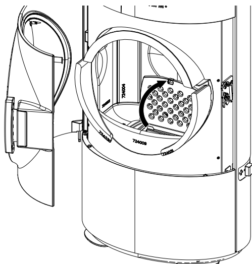
Fig. 29: Relever la grille
