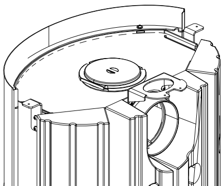
Fig. 11: Recouvrement et tubulure échangés
