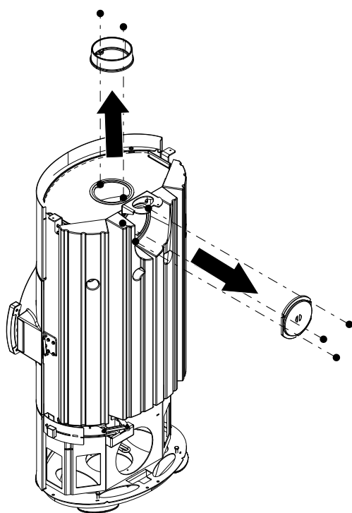
Fig. 9: Démonter le recouvrement et la tubulure de fumées
