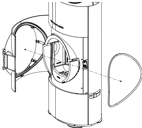
Fig. 28: Remplacer le joint
