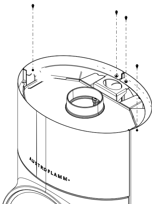
Fig. 40: Dévisser les vis
