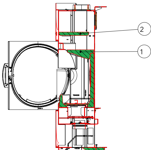
Fig. 42: Enlever la Keramott et la plaque déflectrice
