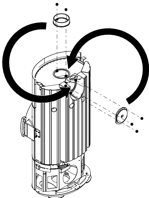
Fig. 10: Échanger le recouvrement et la tubulure
