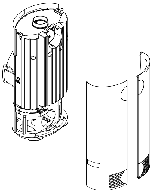
Fig. 41: Enlever l'habillage latéral
