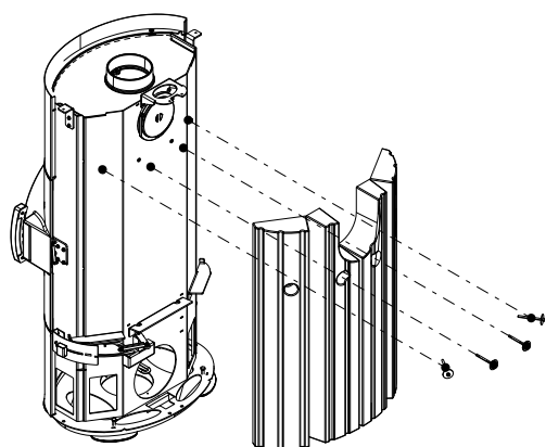
Fig. 43: Dévisser les vis et déposer l'HMS
