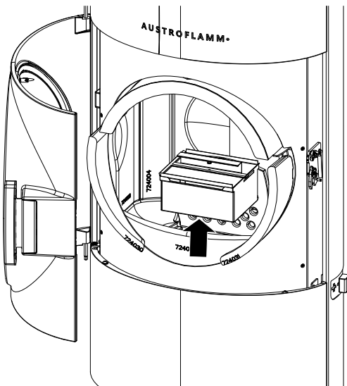
Fig. 32: Enlever et vider le bac à cendres
