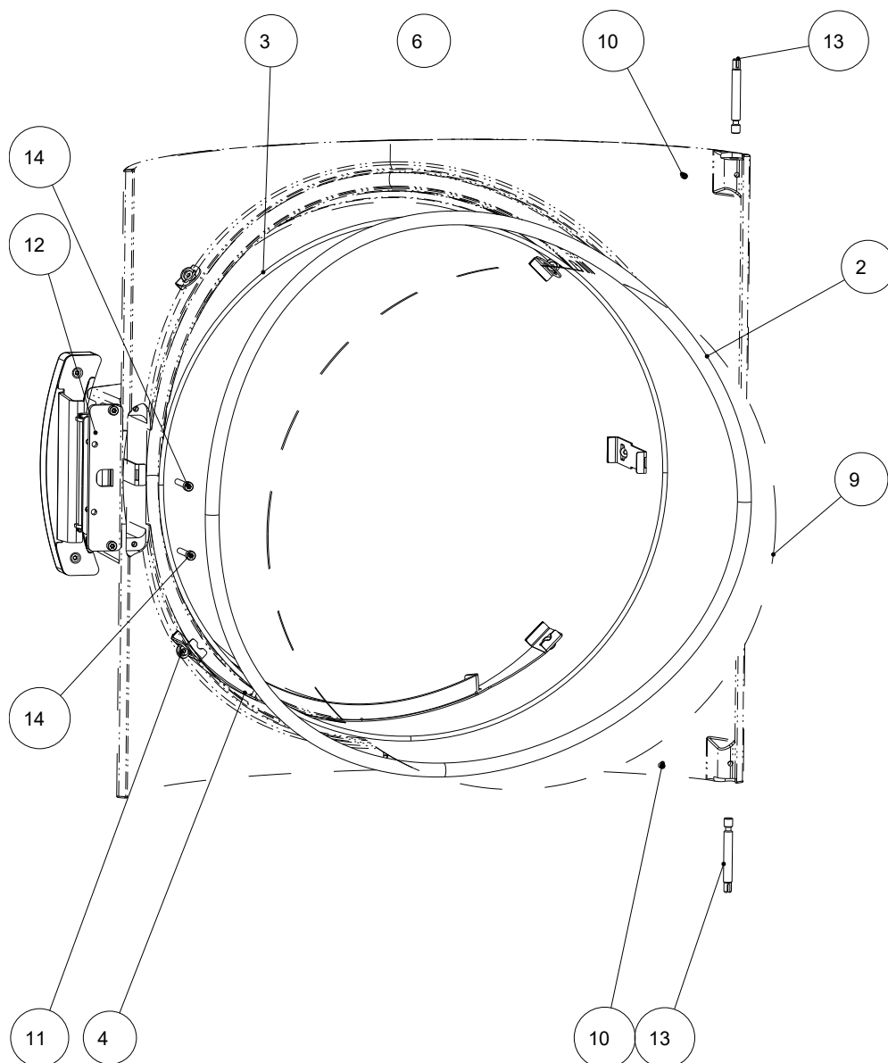
Fig. 38: Porte de la chambre de combustion
