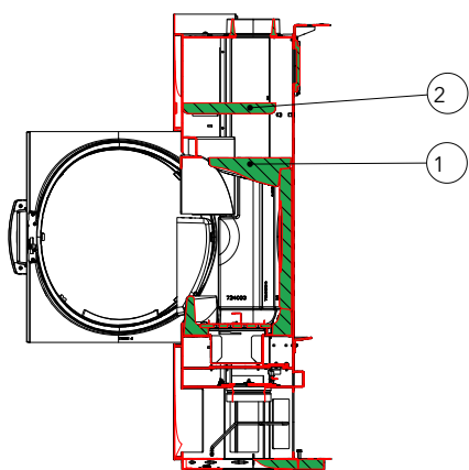
Fig. 42: Rimozione del Keramott e del deflettore
