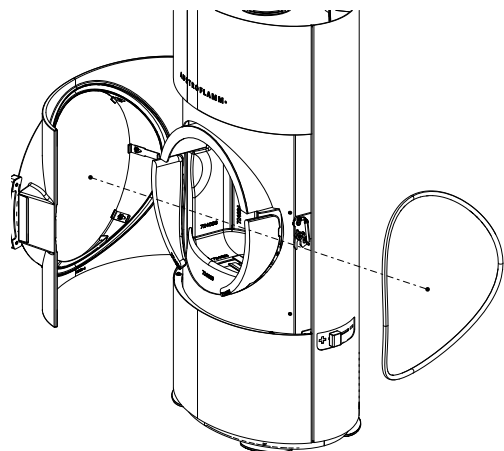
Fig. 28: Sostituzione della guarnizione
