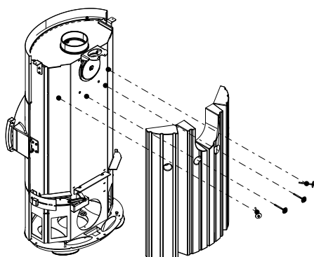
Fig. 43: Svitamento delle viti e smontaggio dell'HMS
