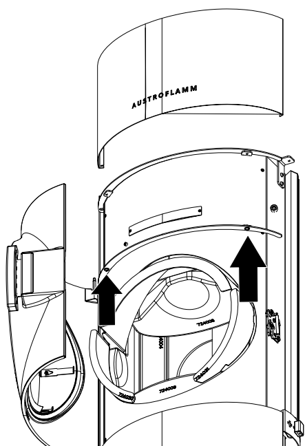
Abb. 17: obere vordere Verkleidung demon- tieren
