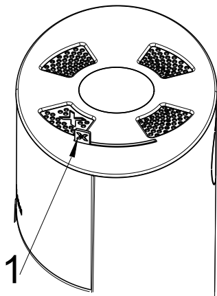
Abb. 33: Konvektionsluftregler
