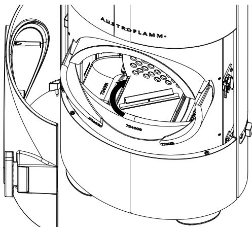
Abb. 30: Deckel auf Aschebox geben
