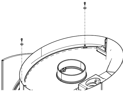
Abb. 16: vordere Verkleidung oben demonstrieren
