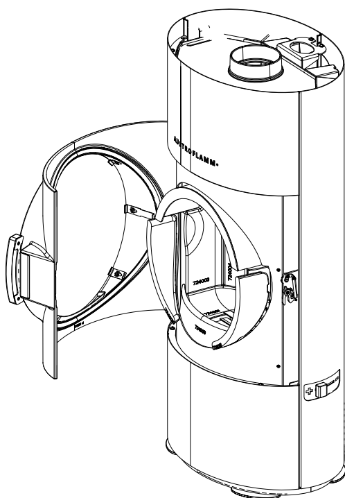
Abb. 22: Tür öffnen
