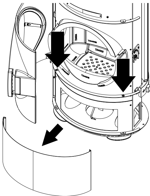
Abb. 18: unten vordere Verkleidung demon- tieren
