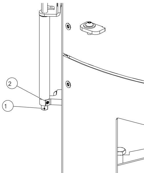
Abb. 24: Türschließkraft einstellen
