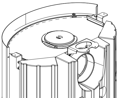
Abb. 11: Abdeckung und Stutzen vertauscht
