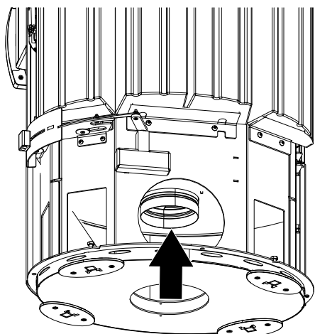
Abb. 14: Aluflexschlauch befestigen
