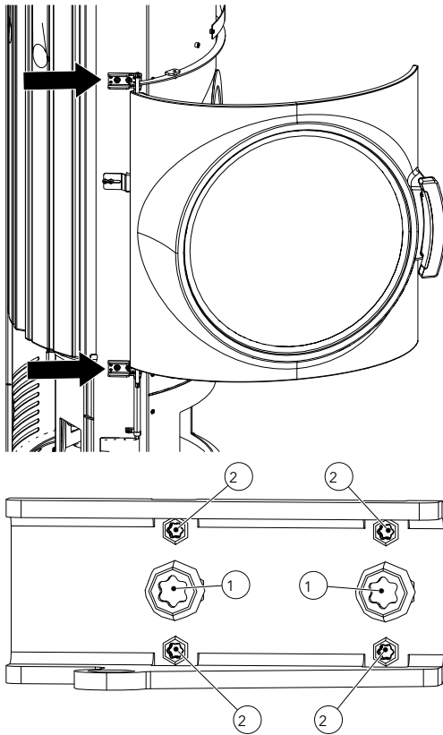
Abb. 19: Türeinstellschrauben
