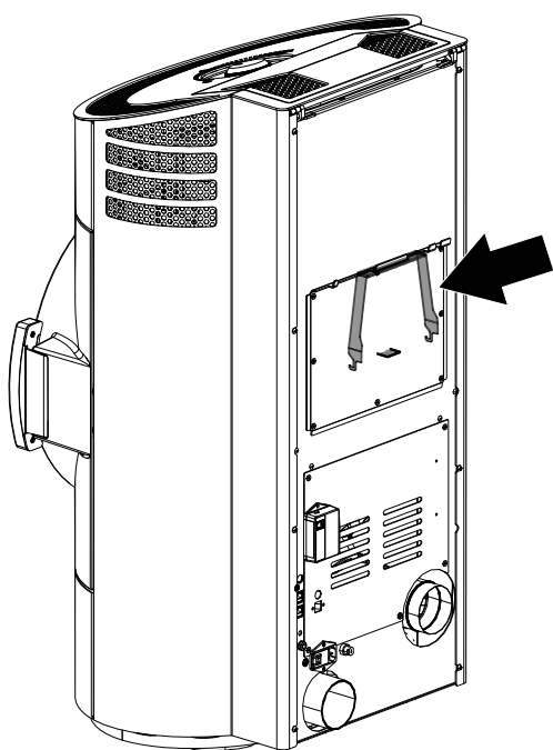
Fig. 23: Outil de levage
