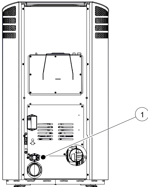
Fig. 34: Limiteur de température de sécurité
