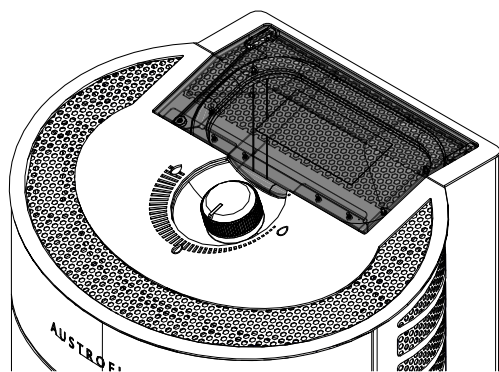
Fig. 29: Refermer le couvercle du réservoir
