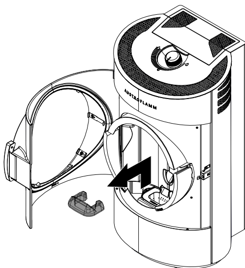
Fig. 24: Enlever la dalle avant
