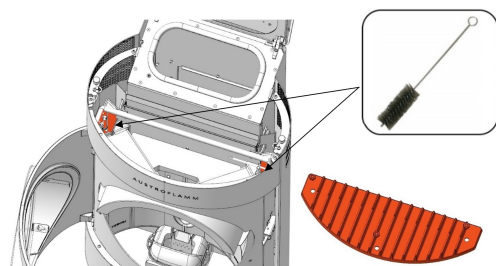
Fig. 34: Spazzolatura delle canne fumarie
