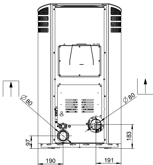
Fig. 10: Collegamento posteriore
