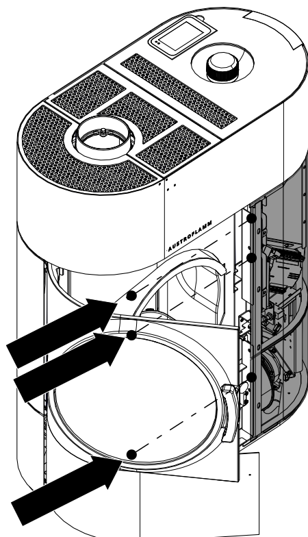
Fig. 19: Dévisser les vis
