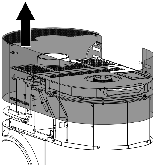
Fig. 95: Enlever l'habillage supérieur
