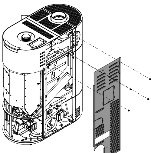
Fig. 22: Enlever le panneau arrière
