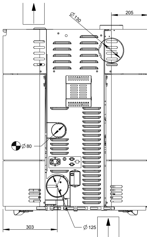
Fig. 33: Raccordement de l'alimentation en air de combustion
