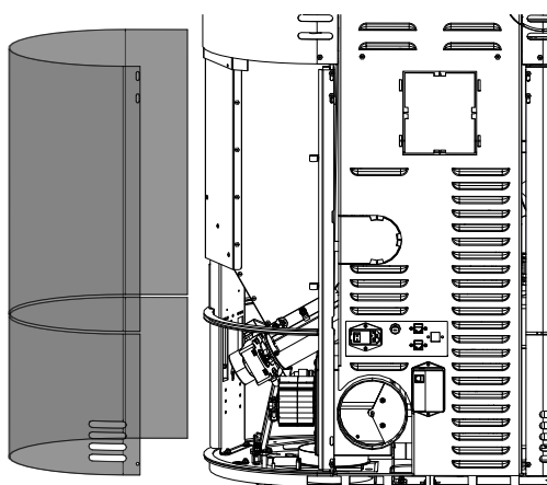
Fig. 21: Enlever l'habillage latéral
