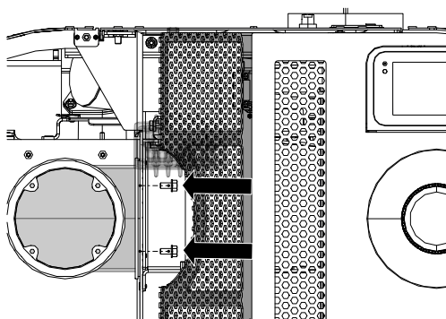
Fig. 15: Déposer le conduit coudé
