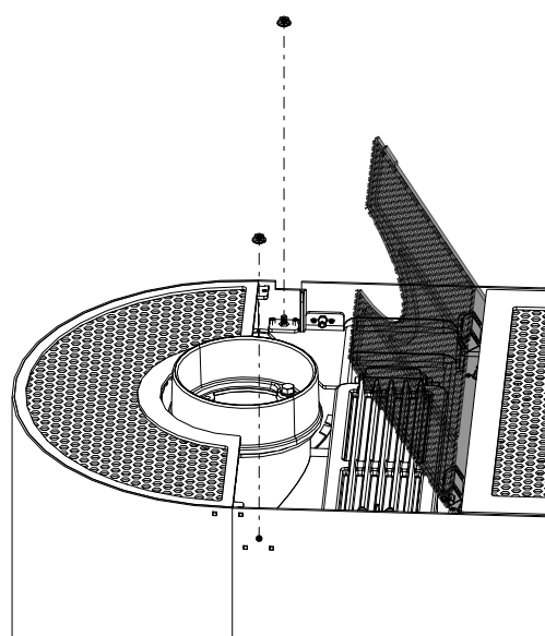
Fig. 93: Dévisser les écrous
