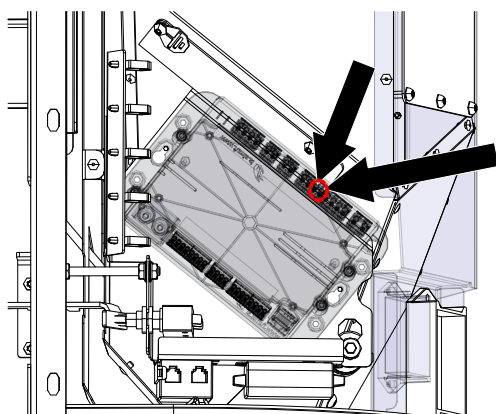
Fig. 27: Brancher le kit canalisation
