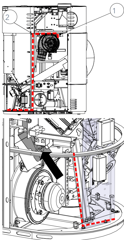
Fig. 25: Poser le câble et fixer le condensateur
