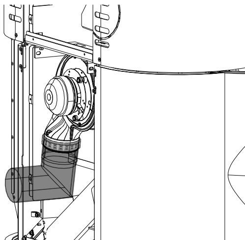
Fig. 29: Mettre le tube sur le kit
