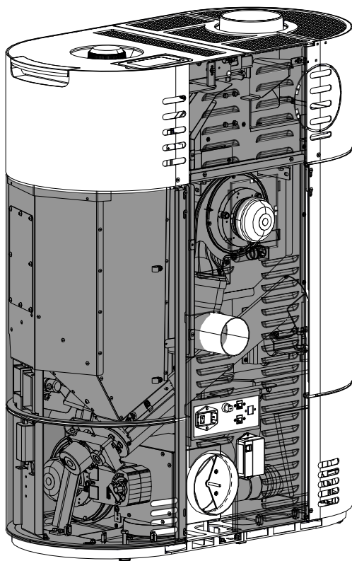
Fig. 31: Remettre tout en place
