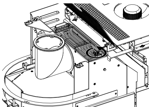
Fig. 14: Ouvrir la trappe de visite
