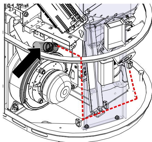
Fig. 25: Poser le câble et fixer le condensateur
