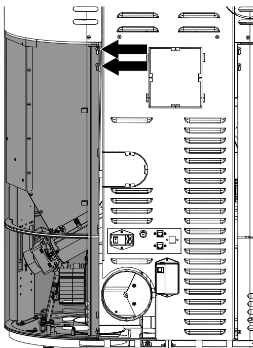
Fig. 20: Dévisser les vis
