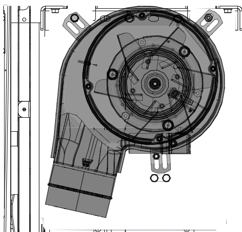
Fig. 23: Installer le kit canalisation
