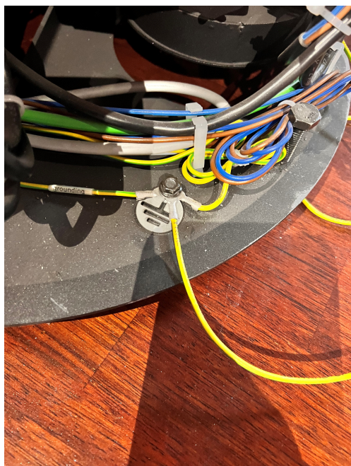
Fig. 28: Raccorder à la mise à la terre centrale
