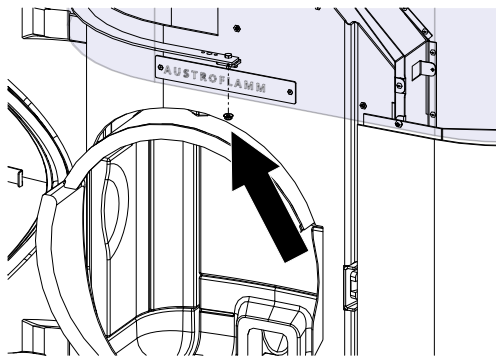
Fig. 94: Ouvrir la porte et dévisser l'écrou.
