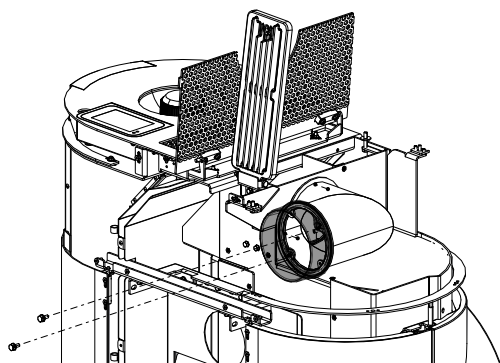
Fig. 17: Installer la tubulure de fumées
