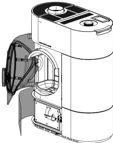
Fig. 18: Ouvrir les portes
