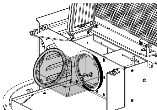
Fig. 16: Tourner le conduit coudé
