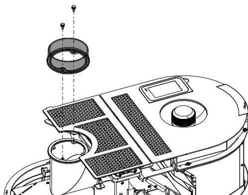
Fig. 13: Enlever la tubulure de fumées
