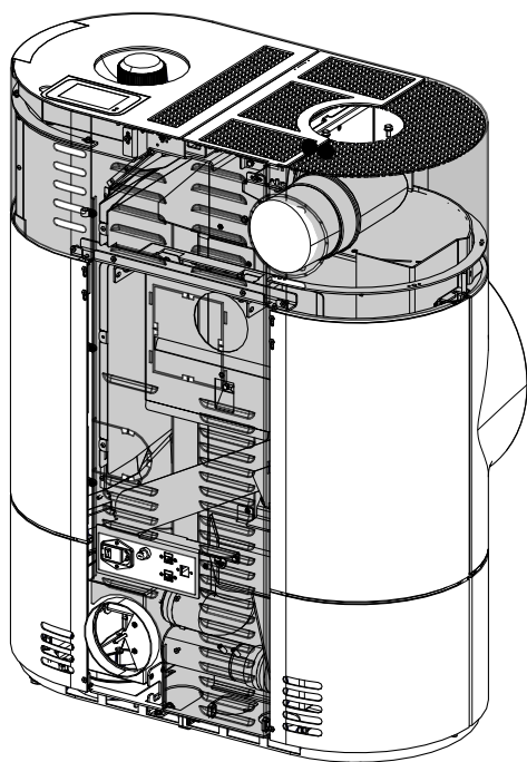
Fig. 17: Installer la tubulure de fumées
