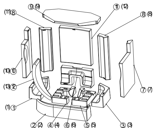
Fig. 9: Installer la Keramott
