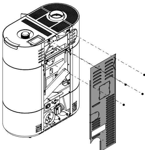
Fig. 10: Enlever le panneau arrière
