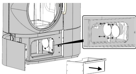
Fig. 85: Rimozione del vassoio della cenere e della copertura
