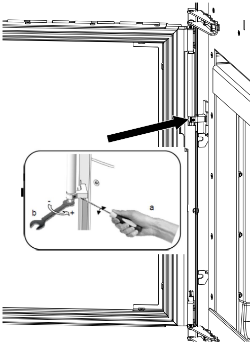
Fig. 73: Regolazione della molla di pressione
