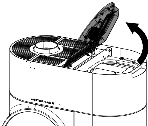
Fig. 90: Apertura del coperchio del serbatoio
