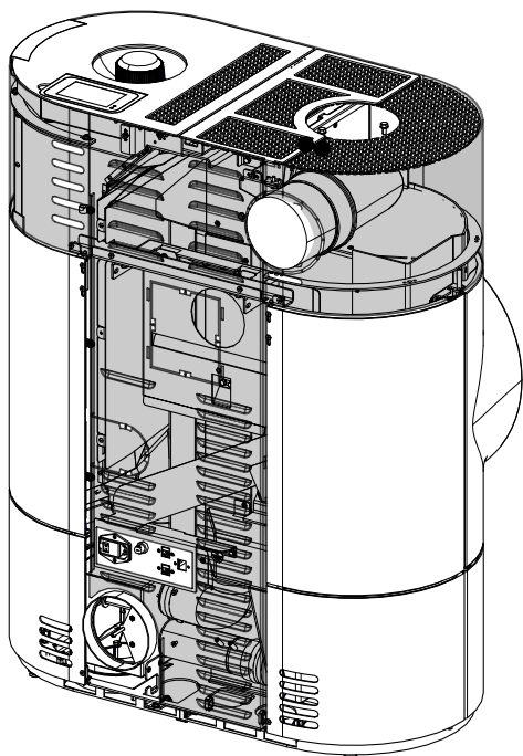
Fig. 16: Montaggio della presa della canna fumaria
