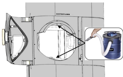
Fig. 84: Apertura dello sportello della camera di combustione e relativa pulizia
