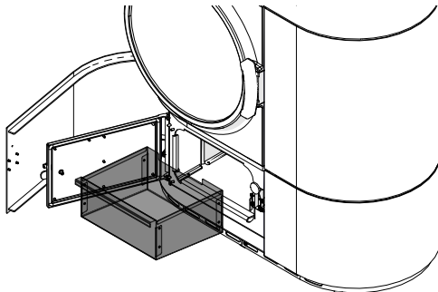
Fig. 79: Rimozione del cassetto della cenere
