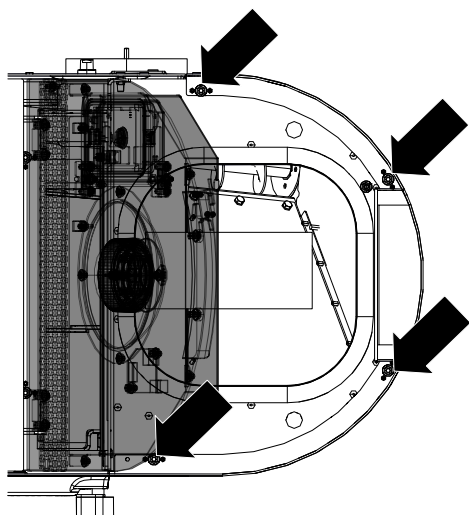
Fig. 91: Svitamento delle viti
