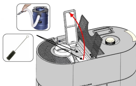
Fig. 83: Apertura del coperchio per la pulizia e relativa pulizia
