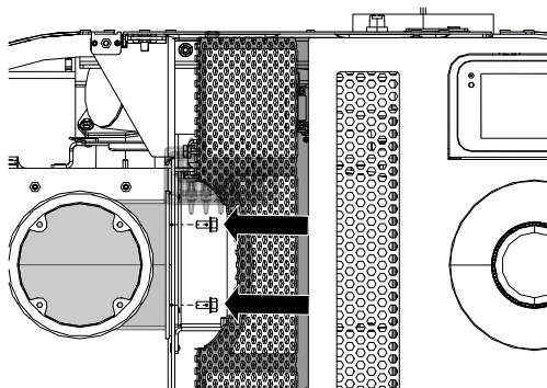
Fig. 14: Smontaggio del gomito del tubo dei fumi
