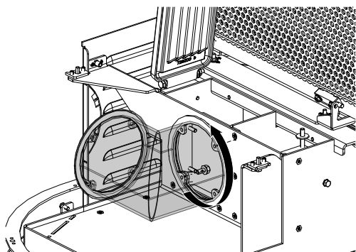
Fig. 15: Rotazione del gomito del tubo dei fumi
