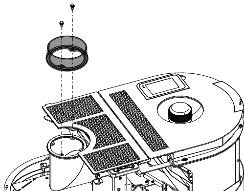
Fig. 12: Rimozione della presa della canna fumaria
