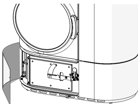
Fig. 77: Aprire lo sportello in basso
