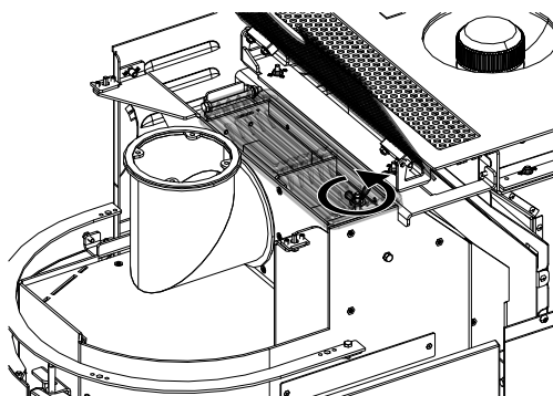
Fig. 13: Apertura del coperchio per la pulizia
