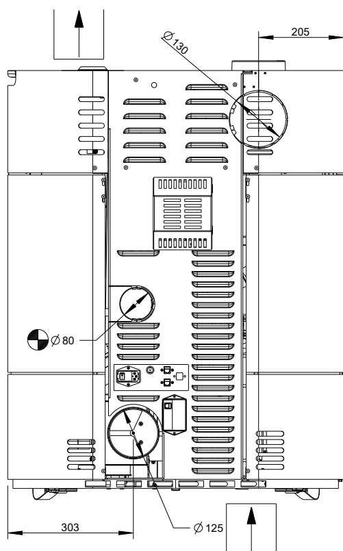
Fig. 32: Collegamento dell'alimentazione esterna di aria comburente
