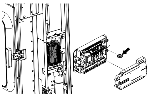
Fig. 76: Sostituzione della batteria tampone
