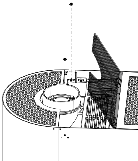
Fig. 92: Svitamento dei dadi
