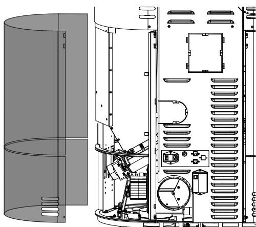
Fig. 20: Rimozione del rivestimento laterale
