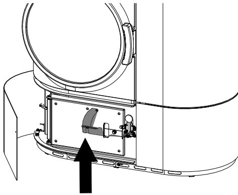
Fig. 78: Apertura dello sportello del cassetto della cenere
