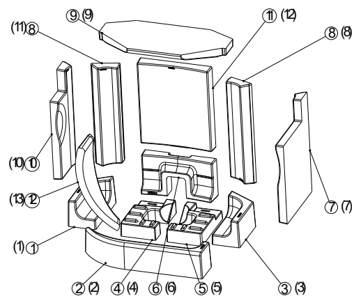
Fig. 8: Montaggio del Keramott
