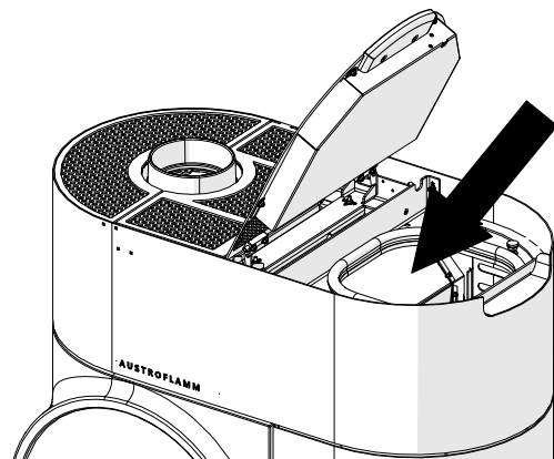
Fig. 40: Riempire i pellet
