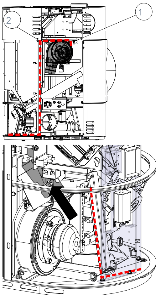
Fig. 24: Posa del cavo e fissaggio del condensatore
