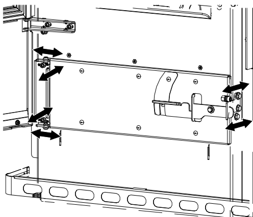
Fig. 75: Regolazione dello sportello del vassoio per la cenere
