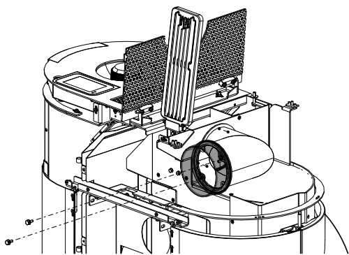
Fig. 16: Montaggio della presa della canna fumaria
