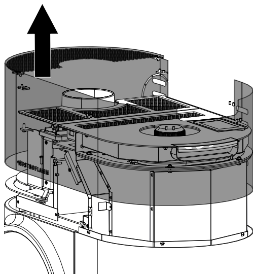
Fig. 94: Rimozione del rivestimento superiore
