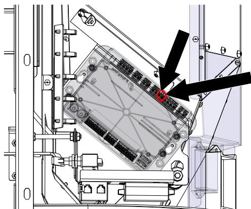
Fig. 26: Collegamento del modulo del diffusore dell'aria
