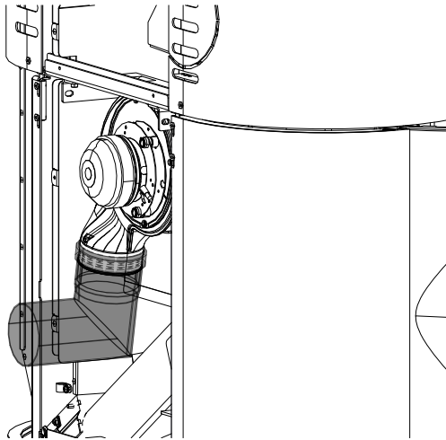
Fig. 28: Collegamento del tubo
