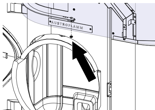
Fig. 93: Apertura dello sportello e svitamento dei dadi
