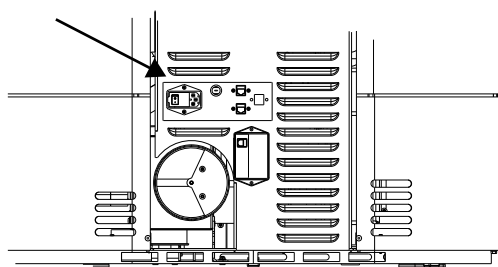
Fig. 33: Collegamento elettrico
