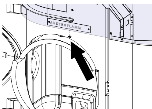
Fig. 93: Apertura dello sportello e svitamento dei dadi
