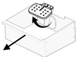
Fig. 82: Griglia a battente
