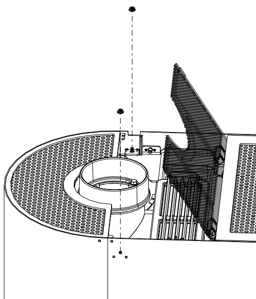
Fig. 92: Svitamento dei dadi
