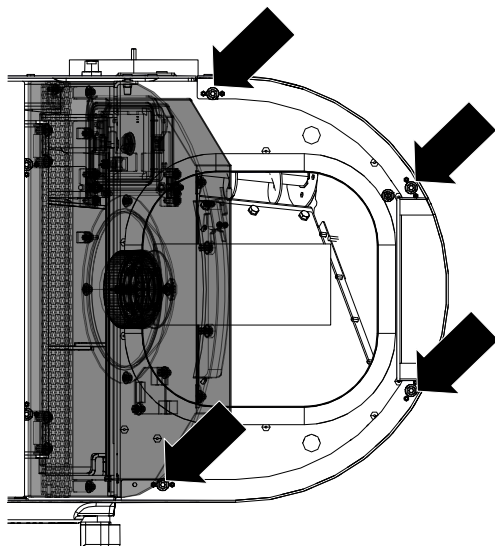
Fig. 91: Svitamento delle viti
