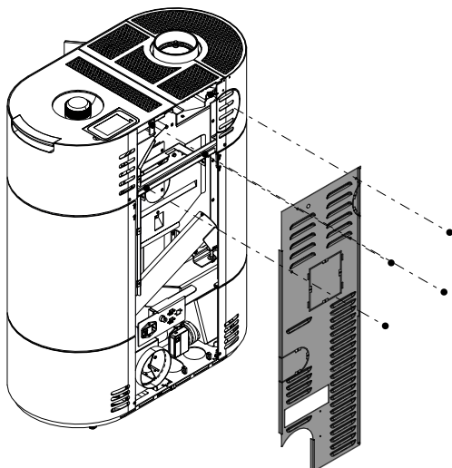
Fig. 9: Rimozione della parete posteriore
