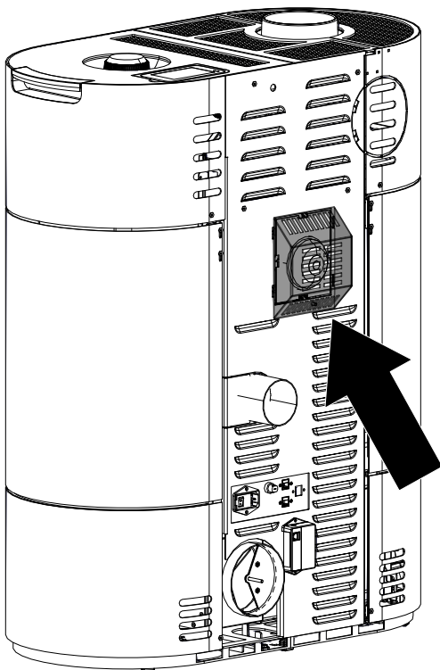
Abb. 33: Abdeckung auf Rückwand anbringen
