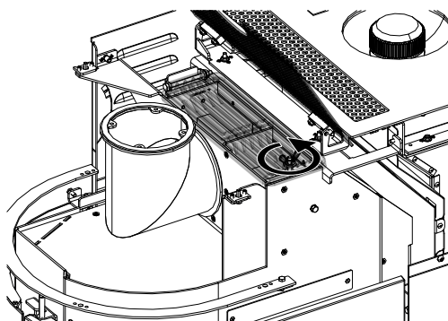
Abb. 15: Putzdeckel öffne
