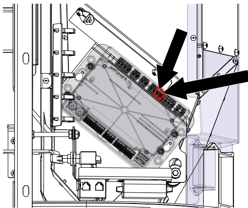
Abb. 28: Luftverteilermodul anstecken
