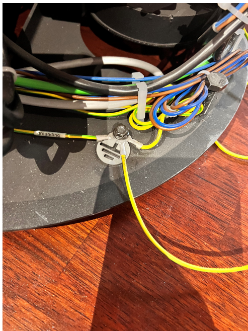
Abb. 29: Zentralerdung anschließen
