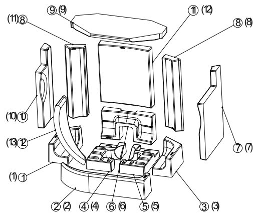
Abb. 10: Keramott montieren
