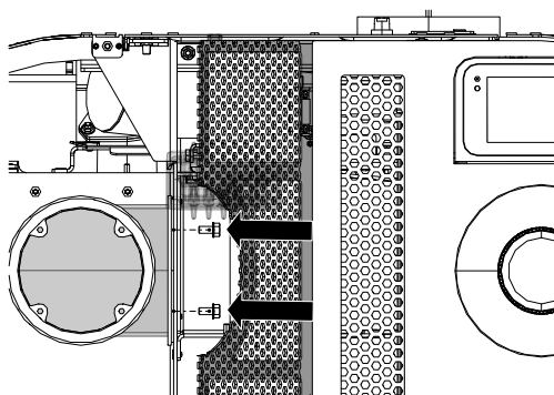
Abb. 16: RR-Bogen demontieren
