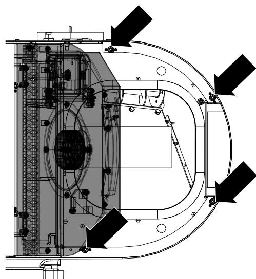
Abb. 93: Schrauben lösen
