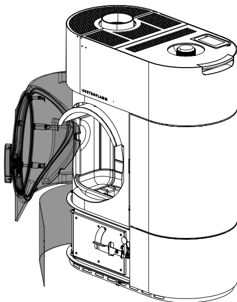
Abb. 19: Türen öffnen
