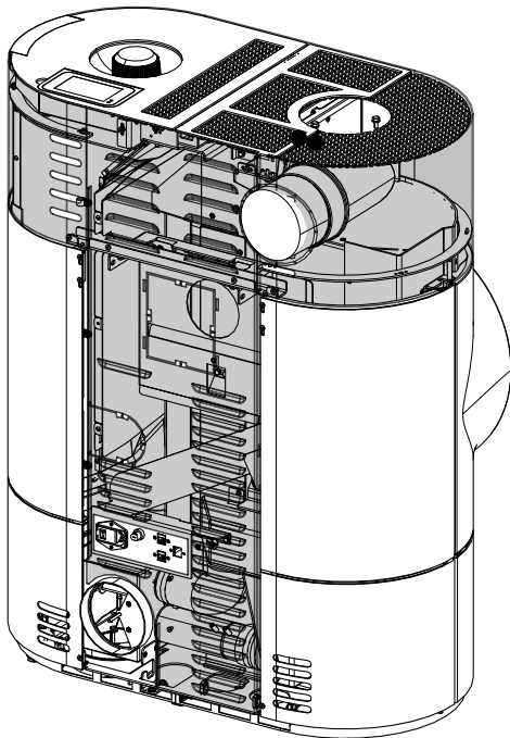
Abb. 18: Rauchrohrstutzen montieren
