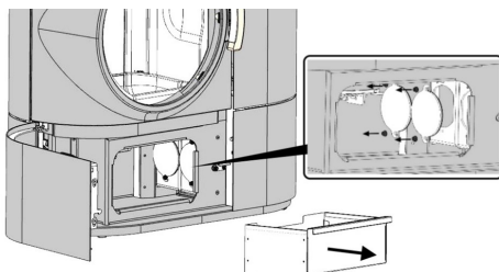
Abb. 87: Aschelade und Abdeckungen entfernen
