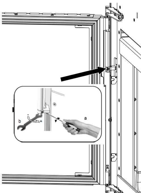
Abb. 75: Spannfeder einstellen
