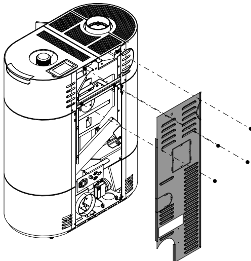
Abb. 11: Rückwand abnehmen
