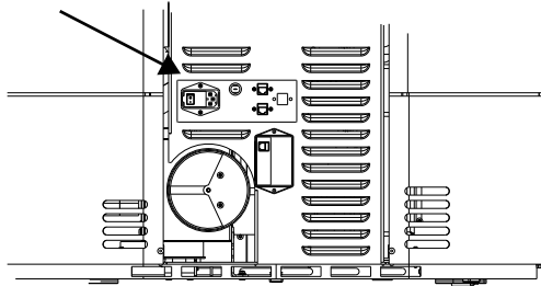
Abb. 91: Elektrischer Anschluss
