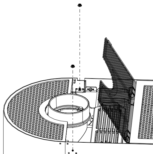
Abb. 93: Schrauben lösen
