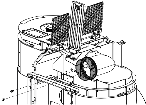
Abb. 18: Rauchrohrstutzen montieren
