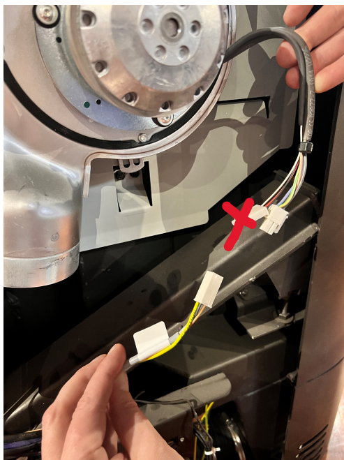
Abb. 25: Kabel verbinden
