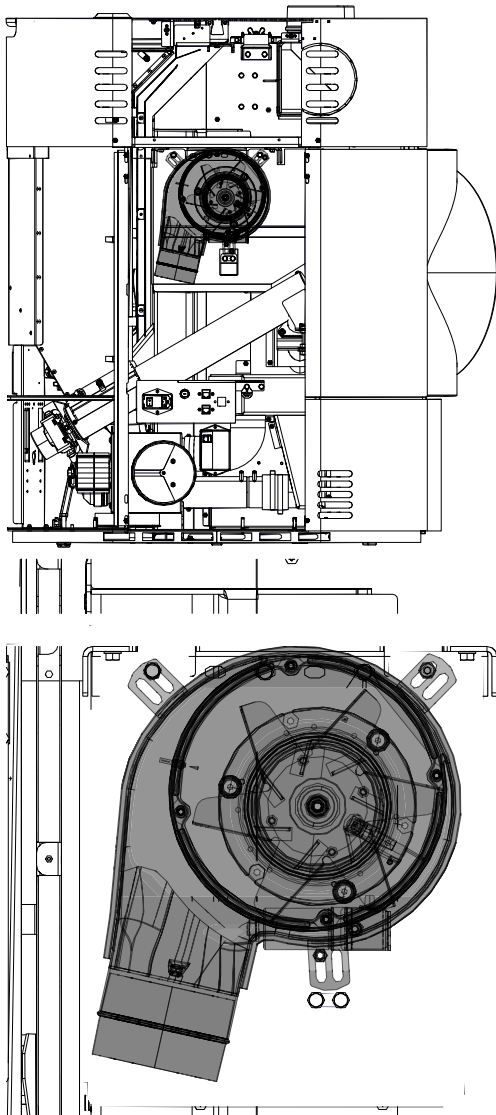
Abb. 24: Luftmodul anbringen
