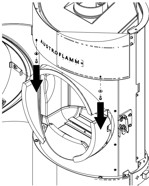
Fig. 40: Svitamento delle viti
