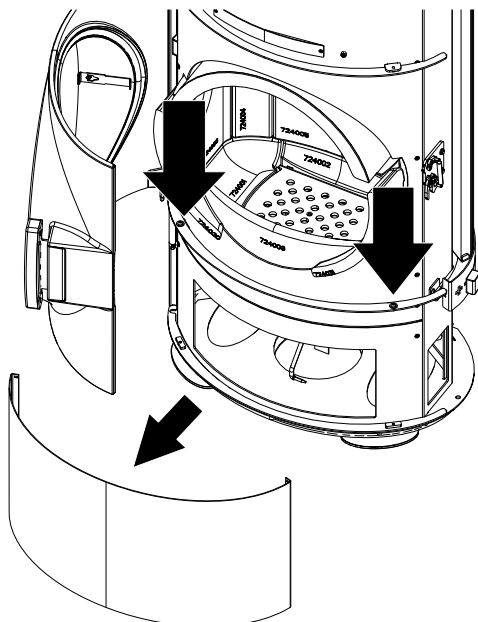
Fig. 27: Smontaggio del rivestimento anteriore
