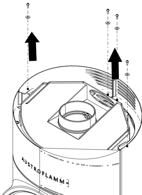
Fig. 37: Svitamento delle viti
