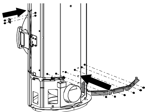
Fig. 15: Montaggio dei supporti dell'HMS
