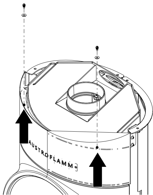
Fig. 22: Svitamento delle viti
