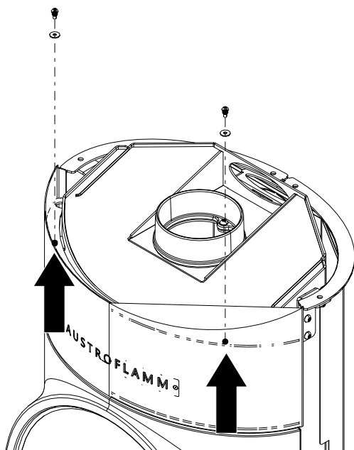
Fig. 39: Svitamento delle viti del rivestimento anteriore superiore
