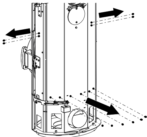
Fig. 14: Rimozione delle viti
