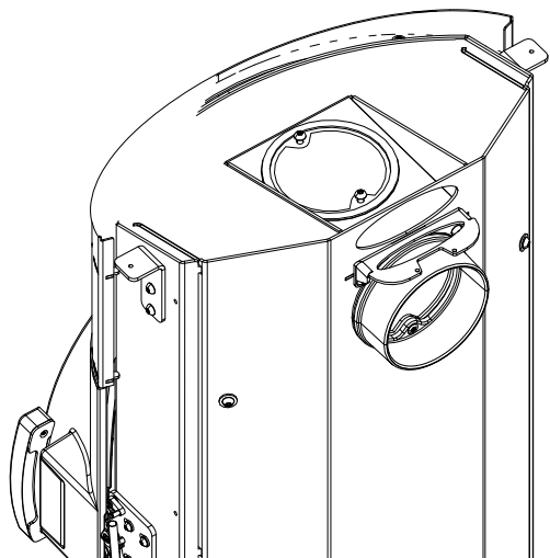
Fig. 9: Copertura e pezzo di collegamento sostituiti
