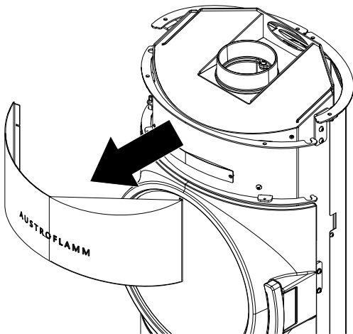
Fig. 41: Rimozione del rivestimento
