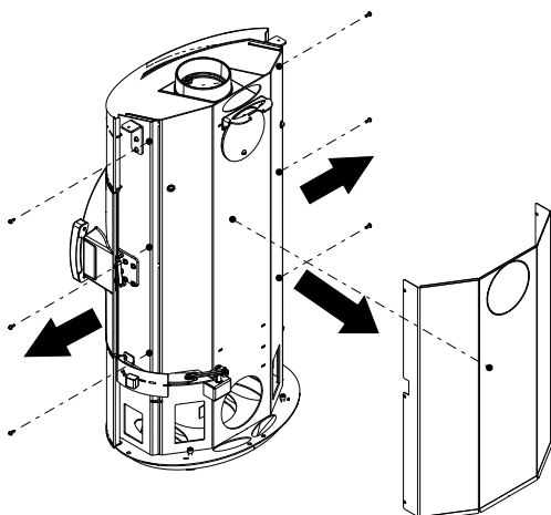
Fig. 6: Smontaggio della copertura
