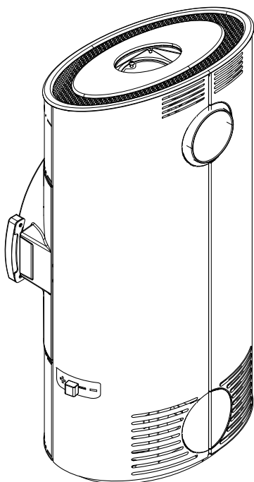
Fig. 10: Montaggio del rivestimento laterale e posizionamento del coperchio
