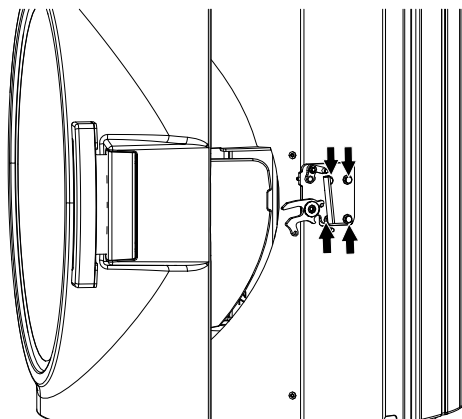
Fig. 26: Regolazione della serratura dello sportello
