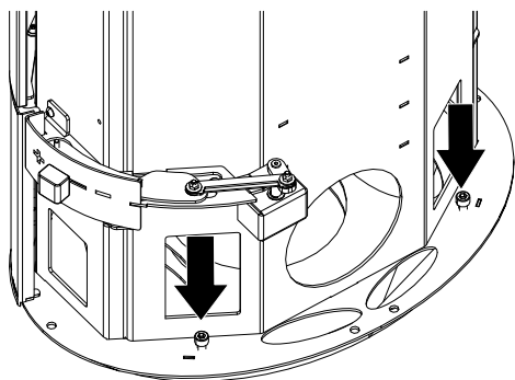
Fig. 21: Allineamento della stufa
