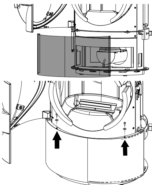
Fig. 19: Posizionamento del rivestimento inferiore anteriore
