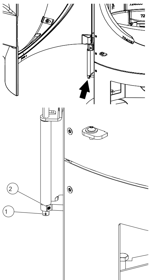
Fig. 28: Regolazione della forza di chiusura dello sportello
