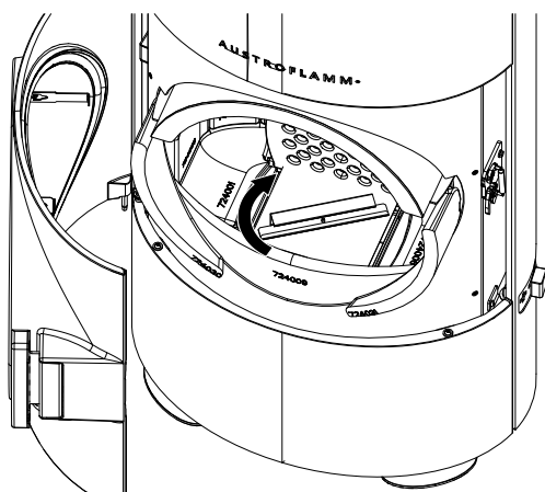
Fig. 33: Coperchio sul box cenere
