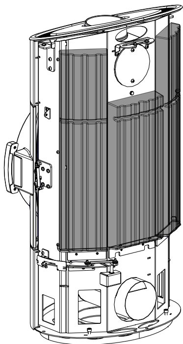
Fig. 16: Collocazione delle pietre HMS
