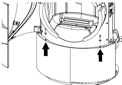
Fig. 42: Svitamento delle viti del rivestimento anteriore inferiore
