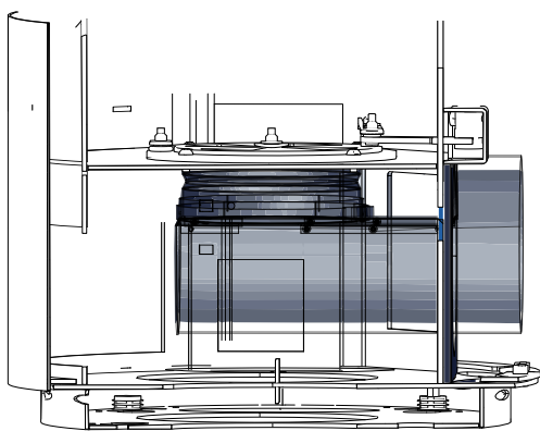
Fig. 18: Montaggio dell'adattatore dell'aria di alimentazione
