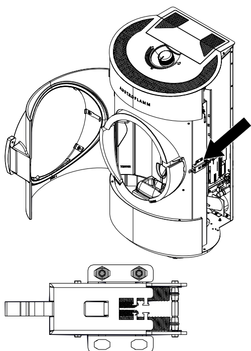
Fig. 21: Régler la serrure de la porte
