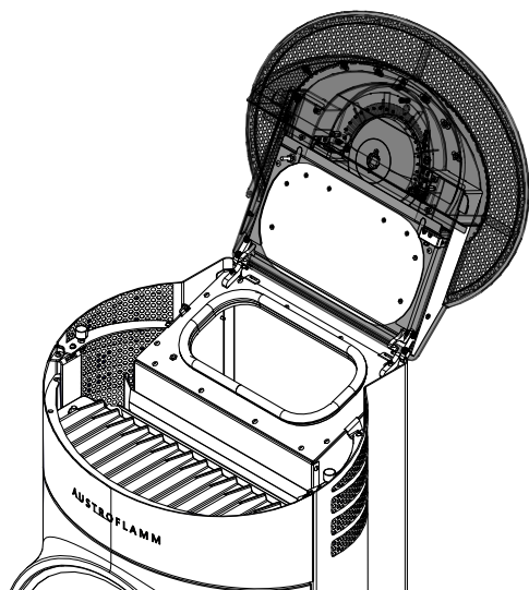
Fig. 40: Relever le couvercle de révision
