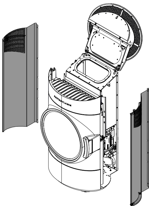
Fig. 42: Enlever l'habillage latéral
