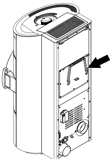
Fig. 24: Outil de levage
