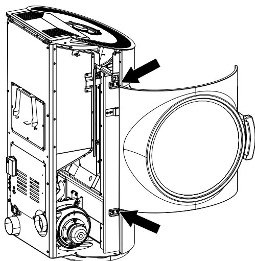
Fig. 18: Enlever l'habillage latéral
