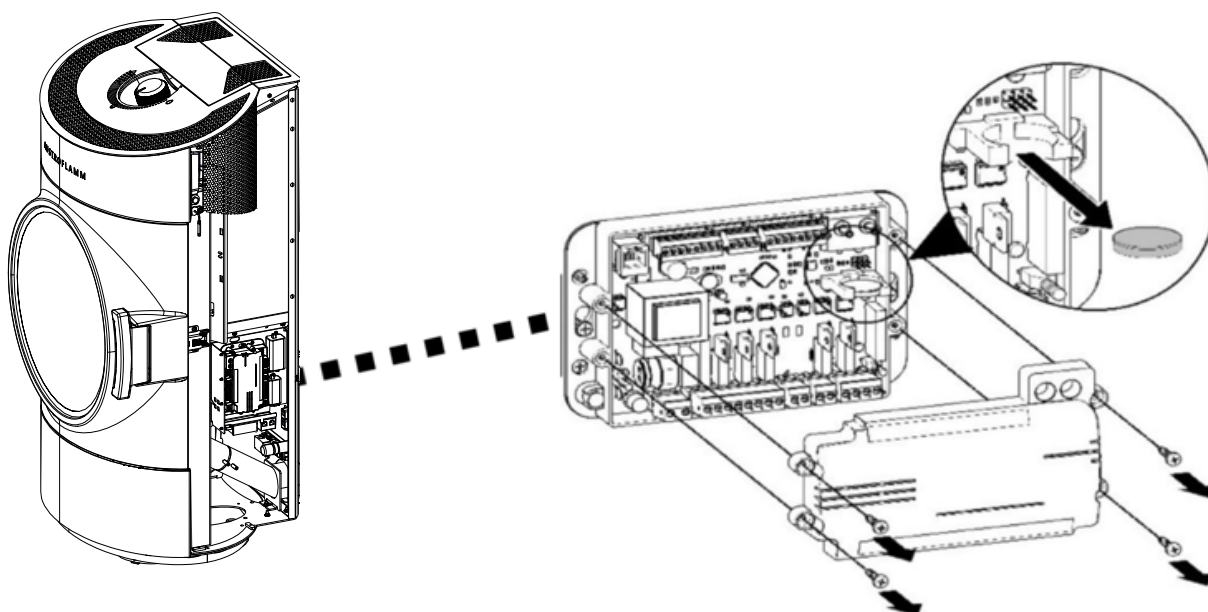
Fig. 23: Remplacer la pile mémoire
