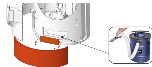
Fig. 34: Aspirer la zone des fumées
