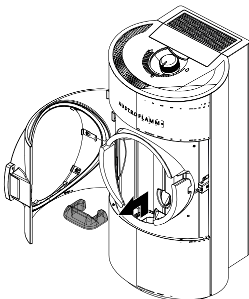
Fig. 25: Enlever la pierre en Keramott
