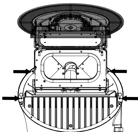
Fig. 41: Dévisser les vis
