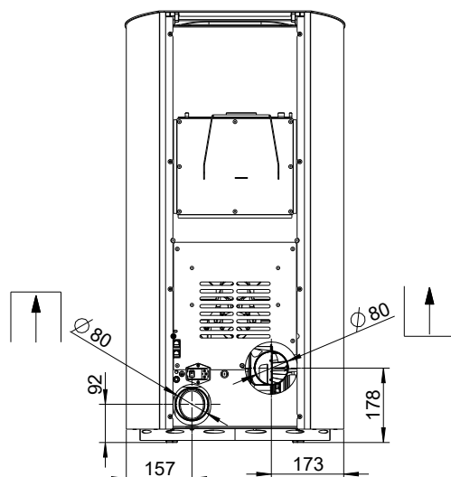
Fig. 9: Raccord par l'arrière
