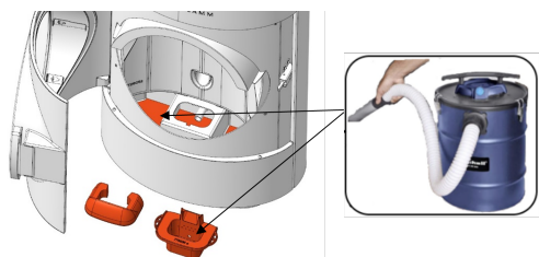
Fig. 27: Aspirer la chambre de combustion et le brasero
