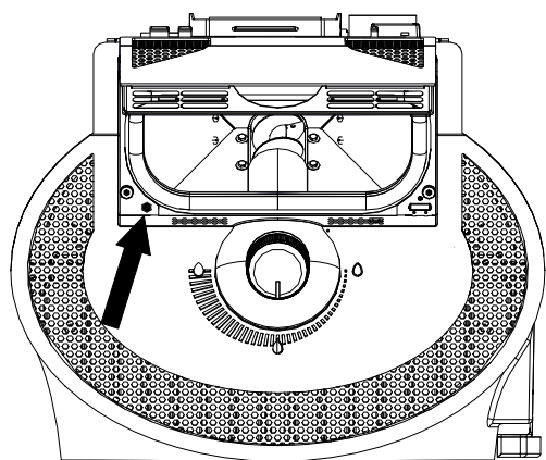
Fig. 29: Dévisser la vis Torx
