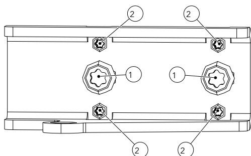
Fig. 19: Vis de réglage de la porte
