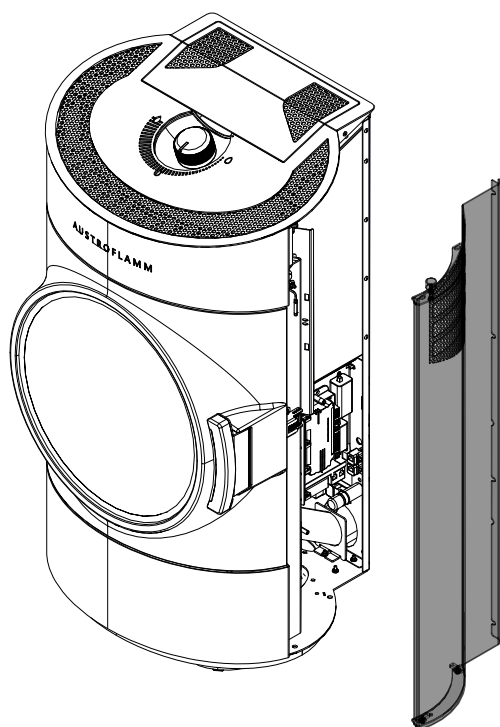
Fig. 22: Enlever l'habillage latéral
