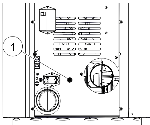
Fig. 35: Limiteur de température de sécurité
