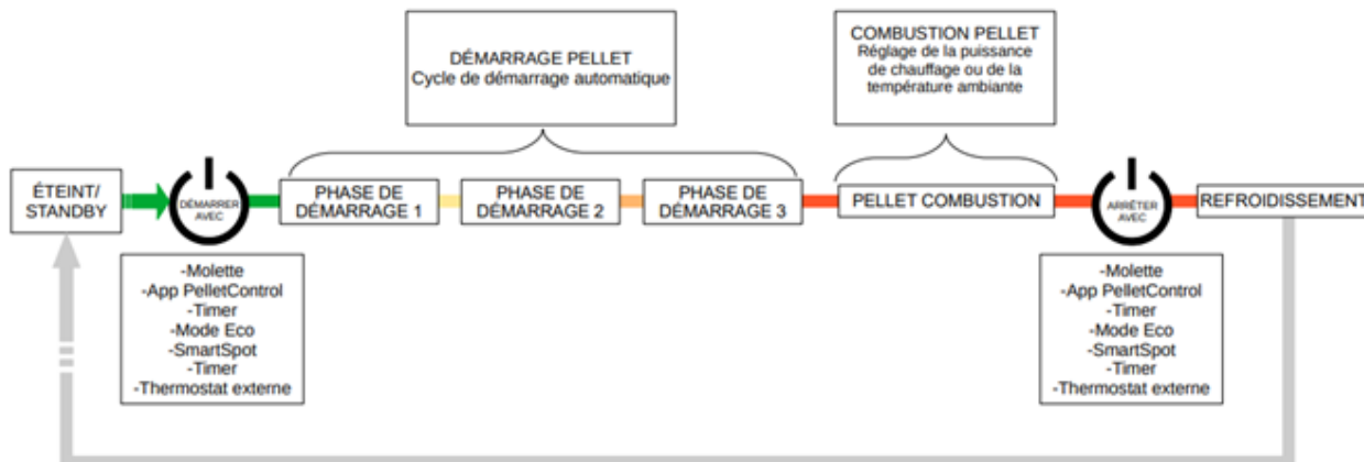
Fig. 15: Diagramme des fonctions
