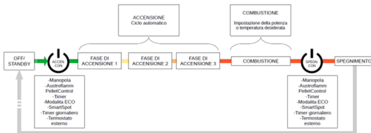
Fig. 15: Diagramma funzionale
