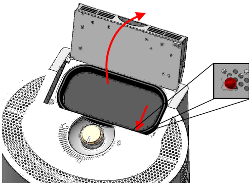
Fig. 11: Pulsante di Reset
