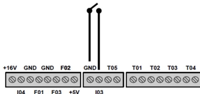
Fig. 17: Termostato esterno
