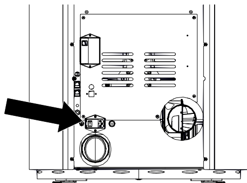
Fig. 36: Cassetto con fusibili in vetro T2,5A
