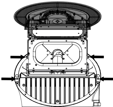
Abb. 42: Schrauben lösen
