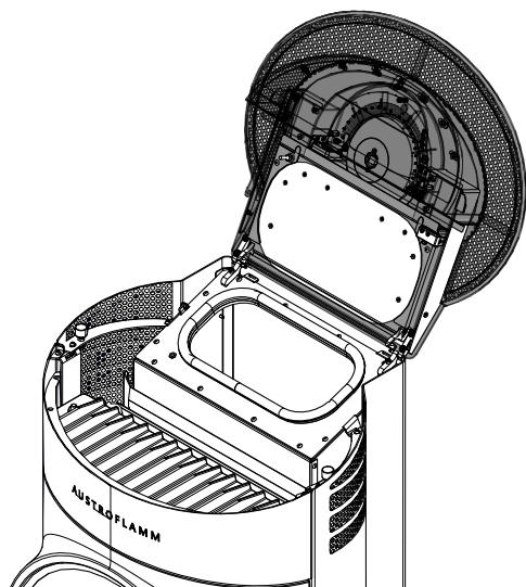
Abb. 32: Revisionsdeckel aufklappen
