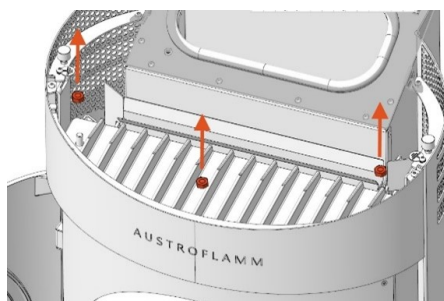
Abb. 33: Befestigungsschrauben abschrauben
