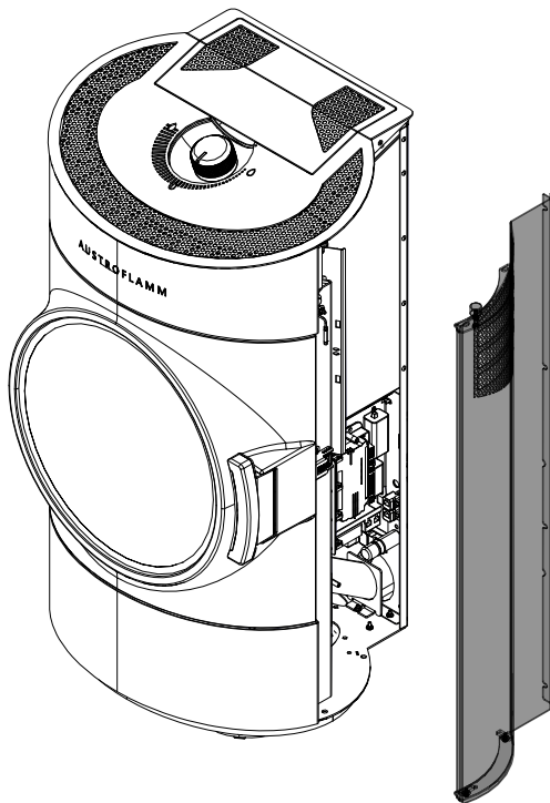
Abb. 23: Seitenverkleidung abnehmen
