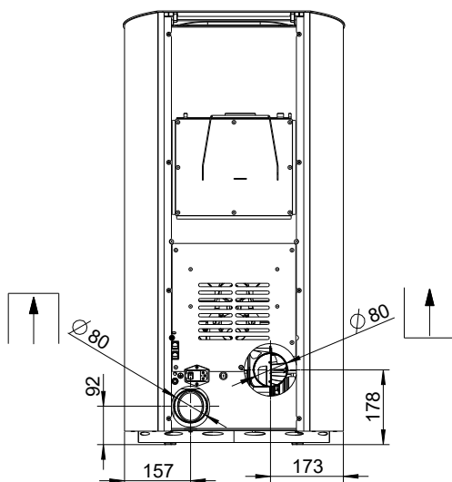
Abb. 10: Anschluss hinten
