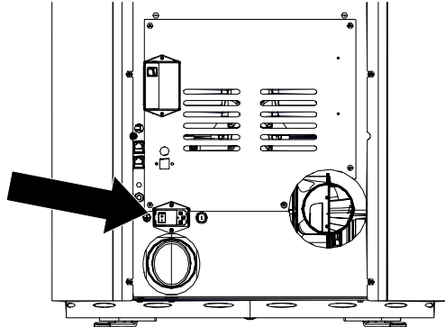
Abb. 37: Sicherungseinschub mit T2,5A-Glasrohrsicherungen
