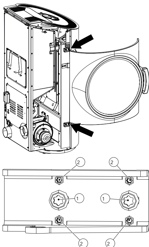
Abb. 20: Türeinstellschrauben
