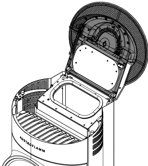
Abb. 41: Revisionsdeckel aufklappen
