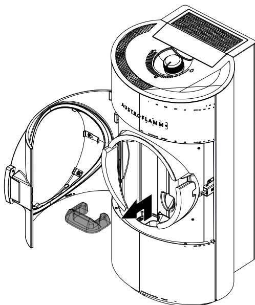
Abb. 26: Keramott-Stein entfernen
