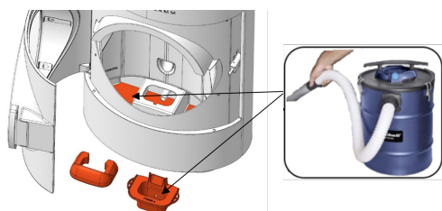
Abb. 28: Feuerraum und Brenntopf aussagen
