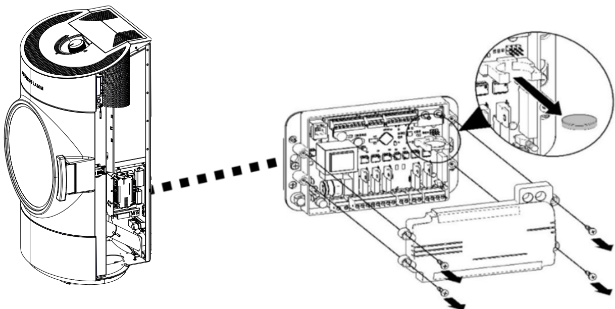
Abb. 24: Speicherbatterie tauschen
