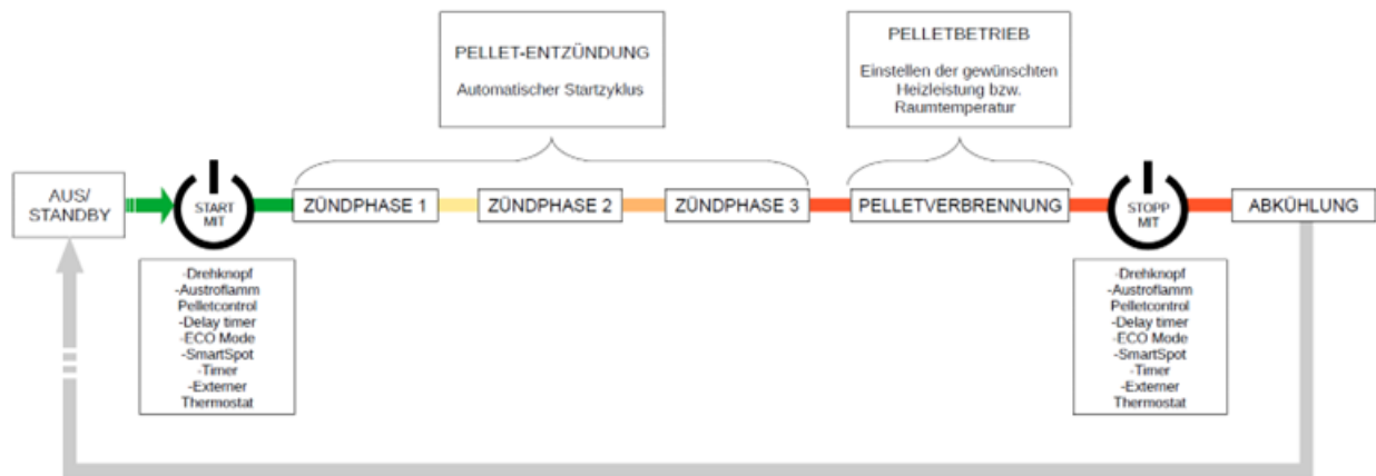
Abb. 16: Funktionsdiagramm
