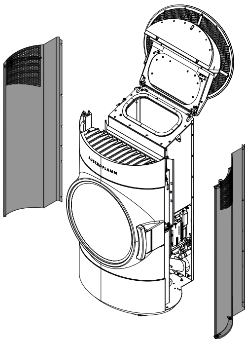
Abb. 43: Seitenverkleidung abnehmen
