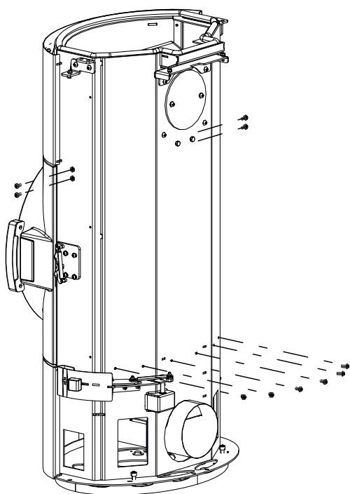
Fig. 21: Dévisser les vis préinstallées
