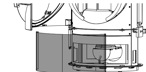
Fig. 27: Installer l'adaptateur d'arrivée d'air
