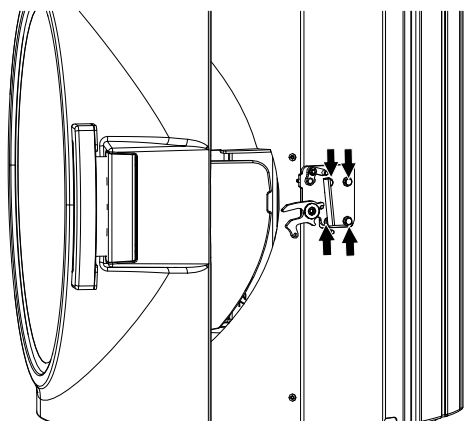
Fig. 39: Régler la serrure de la porte
