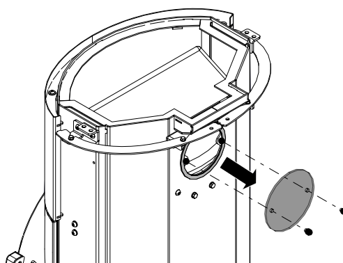
Fig. 18: Enlever le couvercle par l'arrière
