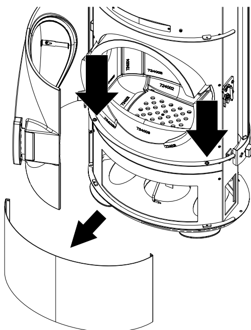
Fig. 37: Déposer l'habillage avant inférieur
