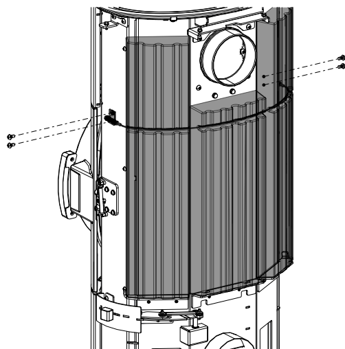
Fig. 24: Installer les pierres HMS
