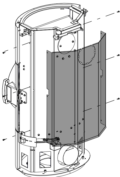
Fig. 17: Déposer la protection contre le rayonnement
