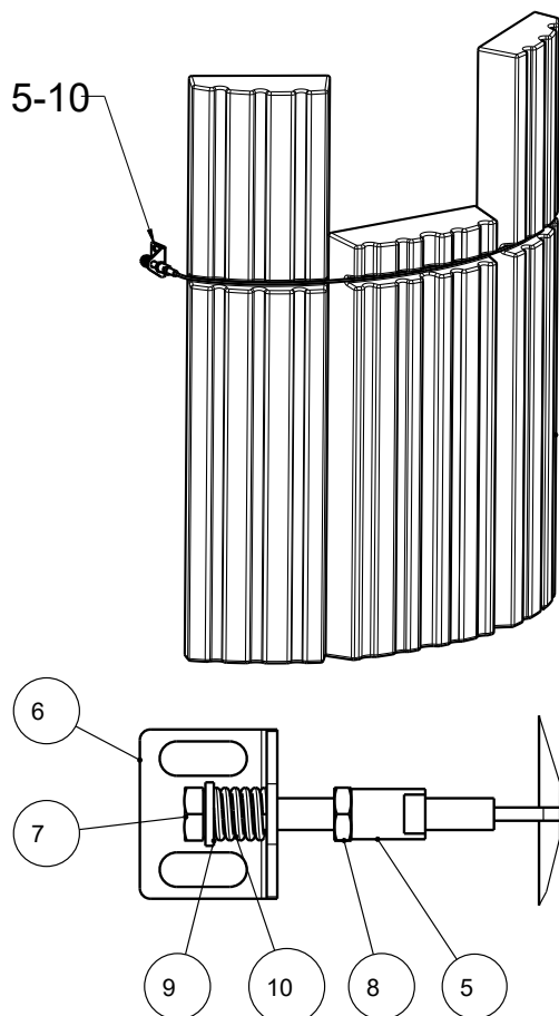
Fig. 24: Fixer le câble
