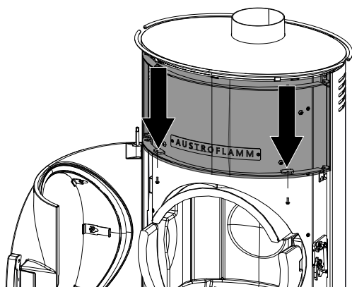
Fig. 32: Installer le capot avant
