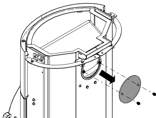
Fig. 19: Enlever le couvercle par l'arrière
