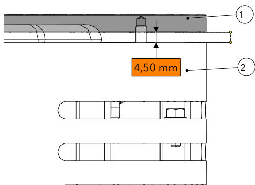
Fig. 11: Espacement entre plaque de cuisson et corps de l'appareil
