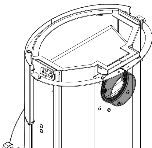
Fig. 20: Installer la tubulure de fumées à l'arrière
