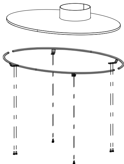
Fig. 7: Installer la main-courante (vue de dessous)
