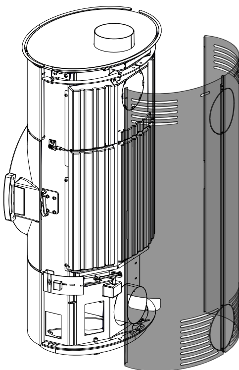
Fig. 50: Enlever l'habillage latéral
