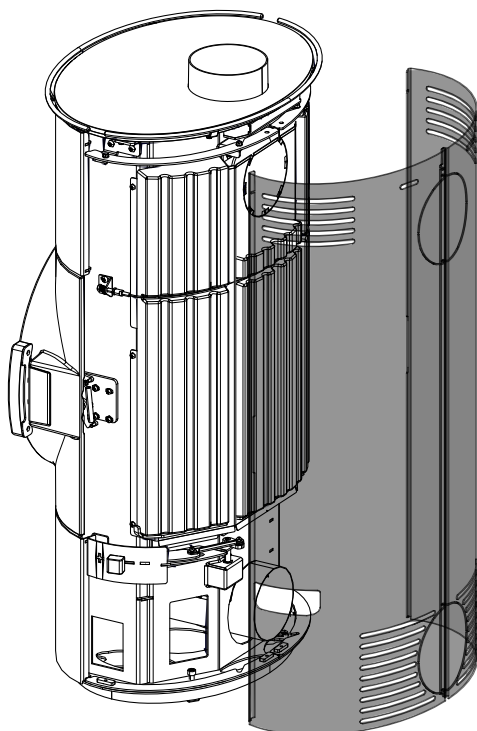
Fig. 30: Poser le capot latéral
