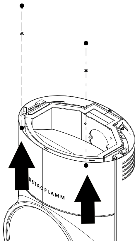
Fig. 35: Dévisser les vis
