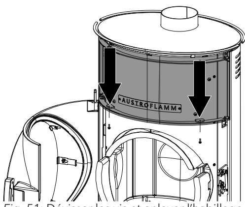
Fig. 51: Dévisser les vis et enlever l'habillage
