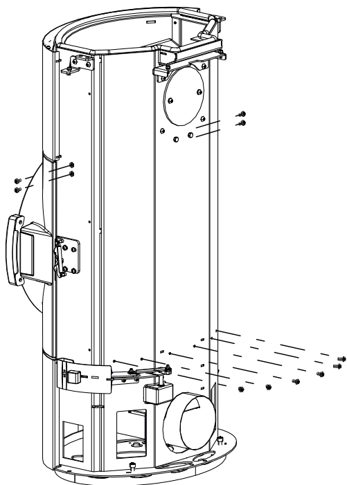
Fig. 22: Dévisser les vis préinstallées
