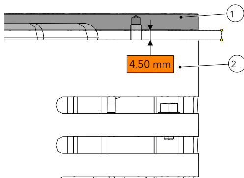
Fig. 14: Espacement entre plaque de cuisson et corps de l'appareil
