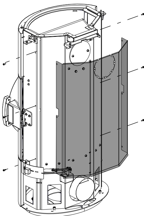
Fig. 21: Déposer la protection contre le rayonnement
