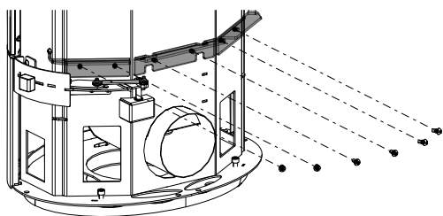
Fig. 23: Installer les fixations HMS
