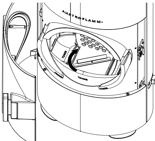
Fig. 46: Coperchio sul box cenere
