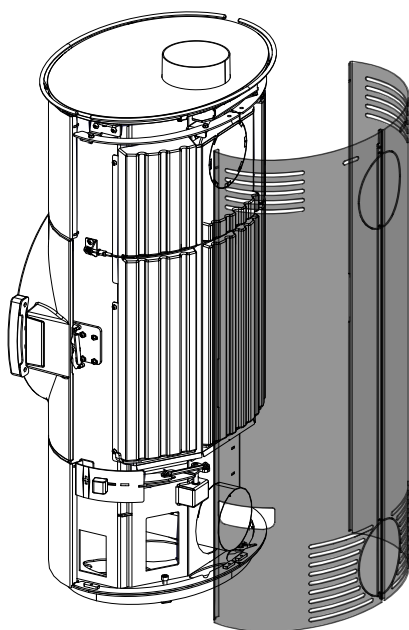
Fig. 30: Collocamento del rivestimento laterale
