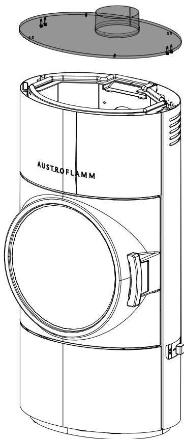
Fig. 14: Rimozione del coperchio
