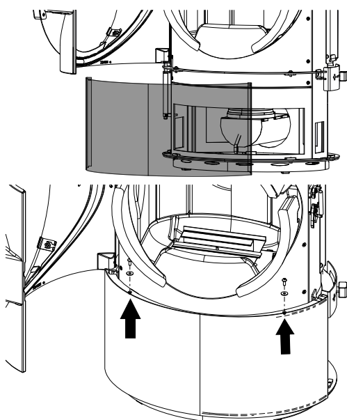
Fig. 33: Posizionamento del rivestimento inferiore anteriore
