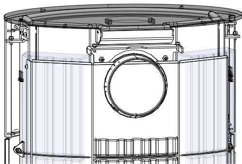
Fig. 9: Fissaggio della piastra riscaldante
