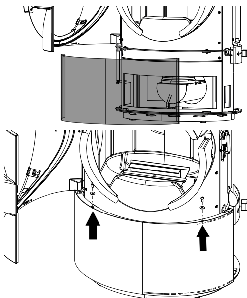
Fig. 28: Posizionamento del rivestimento inferiore anteriore
