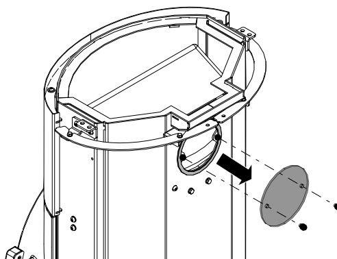
Fig. 18: Smontaggio del coperchio da dietro
