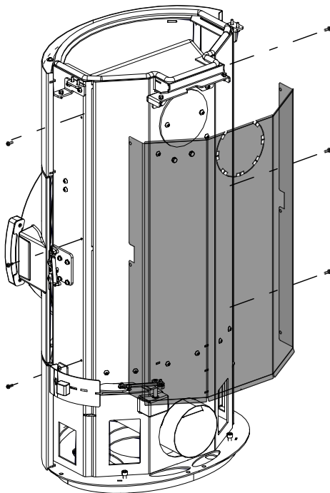
Abb. 21: Strahlungsschutz abmontieren
