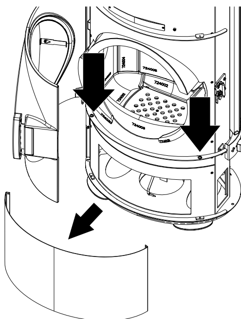
Abb. 38: unten vordere Verkleidung demon- tieren
