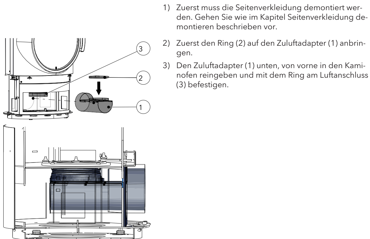
Abb. 28: Zuluftadapter montieren
