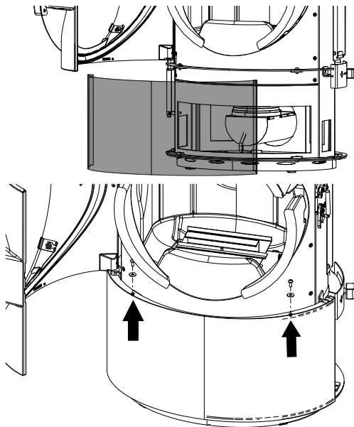
Abb. 29: Untere vordere Verkleidung anbringen
