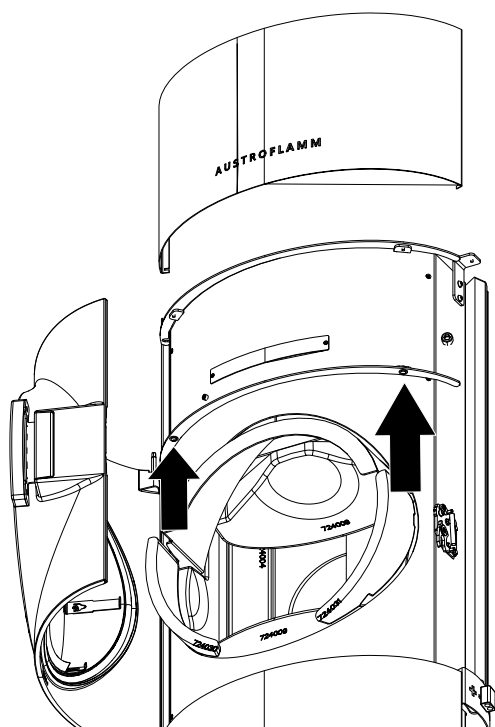
Abb. 37: obere vordere Verkleidung demon- tieren
