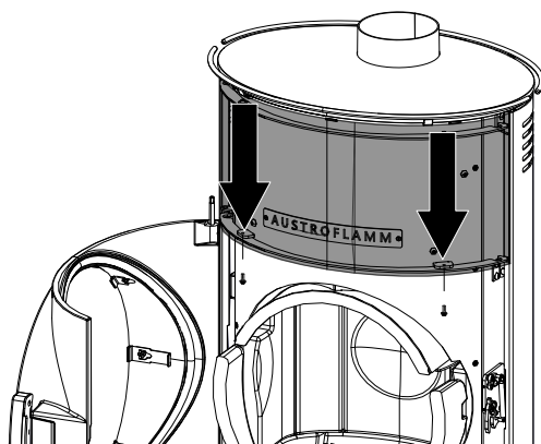
Abb. 52: Schrauben lösen und Verkleidung abnehmen
