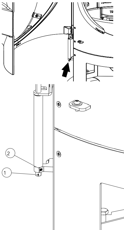
Abb. 42: Türschließkraft einstellen
