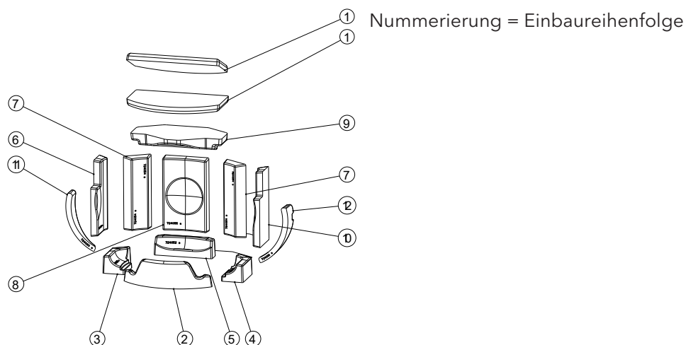
Abb. 27: Keramott einbauen
