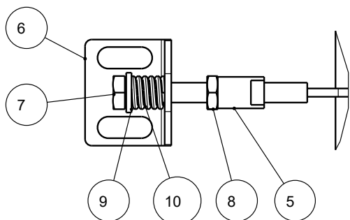
Abb. 24: Seil befestigen
