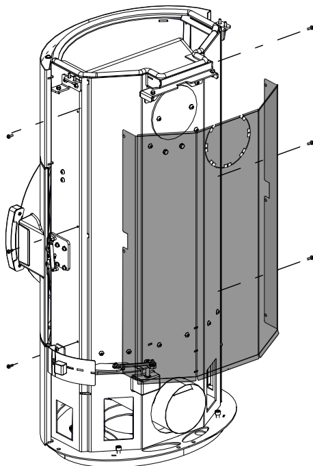
Abb. 17: Strahlungsschutz abmontieren
