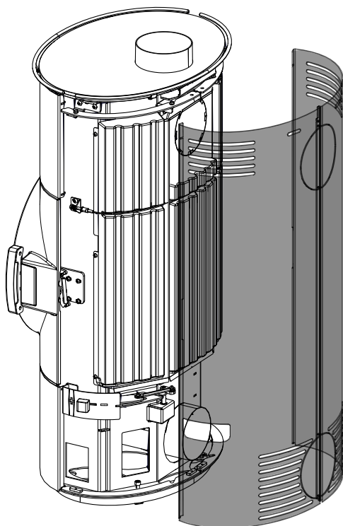
Abb. 31: Seitenverkleidung anbringen
