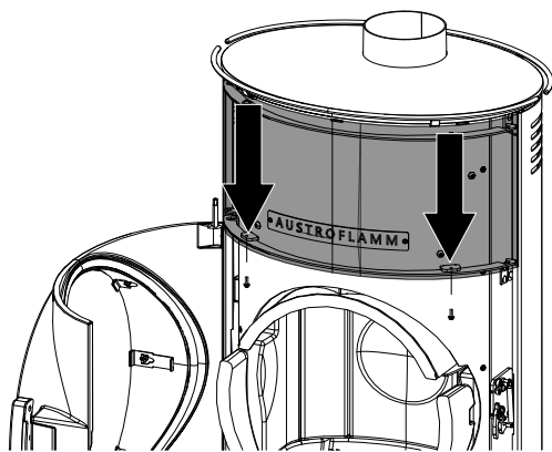
Abb. 33: Vordere Verkleidung montieren
