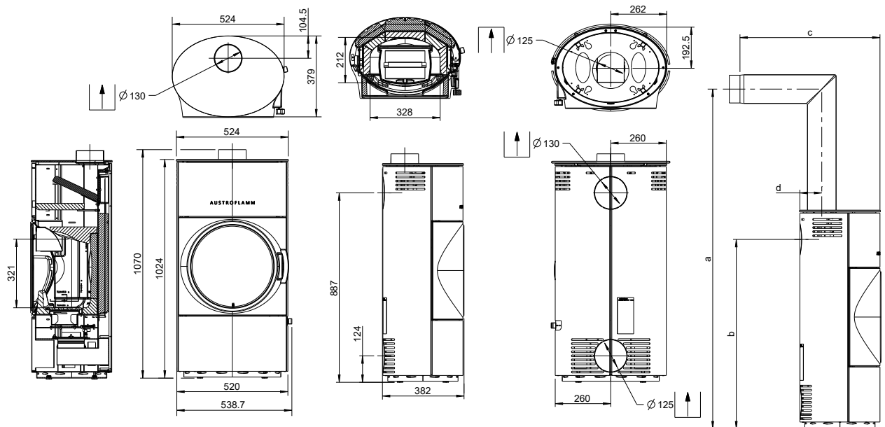
Abb. 2: Abmessungen
