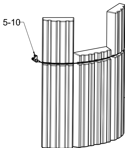
Abb. 23: HMS-Halter montieren
