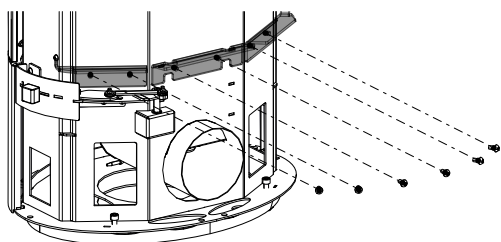
Abb. 23: HMS-Halter montieren
