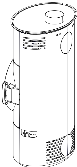
Abb. 12: Seitenverkleidung montieren
