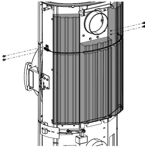
Abb. 25: HMS-Steine montieren
