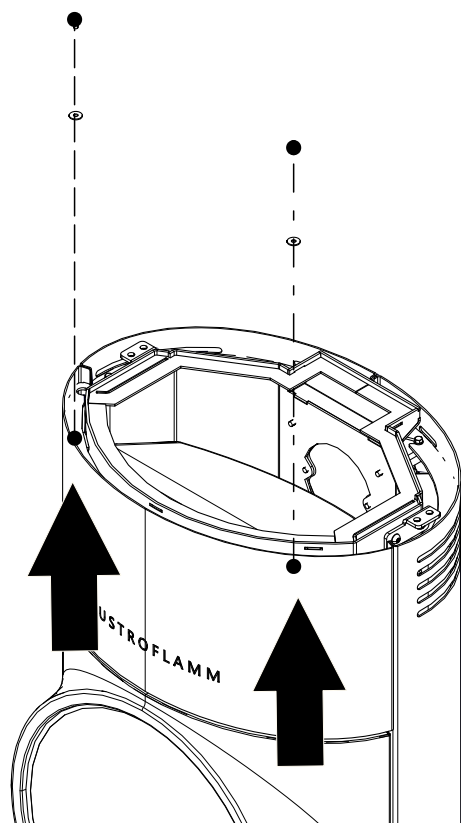
Abb. 36: Schrauben lösen
