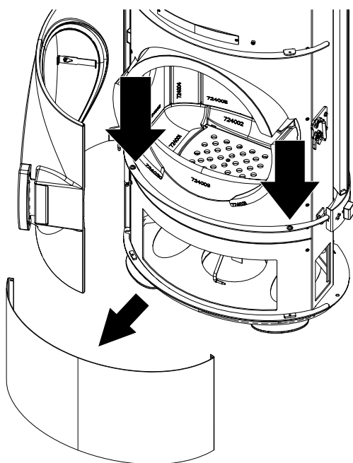
Abb. 29: unten vordere Verkleidung demon- tieren
