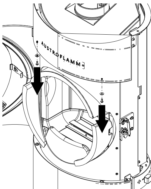
Abb. 13: Schrauben lösen
