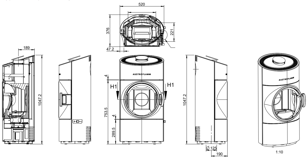
Abb. 2: Abmessungen
