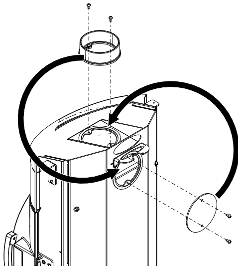
Abb. 20: Abdeckung und Stützen tauschen
