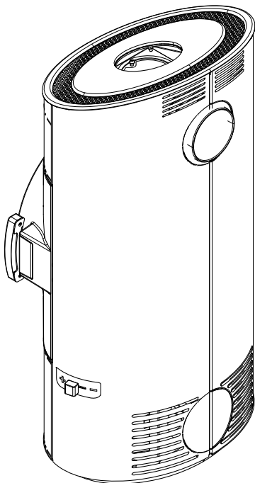
Abb. 22: Seitenverkleidung montieren und Deckel anbringen
