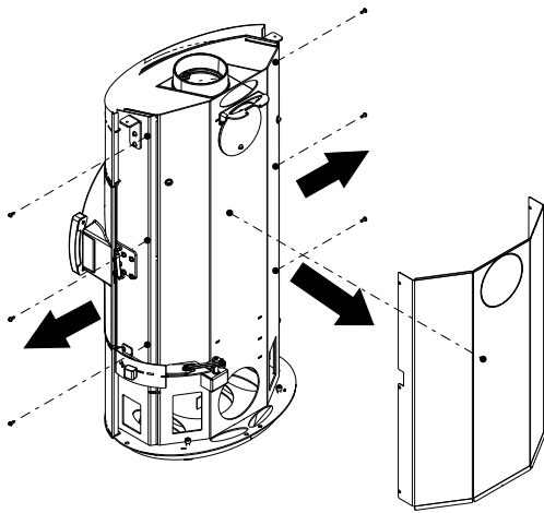
Abb. 18: Abdeckung demontieren
