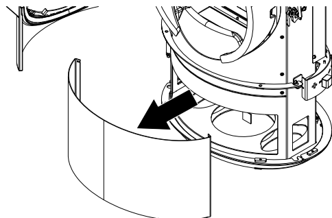
Abb. 16: Untere Blende abnehmen
