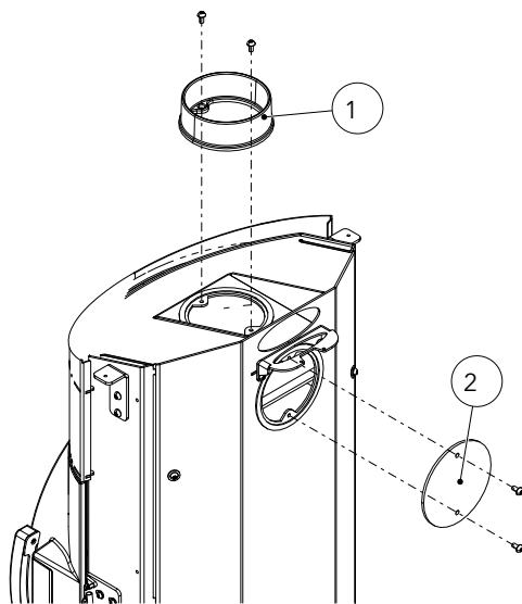
Abb. 19: Rauchrohrstutzen und Abdeckung demontieren
