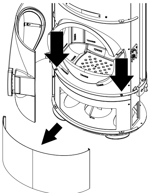
Abb. 32: Unten vordere Verkleidung demonstrieren
