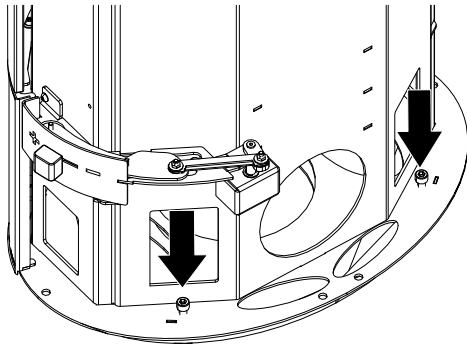
Abb. 26: Kaminofen ausrichten
