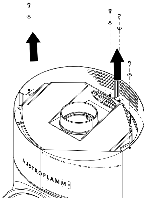
Abb. 10: Schrauben lösen
