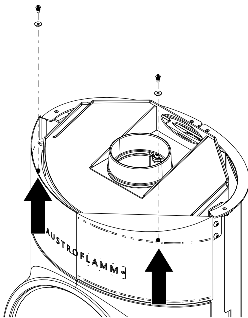
Abb. 27: Schrauben lösen
