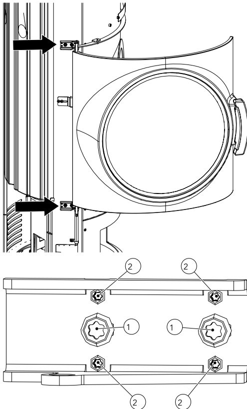
Abb. 30: Türeinstellschrauben
