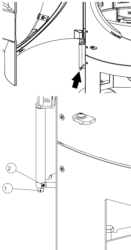
Abb. 33: Türschließkraft einstellen
