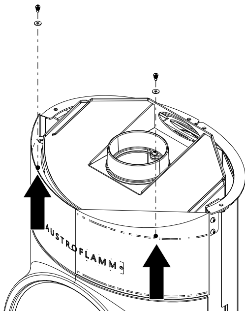
Abb. 12: Schrauben der oberen, vorderen Verkleidung lösen
