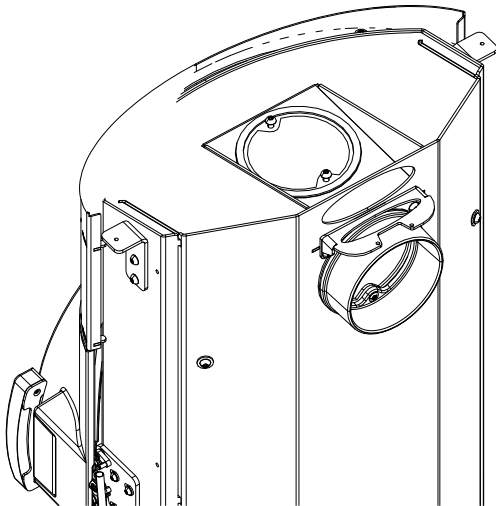
Abb. 21: Abdeckung und Stützen vertauscht
