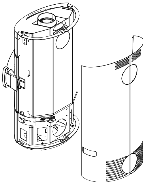
Abb. 11: Seitenverkleidung abnehmen
