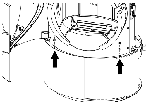
Abb. 15: Schrauben der unteren, vorderen Verkleidung lösen
