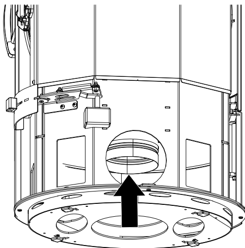
Abb. 24: Aluflexschlauch befestigen
