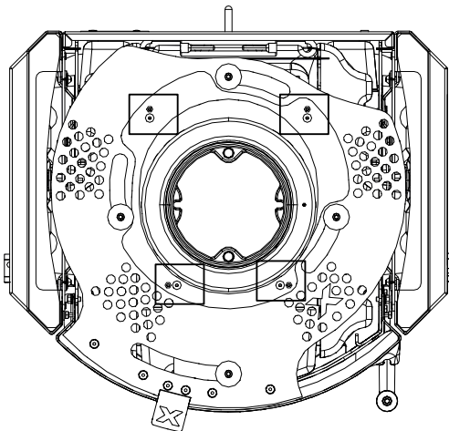
Fig. 42: Aérateur vu du dessus
