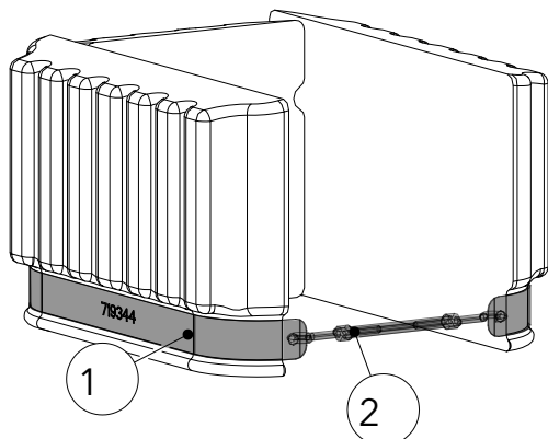
Fig. 23: Installer la bande de fixation
