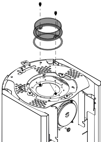
Fig. 27: Smontaggio della presa della canna fumaria.
