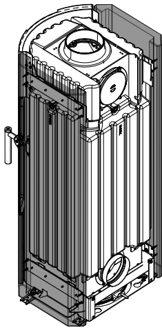
Fig. 25: Agganciamento del rivestimento laterale
