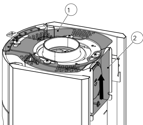
Fig. 20: Rimozione del pannello di protezione dal calore
