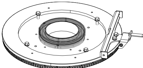
Fig. 35: Inserimento dell'adattatore di tenuta
