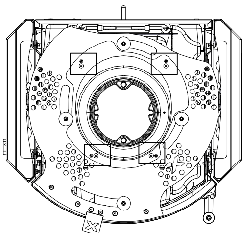
Fig. 42: Ventola dall'alto
