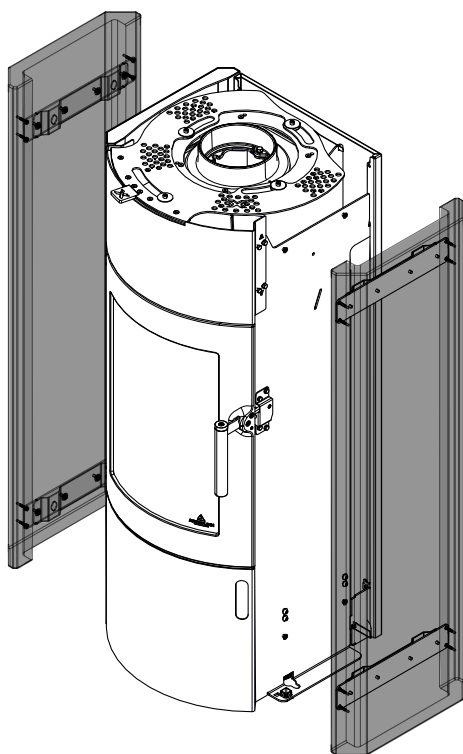
Fig. 50: Sganciamento del rivestimento laterale
