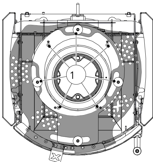
Fig. 19: Svitamento delle viti della ventola
