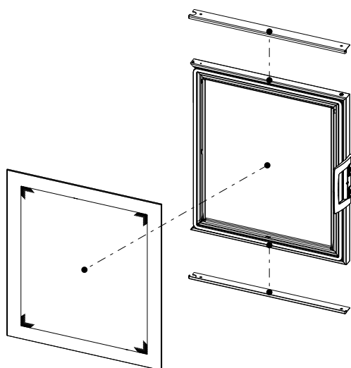
Fig. 24: Smontare tutte le parti
