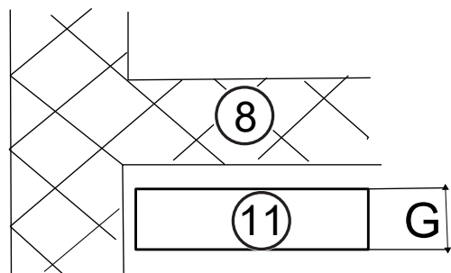
Fig. 16: Soffitto sopra l'inserto per caminetti
