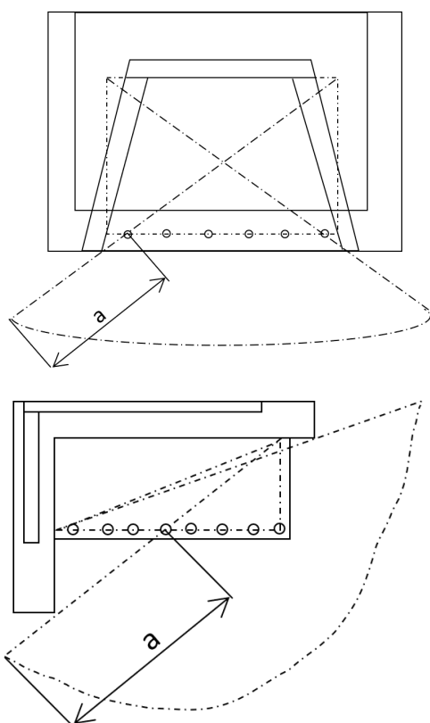
Fig. 8: Misura "a" secondo i Dati tecnici (distanza di sicurezza anteriore)
