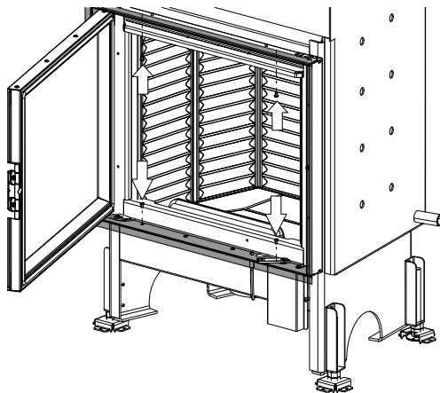
Abb. 29: Designrahmen befestigen
