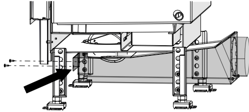
Abb. 31: Flachknie anbringen
