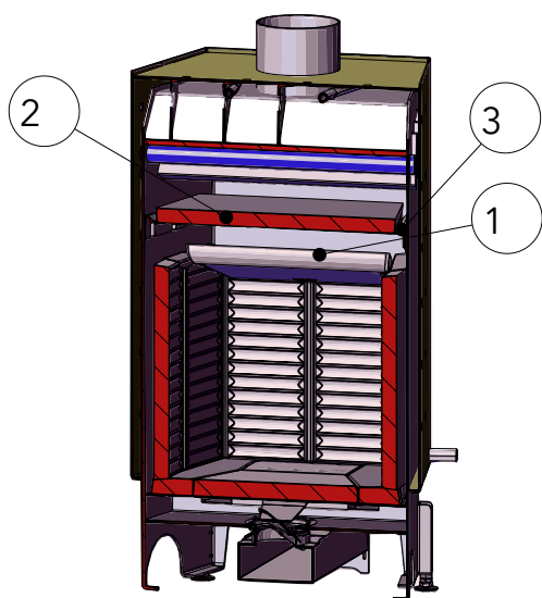
Abb. 22: Umlenkplatte einbauen
