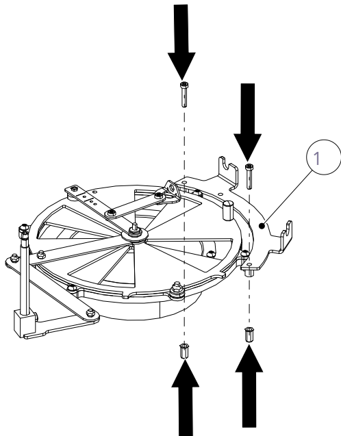
Abb. 57: Montageset montieren
