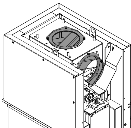
Abb. 25: Rauchrohranschluss umbauen
