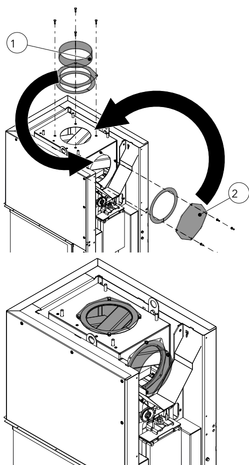
Abb. 25: Rauchrohranschluss umbauen
