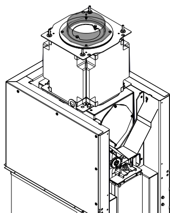
Abb. 30: Rauchrohrstutzen montieren
