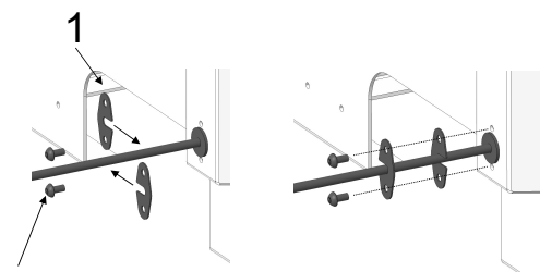
Abb. 62: Flansch Bowdenzug
