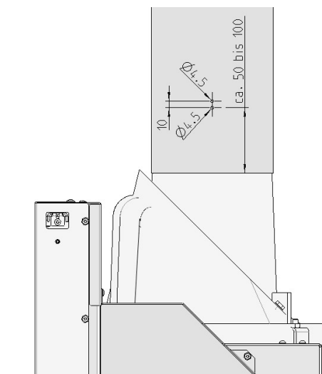
Abb. 52: Bohrschema-Rauchrohr
