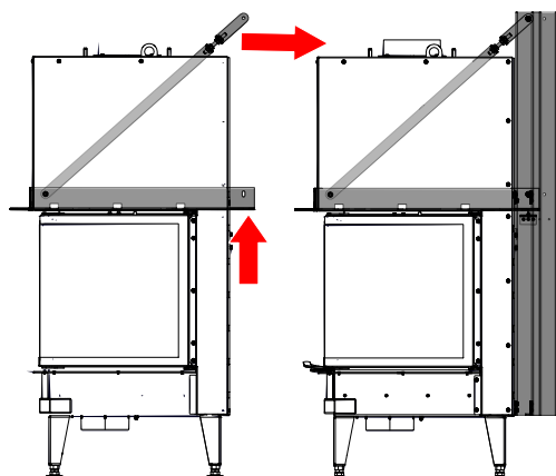
Abb. 48: Tragrahmen ausrichten
