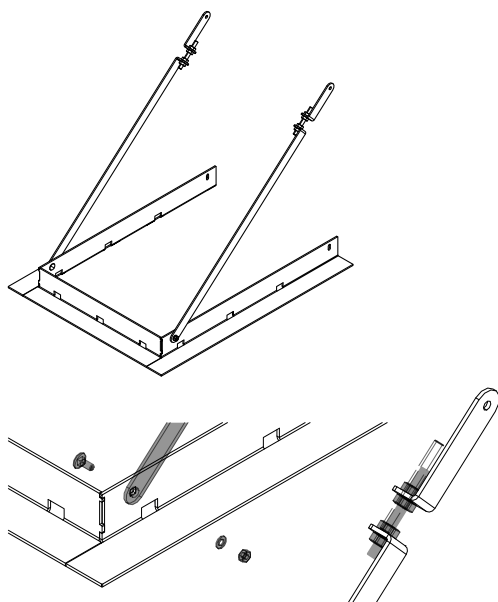
Abb. 38: Designrahmen zusammenbauen
