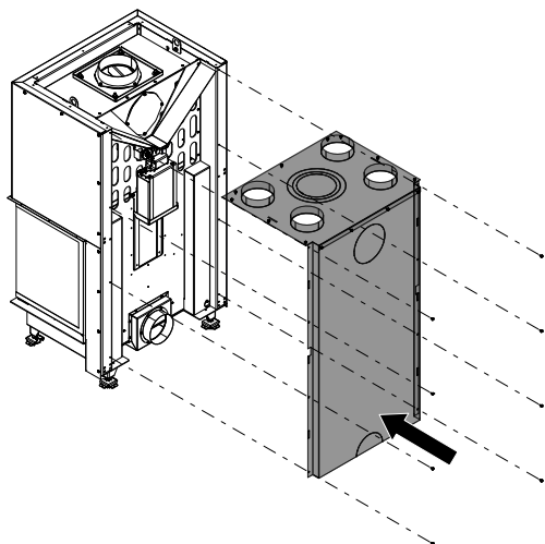
Abb. 32: KV-Mantel montieren
