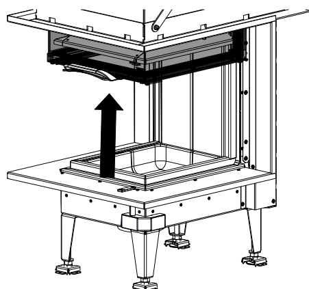
Abb. 23: Tür öffnen
