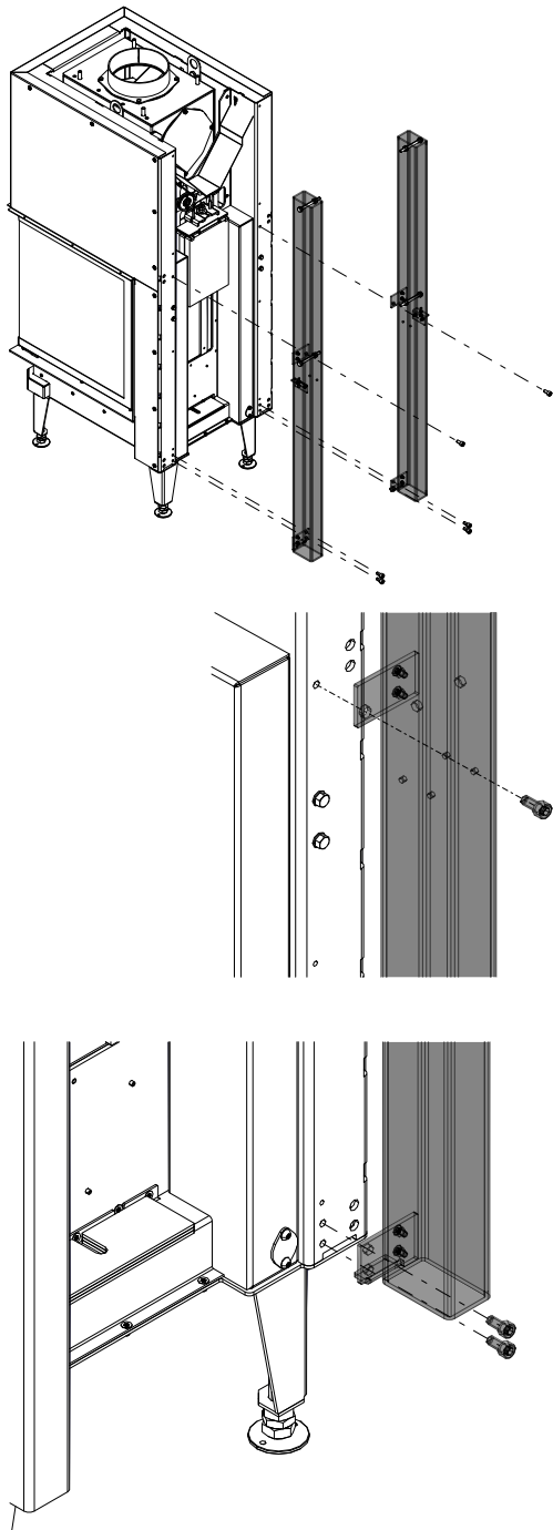
Abb. 49: Traggestell montieren
