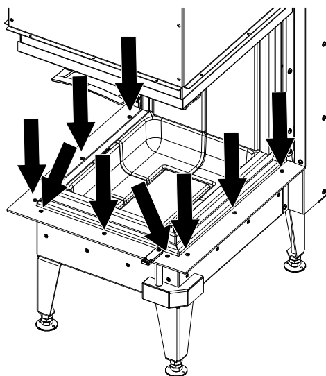
Abb. 34: Gewinde lösen
