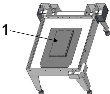
Abb. 56: Keramik Auflageblech entfernen
