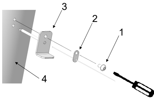
Abb. 53: Temperatur-Sensor montieren
