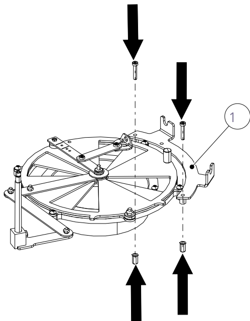
Abb. 57: Montageset montieren
