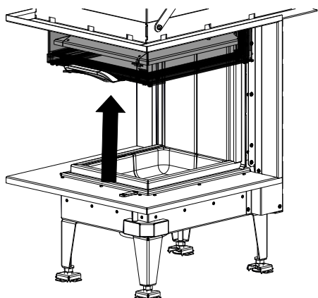
Fig. 22: Ouvrir la porte
