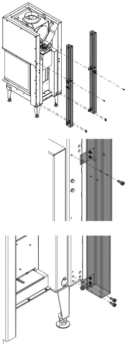
Fig. 48: Installer le châssis porteur
