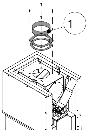
Fig. 27: Démonter la tubulure de fumées
