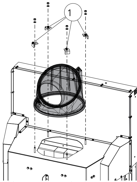
Abb. 29: Rauchsammler abmontieren
