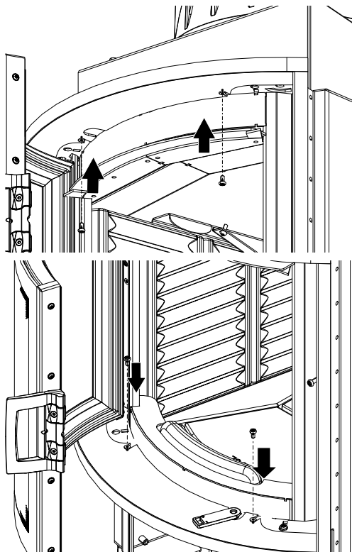
Abb. 88: Designrahmen befestigen
