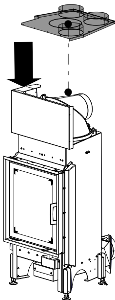
Abb. 68: KV-Deckel montieren
