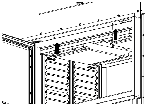
Abb. 94: Designrahmen oben befestigen
