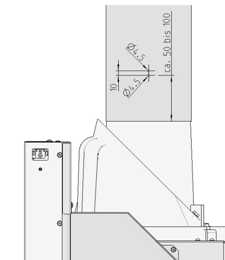
Abb. 49: Bohrschema-Rauchrohr
