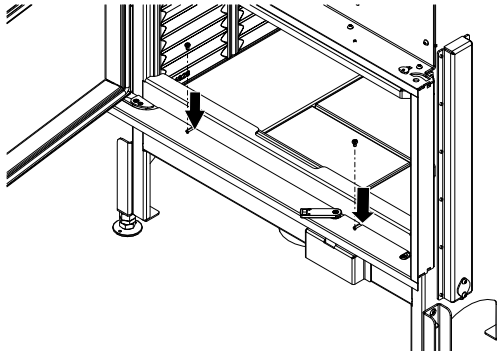
Abb. 91: Designrahmen unten befestigen
