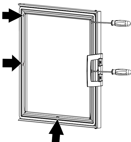
Abb. 25: Laschen aufbiegen
