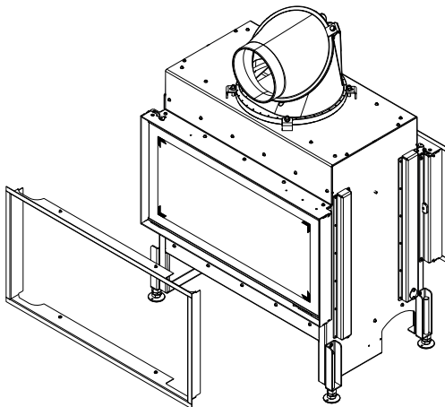
Abb. 92: Designrahmen auf Rückseite positionieren
