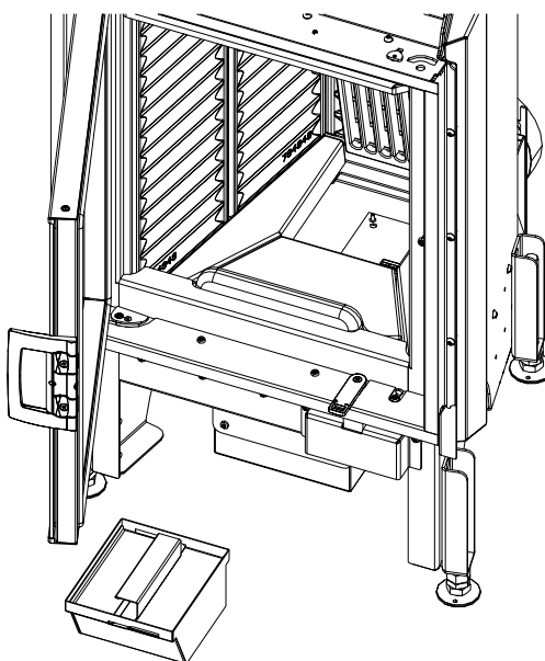
Abb. 109: Aschebox rausnehmen und entleeren
