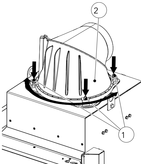
Abb. 102: Rauchsammler in gewünschte Position drehen
