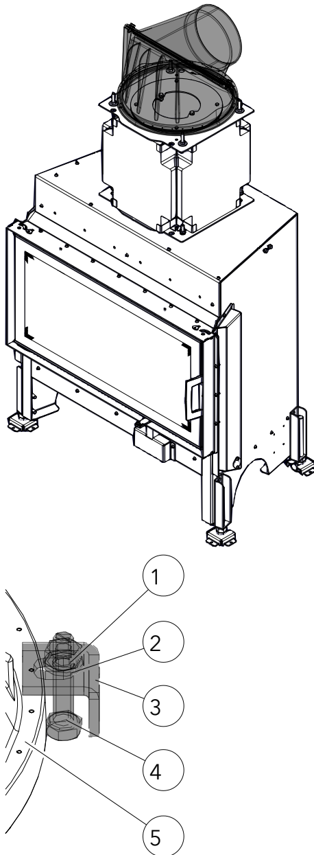
Abb. 45: Abgassammler montieren
