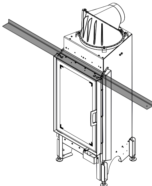
Abb. 96: Tragrahmen montieren
