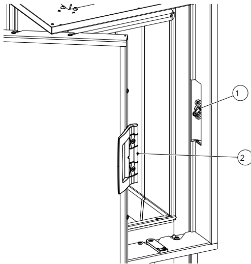
Abb. 101: Tür einstellen
