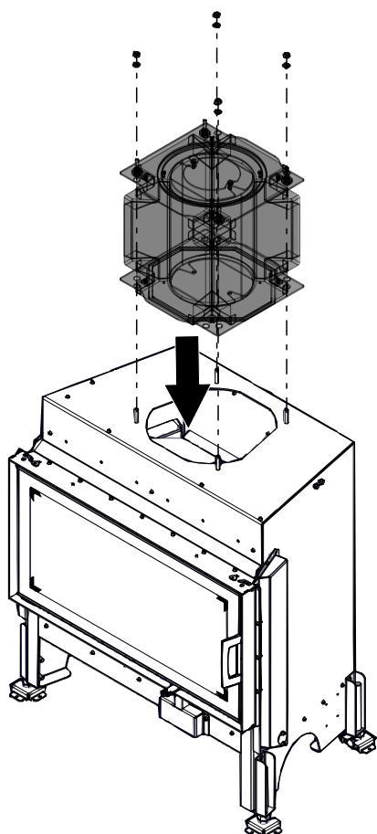
Abb. 44: Speicherbox klein aufsetzen
