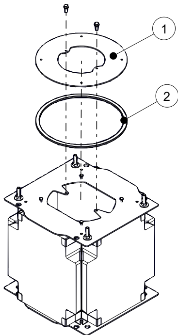
Abb. 42: Dichtung und Adapterblech entfernen
