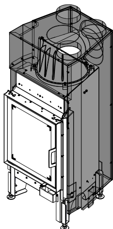
Abb. 72: KVM montiert
