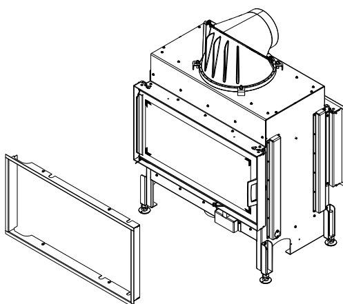
Abb. 89: Designrahmen positionieren
