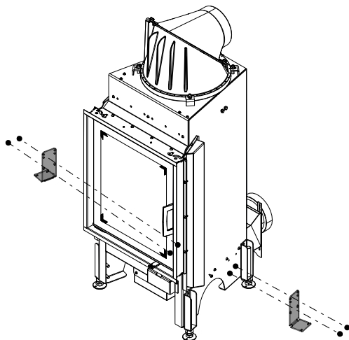
Abb. 63: Halterung links und rechts montieren
