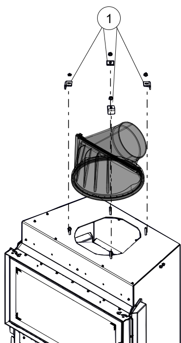
Abb. 43: Rauchsammler abmontieren
