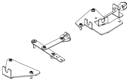
Abb. 47: Montageset 363000
