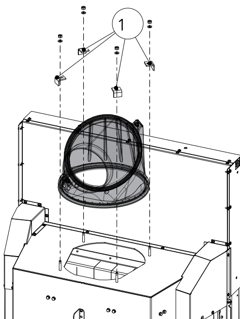
Abb. 36: Rauchsammler abmontieren
