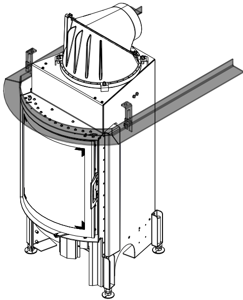
Abb. 97: Tragrahmen montieren
