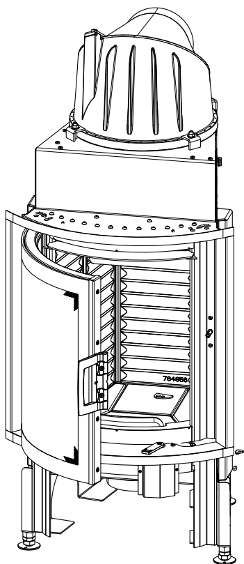
Abb. 86: Tür öffnen
