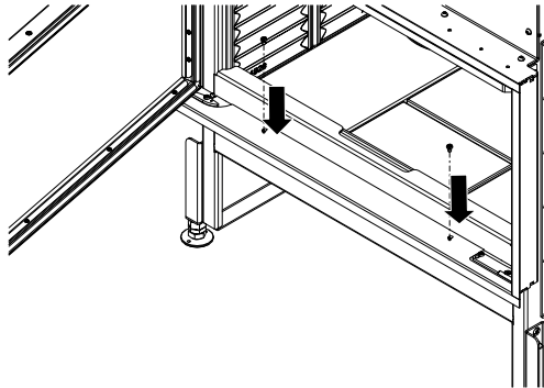
Abb. 95: Designrahmen unten befestigen
