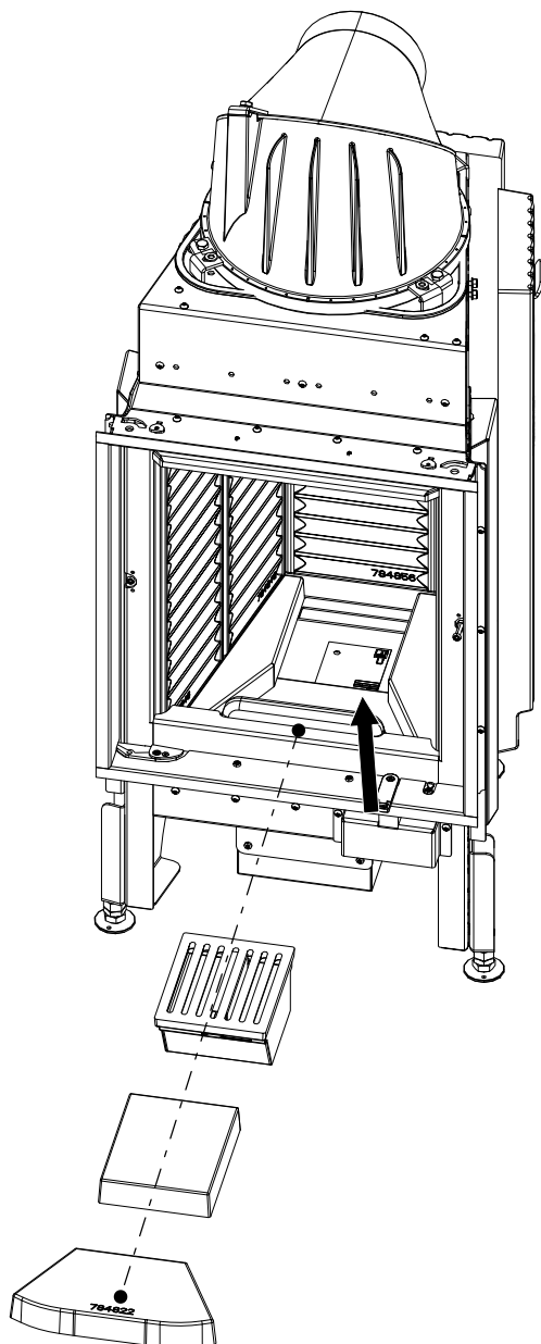
Abb. 98: Aschenkasten einlegen
