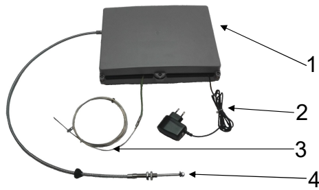
Abb. 46: Steuerungseinheit
