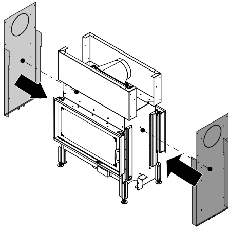
Abb. 77: KV-Wand links und rechts anbringen
