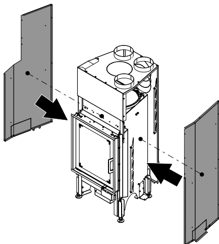
Abb. 69: KV-Wand rechts und links anbringen
