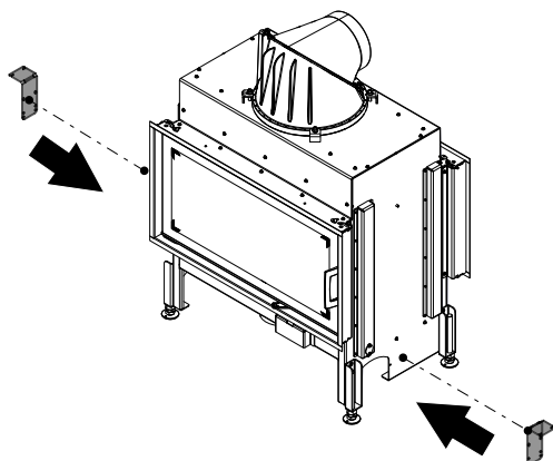
Abb. 73: Halterung links und rechts montieren
