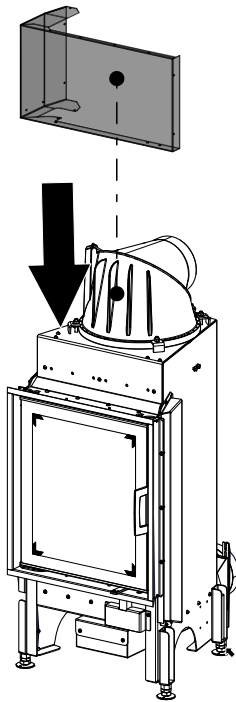
Abb. 67: KV-Wand vorne montieren
