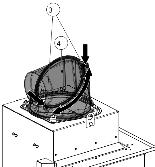
Abb. 103: Rauchsammlerstutzen einstellen
