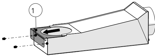
Abb. 39: Schrauben lösen
