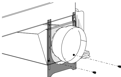
Abb. 41: Befestigung montieren
