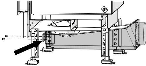
Abb. 40: Flachknie anbringen
