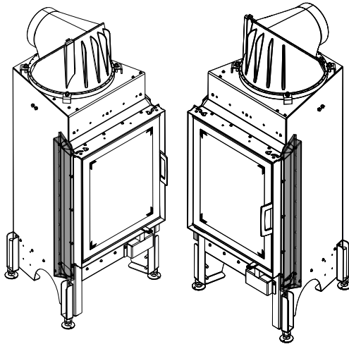
Abb. 51: Bohrung für Bowdenzug
