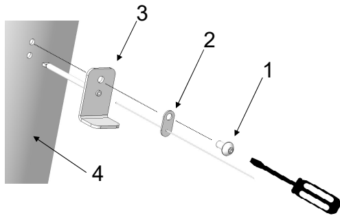
Abb. 50: Temperatur-Sensor montieren
