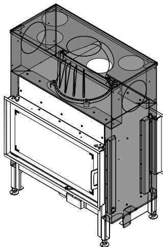
Abb. 80: KVM montiert
