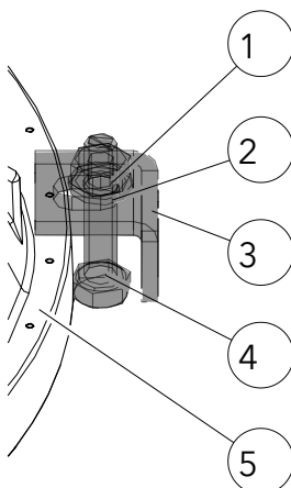
Abb. 38: Abgassammler montieren
