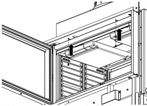
Abb. 90: Designrahmen oben befestigen
