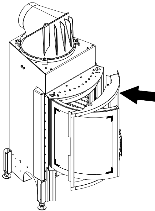
Abb. 87: Designrahmen einsetzen
