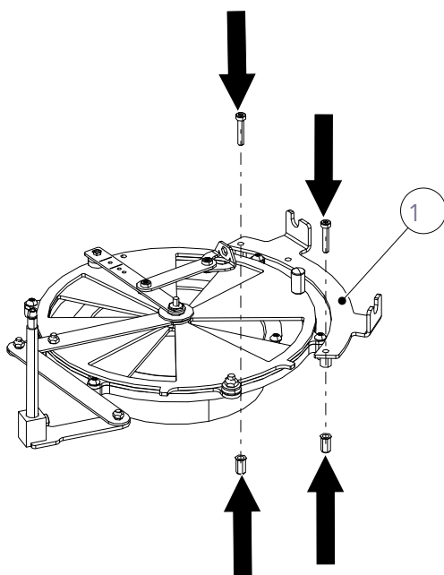
Abb. 55: Montageset montieren
