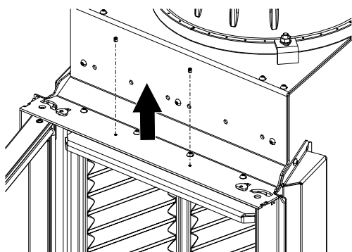
Abb. 82: Bolzen oben rausdrehen
