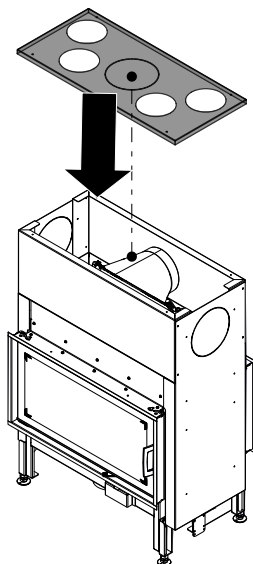
Abb. 79: KV-Deckel montieren
