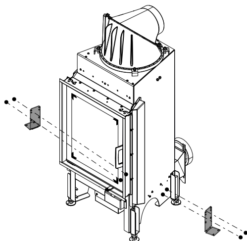
Fig. 62: Installer les fixations gauche et droite
