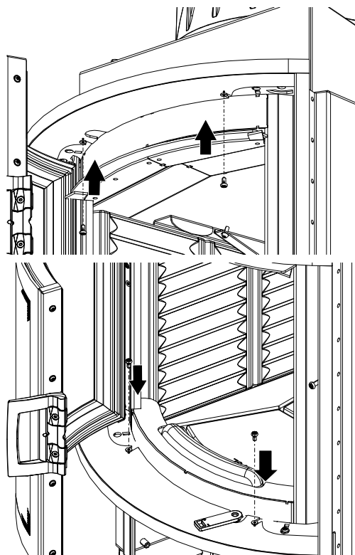
Fig. 87: Fixer le cadre design
