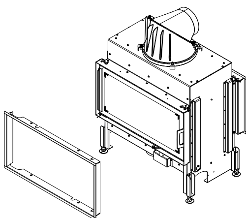
Fig. 88: Positionner le cadre design
