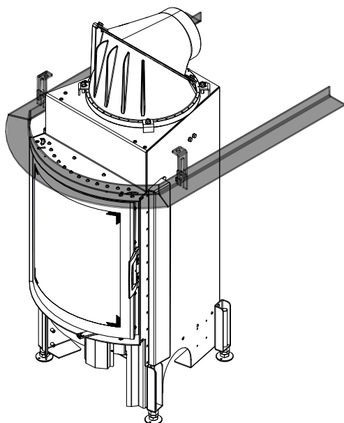
Fig. 96: Installer le cadre porteur
