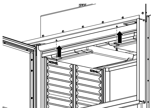
Fig. 93: Fixer le cadre design en haut
