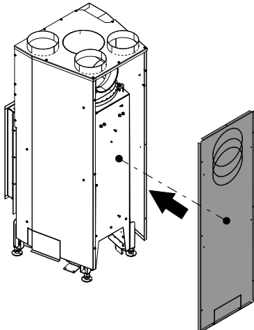
Fig. 70: Installer la paroi de convection arrière
