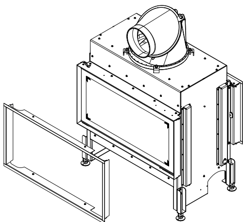
Fig. 91: Positionner le cadre design au dos
