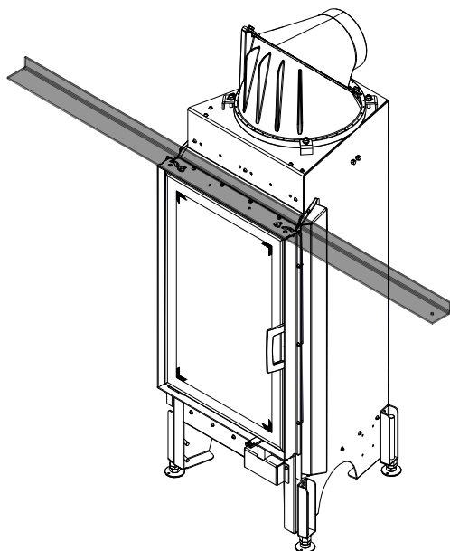
Fig. 95: Installer le cadre porteur
