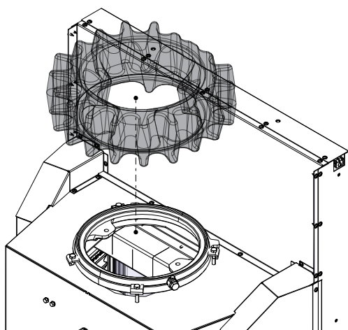
Fig. 31: Poser l'anneau d'accumulation
