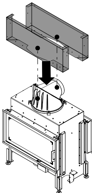
Fig. 75: Installer les parois de convection supérieures (avant + arrière)
