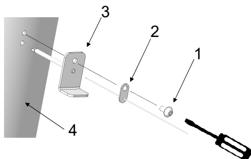
Fig. 49: Installer la sonde de température
