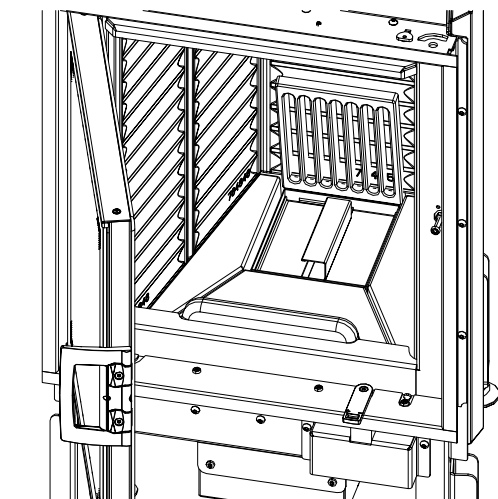
Fig. 107: Fermer le couvercle
