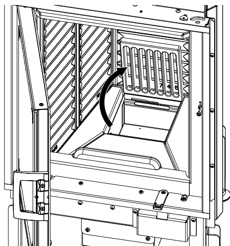
Fig. 105: Extraire ou relever grille
