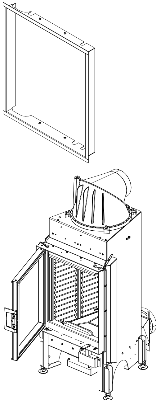
Fig. 80: Ouvrir la porte
