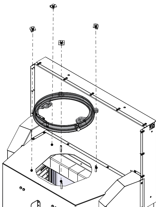
Fig. 29: Installer l'anneau de fixation inférieur
