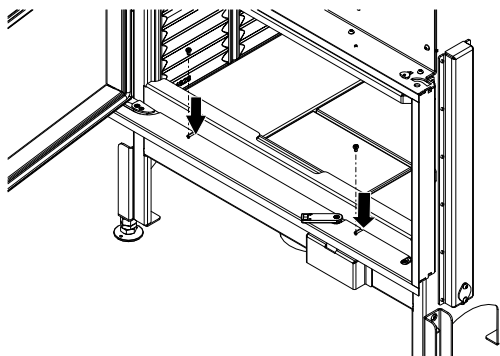
Fig. 90: Fixer le cadre design en bas
