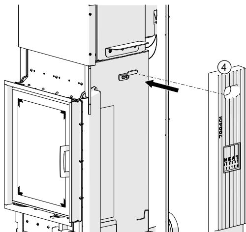
Fig. 27: Poser la pierre HMS
