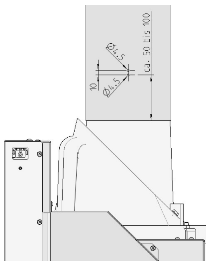
Fig. 48: Schéma de perçage pour conduit de fumée
