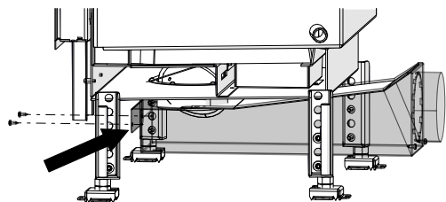
Fig. 39: Mettre le coude plat en place
