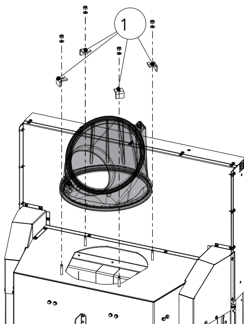
Fig. 28: Déposer l'avaloir de fumées
