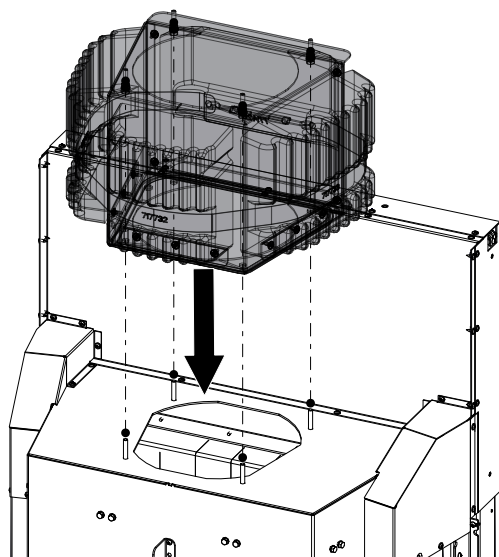
Fig. 36: Poser le grand caisson d'accumulation sur les boulons
