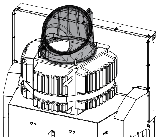
Fig. 36: Poser le grand caisson d'accumulation sur les boulons
