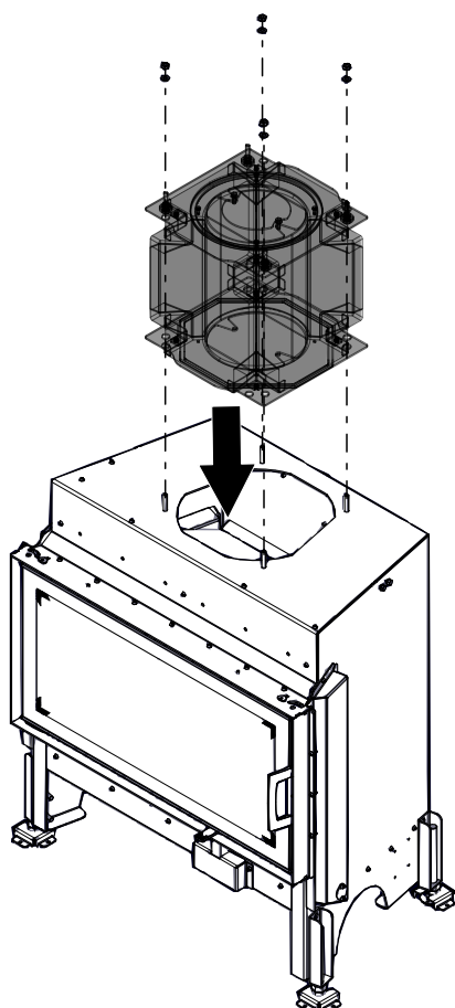
Fig. 43: Poser le petit caisson d'accumulation
