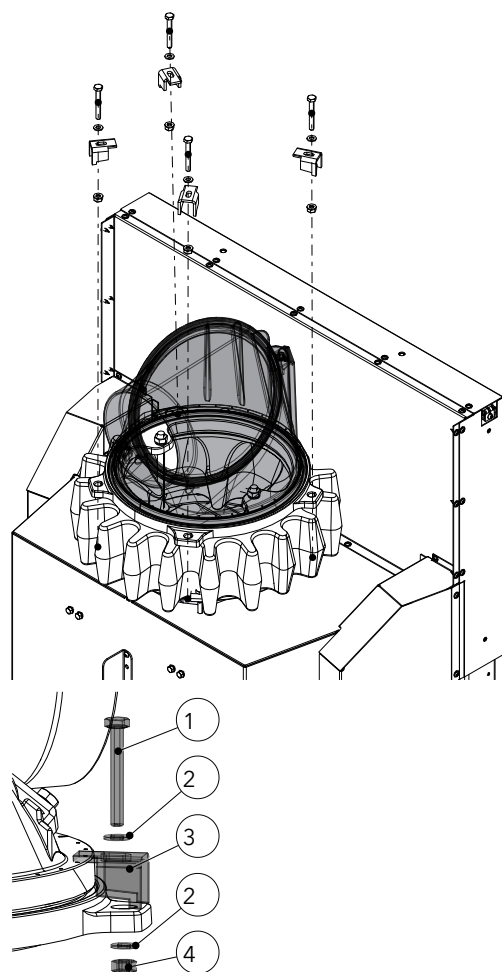
Fig. 34: Installer l'avaloir de fumées
