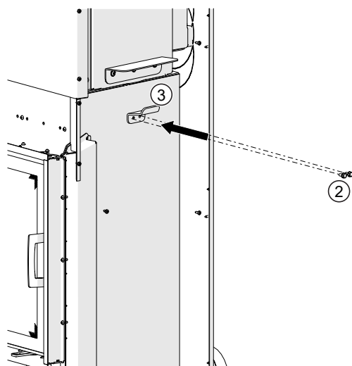
Fig. 26: Installer la fixation HMS
