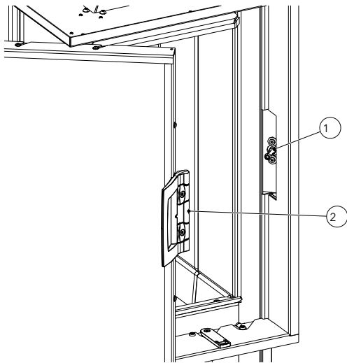
Fig. 100: Régler la porte
