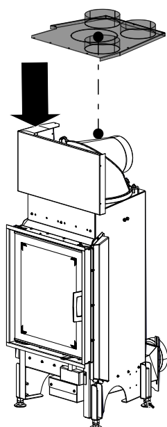
Fig. 67: Installer le couvercle de convection
