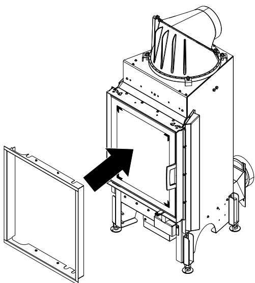
Fig. 83: Poser le cadre design
