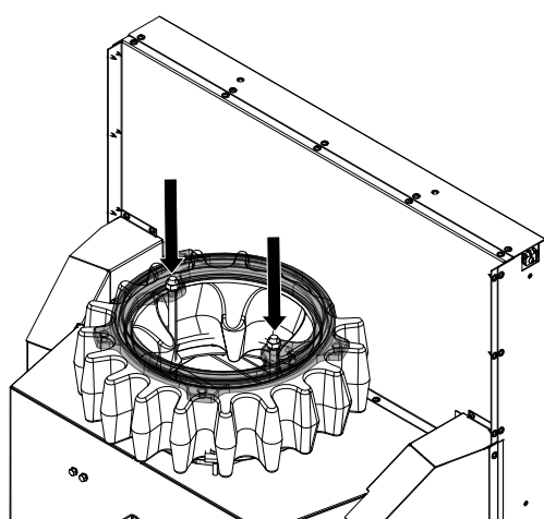
Fig. 33: Fixer l'anneau de fixation supérieur
