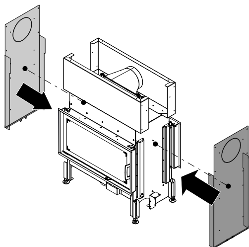
Fig. 76: Poser les parois de convection gauche et droite
