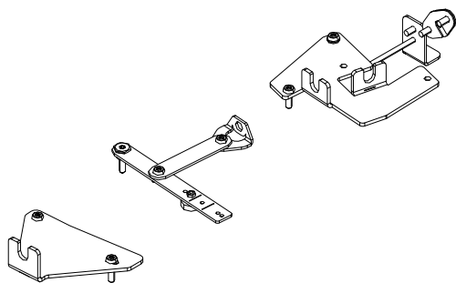
Fig. 46: Kit de montage 363000
