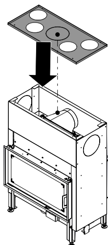
Fig. 78: Installer le couvercle de convection
