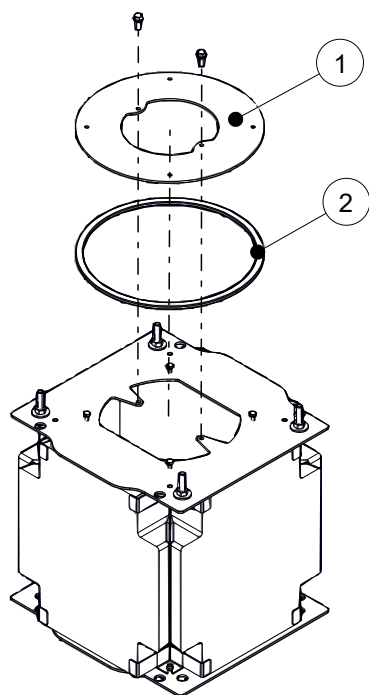
Fig. 41: Enlever le joint et la plaque d'adaptation
