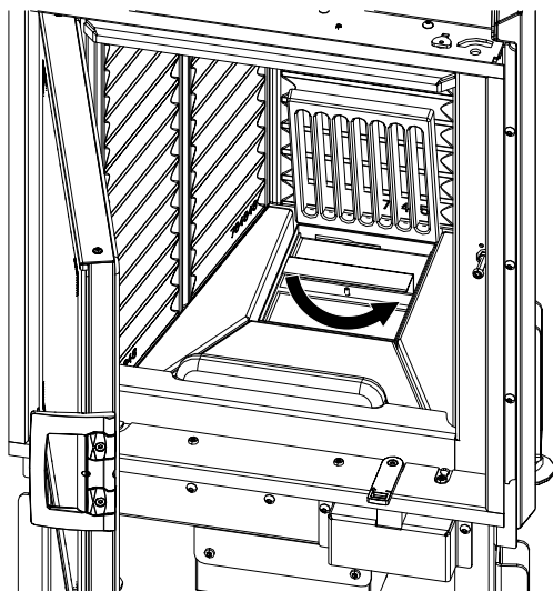
Fig. 106: Mettre le couvercle sur le bac à cendres
