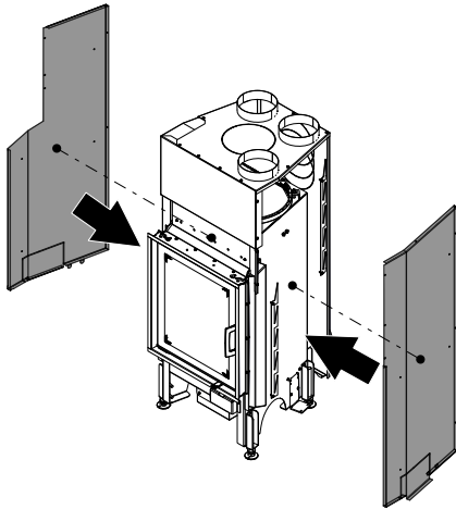
Fig. 68: Poser les parois de convection droite et gauche
