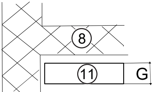
Fig. 11: Plafond au-dessus du foyer
