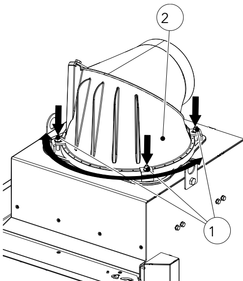
Fig. 101: Orienter l'avaloir de fumées dans la position souhaitée
