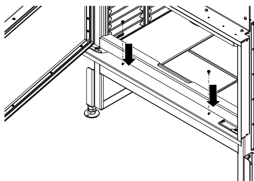
Fig. 94: Fixer le cadre design en bas
