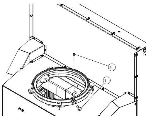
Fig. 30: Fixer la vis ou la sonde
