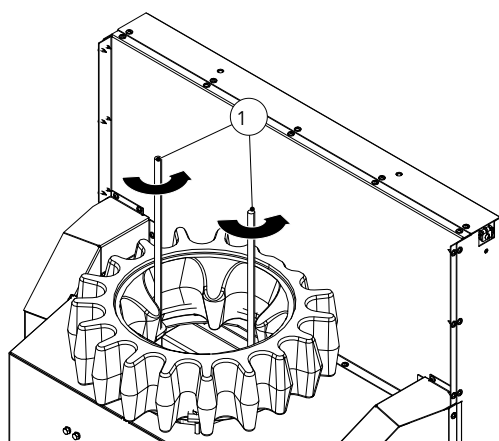
Fig. 32: Installer les tiges filetées
