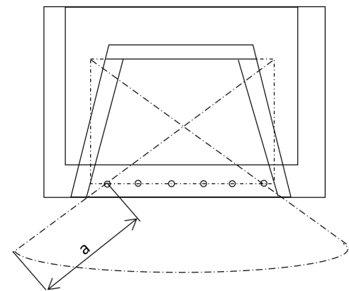
Fig. 12: a : Distance de sécurité
