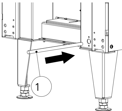
Fig. 56: Enfiler le câble Bowden
