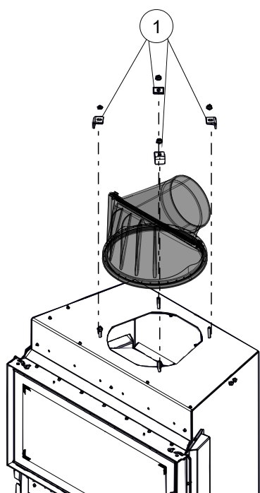
Fig. 42: Déposer l'avaloir de fumées
