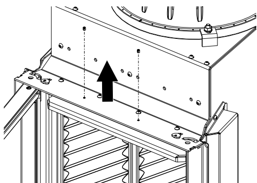
Fig. 81: Dévisser les boulons du haut
