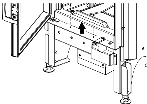
Fig. 82: Dévisser les boulons du bas
