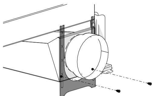
Fig. 40: Installer la fixation
