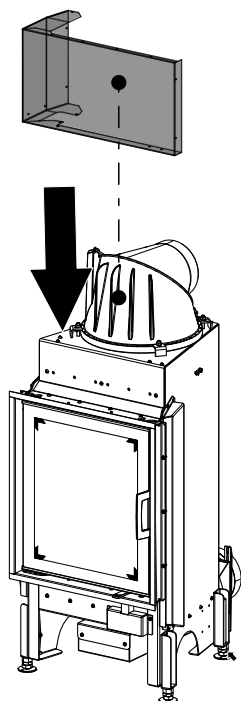
Fig. 66: Installer la paroi de convection avant
