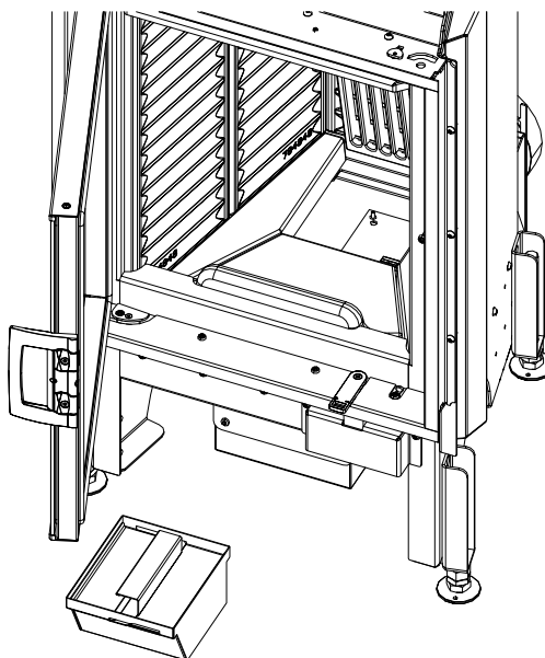
Fig. 108: Enlever et vider le bac à cendres
