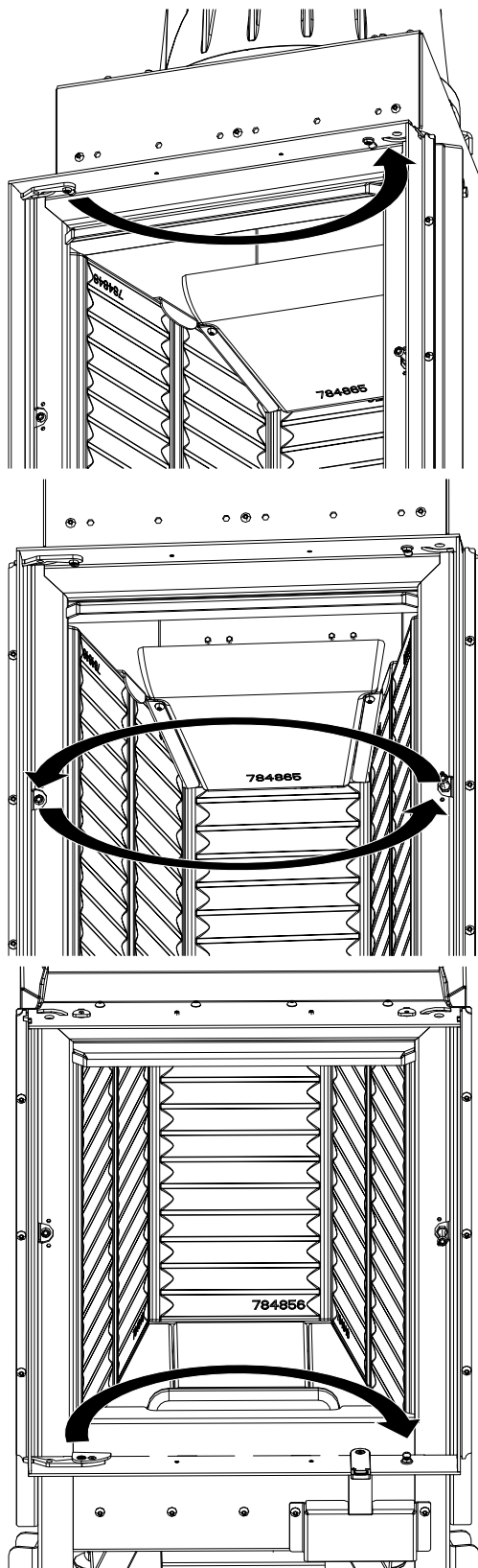
Fig. 22: Changer les vis et logements de charnière de côté
