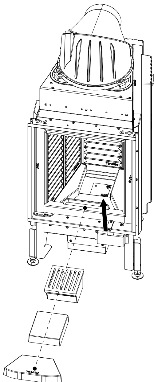
Fig. 97: Mettre le bac à cendres en place
