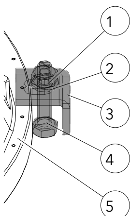
Fig. 44: Installer l'avaloir de fumées
