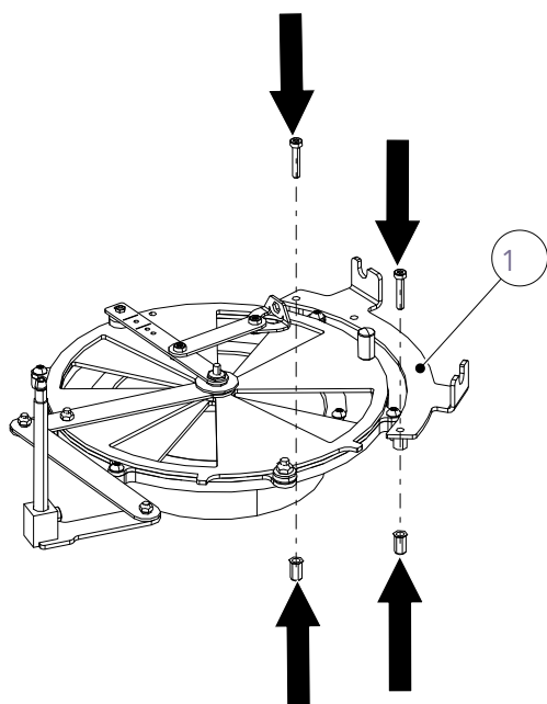
Fig. 54: Installer le kit de montage
