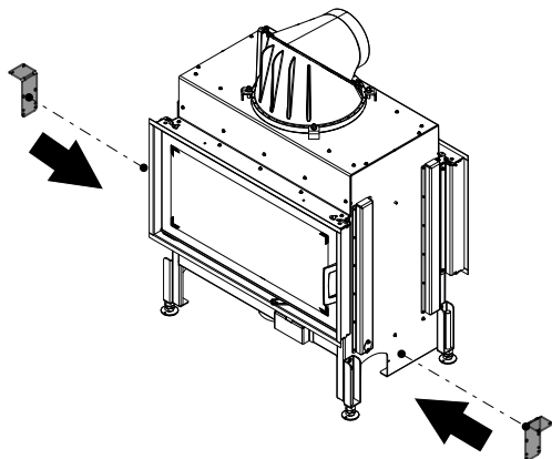
Fig. 72: Installer les fixations gauche et droite
