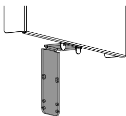
Fig. 77: Enclencher les parois de convection gauche et droite
