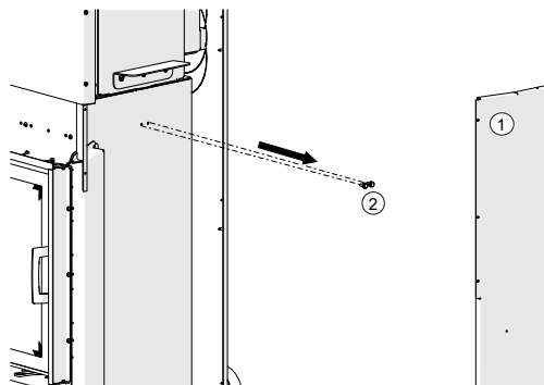
Fig. 25: Démontez le recouvrement et les vis
