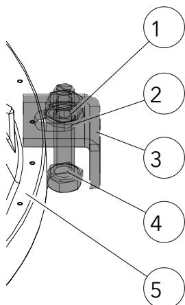
Fig. 37: Installer l'avaloir de fumées
