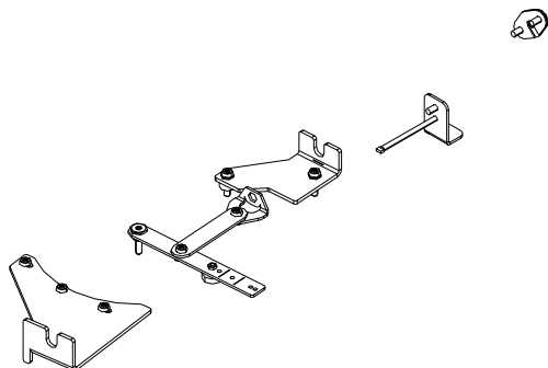
Fig. 47: Kit de montage 363011
