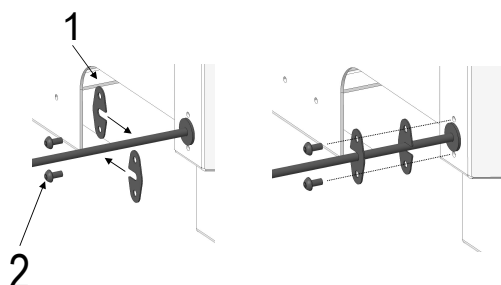
Fig. 59: Brides pour câble Bowden
