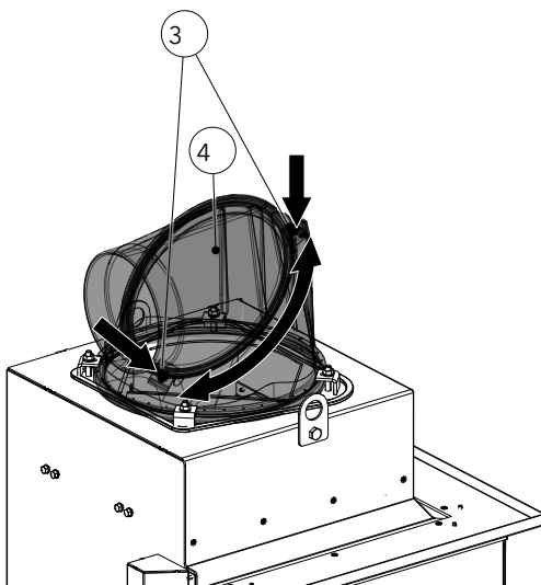
Fig. 102: Régler la buse de l'avaloir de fumées
