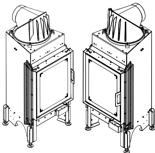
Fig. 50: Perçage pour câble Bowden
