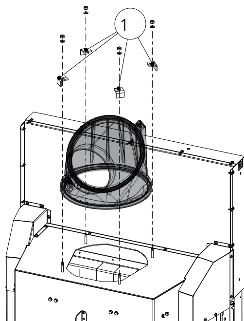
Fig. 35: Déposer l'avaloir de fumées
