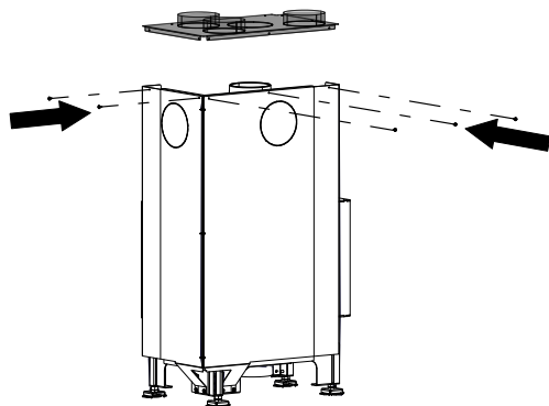
Fig. 71: Fissaggio del coperchio del cappot- to KV
