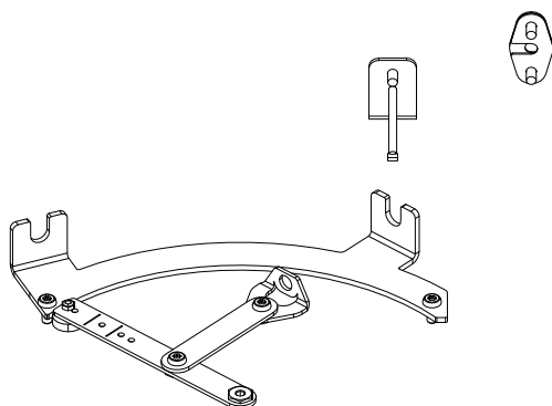
Fig. 52: Kit di montaggio 363004
