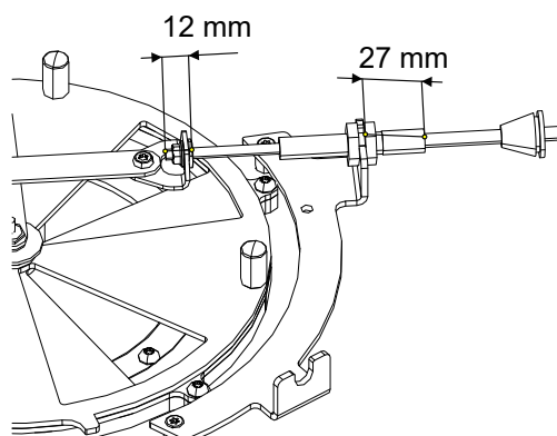
Fig. 63: Collegamento del cavo Bowden
