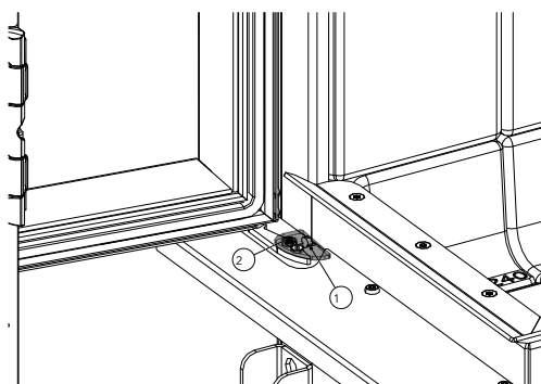
Fig. 78: Regolazione dello sportello in basso
