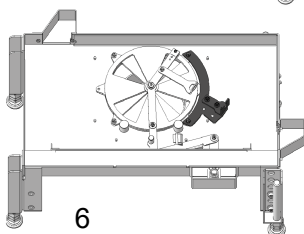
Fig. 56: Montaggio angolo K sx e dx
