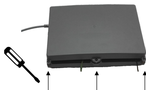
Fig. 66: Scollegamento dell'alimentatore
