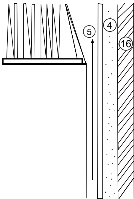
Fig. 8: Cintura di convezione
