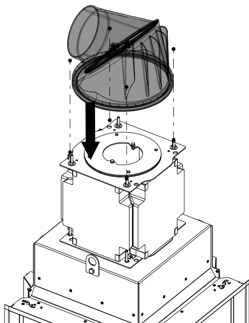
Fig. 41: Collocazione della cassetta sui bulloni
