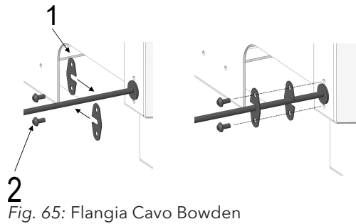
Fig. 65: Flangia Cavo Bowden
