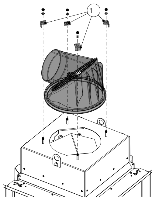
Fig. 40: Smontaggio del collettore dei fumi
