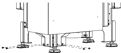
Fig. 68: Avvitare leggermente le viti SK.
