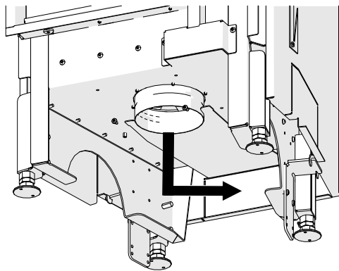
Fig. 5: Raccordo per l'aria comburente
