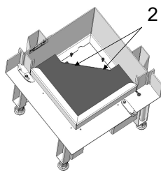
Fig. 57: Smontaggio dei pezzi 38x
