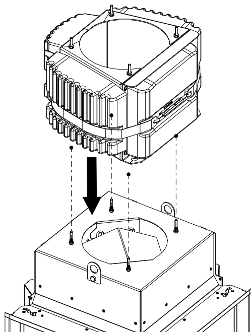
Fig. 38: Poser le grand caisson d'accumulation sur les boulons
