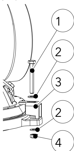
Fig. 49: Installer l'avaloir de fumées
