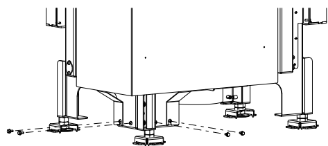
Fig. 50: Visser légèrement les vis hexagonales.
