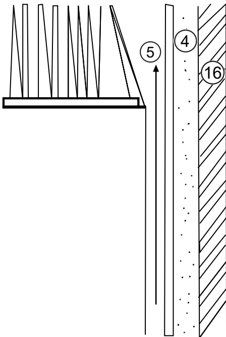
Fig. 8: Espace de convection
