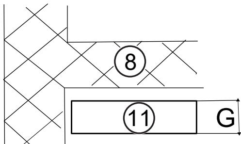
Fig. 12: Plafond au-dessus du foyer
