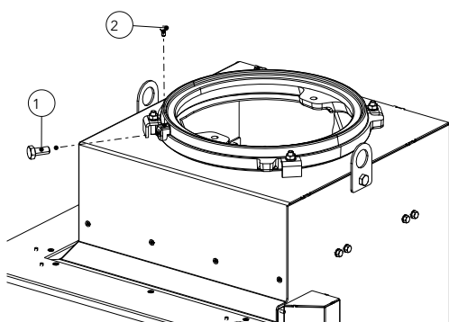
Fig. 45: Fixer la vis ou la sonde
