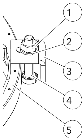
Fig. 42: Installer l'avaloir de fumées sur le caisson d'accumulation
