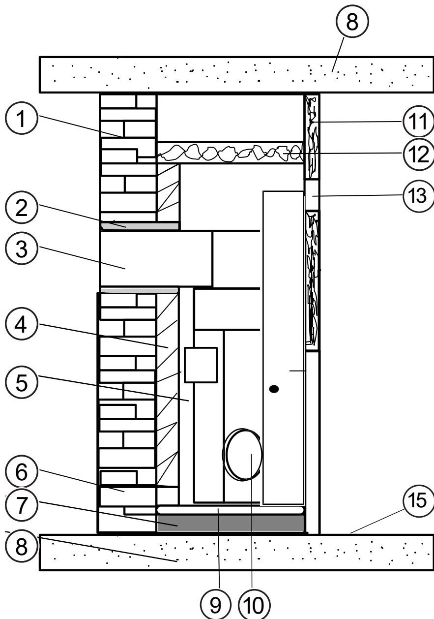
Fig. 6: Construction devant / à côté d'un mur à protéger
