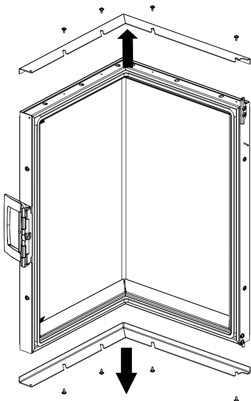
Fig. 27: Déposer les parcloses
