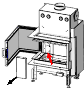
Fig. 2: Plaque signalétique pour appareils en angle
