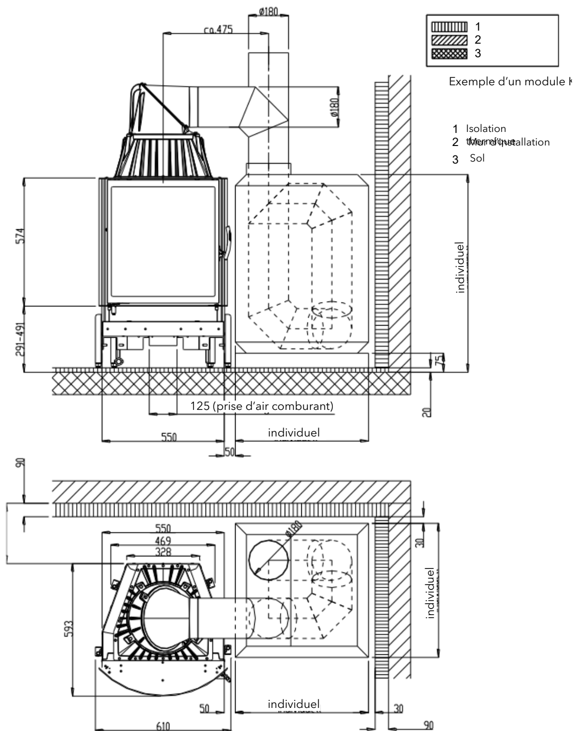
Fig. 15: Système KMS
