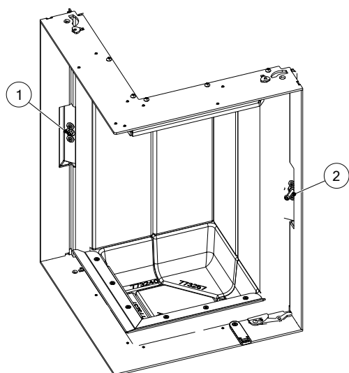
Fig. 30: Interchanger/ajuster les pièces
