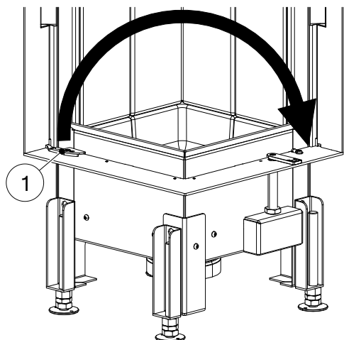
Fig. 26: Changer les recouvrements de côté
