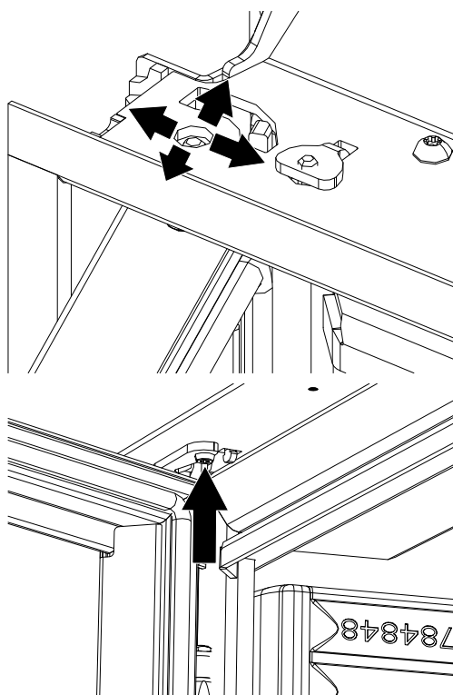
Fig. 57: Régler la porte
