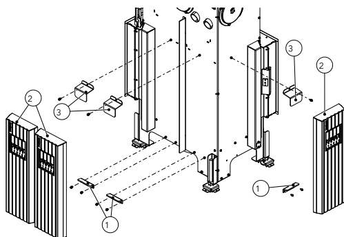
Fig. 36: Installer l'HMS 63x40x42
