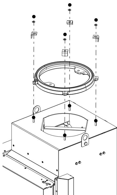
Fig. 44: Installer l'anneau de fixation inférieur
