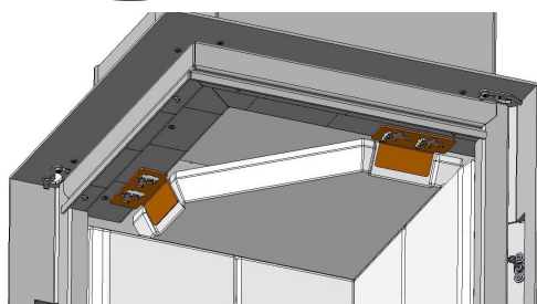
Fig. 19: Déflecteurs pour 55x55x
