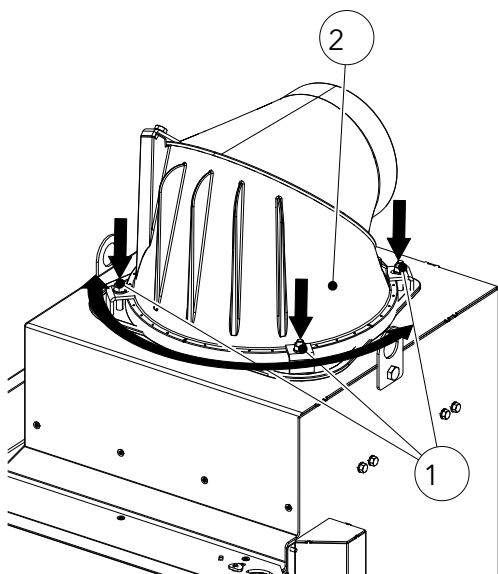
Fig. 60: Orienter l'avaloir de fumées dans la position souhaitée
