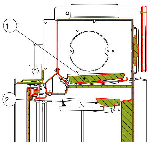
Fig. 18: Déflecteurs pour 38x38x57
