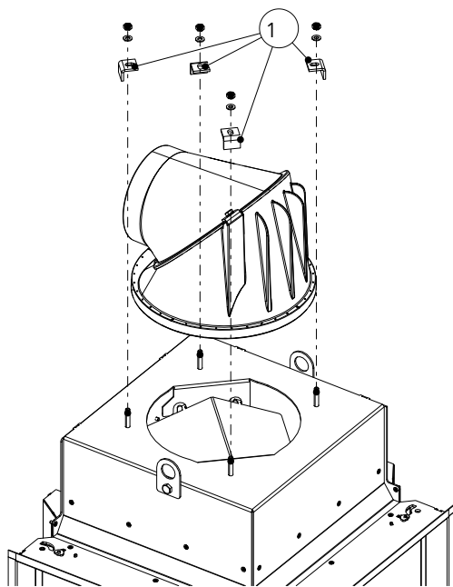
Fig. 40: Déposer l'avaloir de fumées
