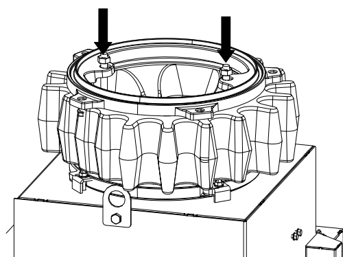
Fig. 48: Fixer l'anneau de fixation supérieur
