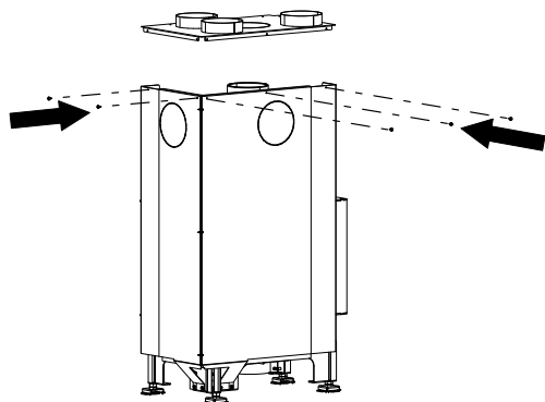
Fig. 53: Fixer le couvercle du kit de convection
