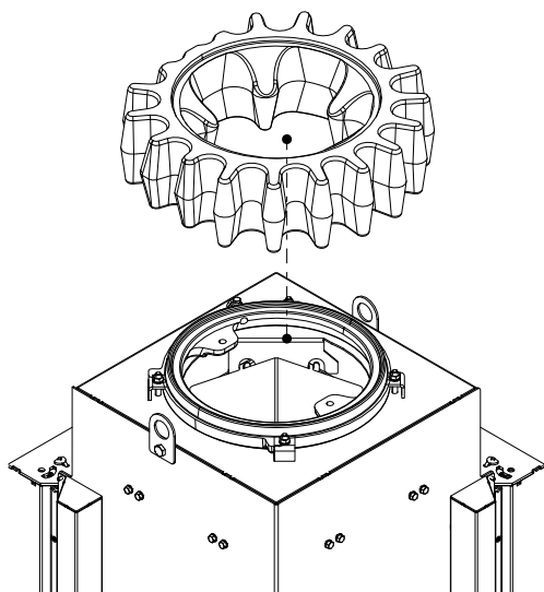
Fig. 46: Poser l'anneau d'accumulation
