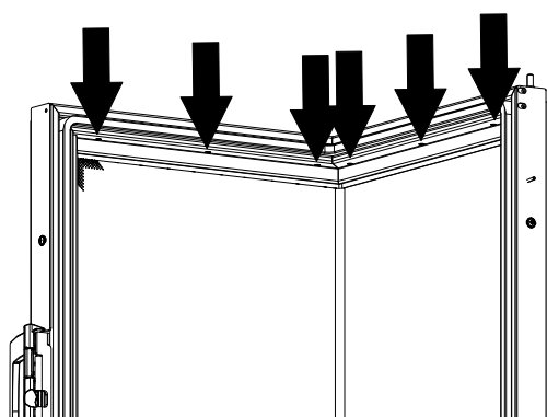
Fig. 28: Dévisser les vis sans tête
