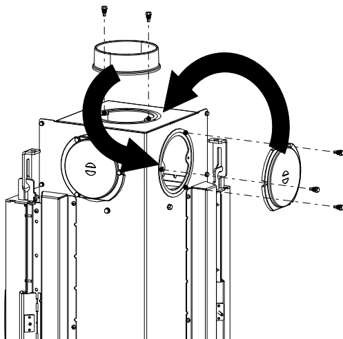
Fig. 32: Interchanger les pièces
