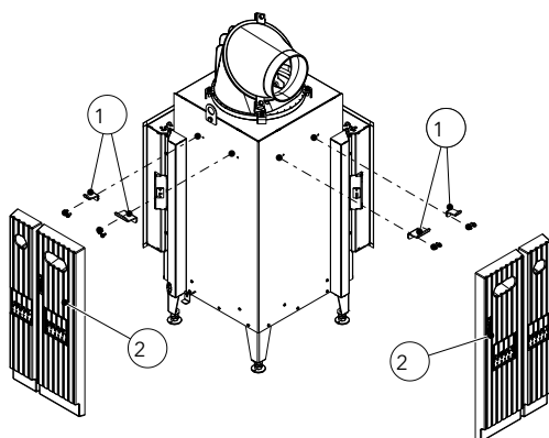
Fig. 35: Installer l'HMS 55x55x K
