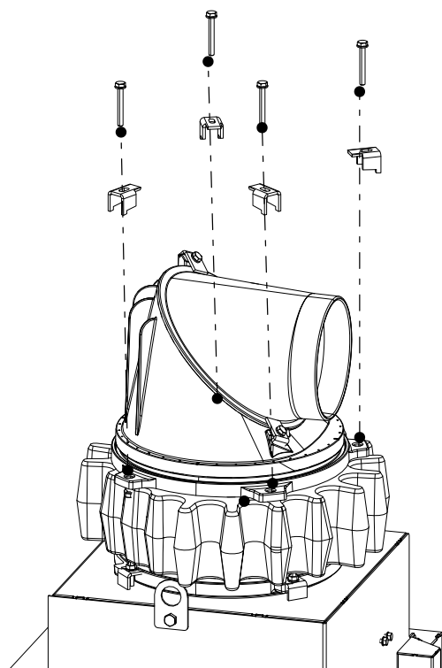
Fig. 48: Fixer l'anneau de fixation supérieur
