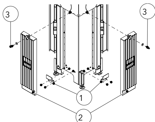
Fig. 34: Installer l'HMS 38x38x57 K
