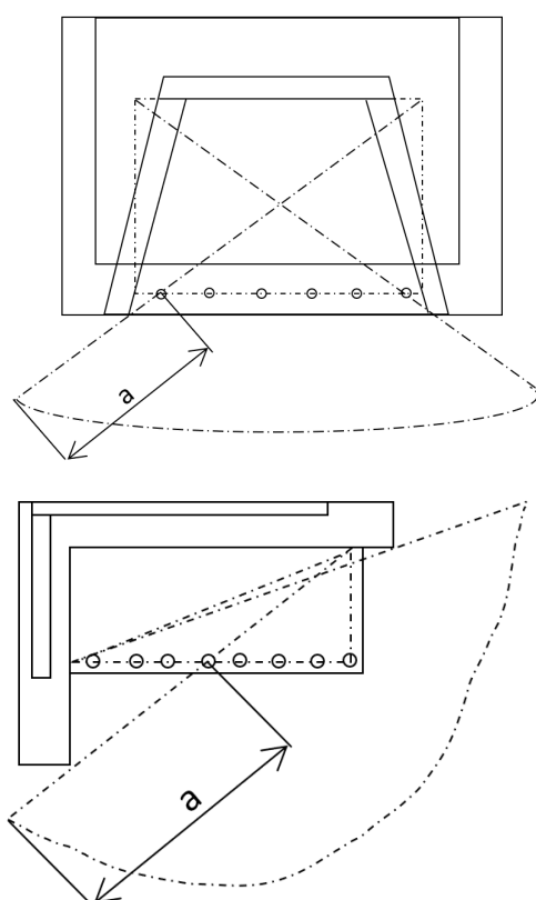
Fig. 1: Cotes « a » selon Données techniques (Distance de sécurité avant)
