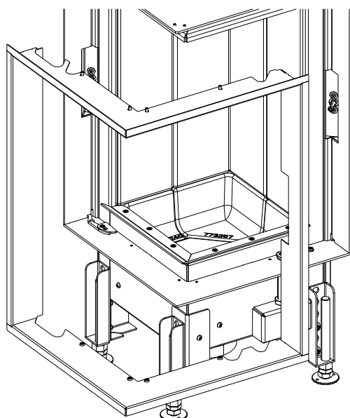
Fig. 56: Poser et fixer le cadre design
