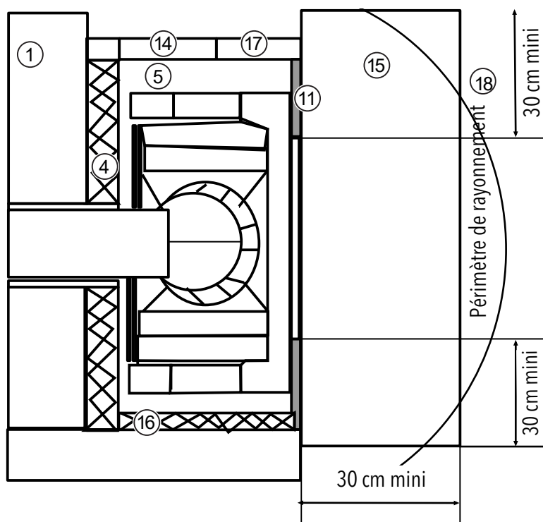
Fig. 7: Construction devant / à côté d'un mur à protéger
