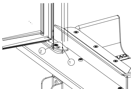
Fig. 58: Régler la porte en bas
