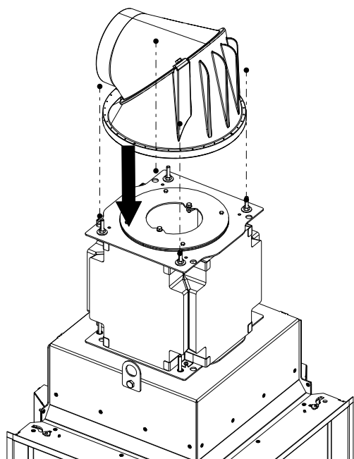
Fig. 41: Poser le petit caisson d'accumulation sur les boulons
