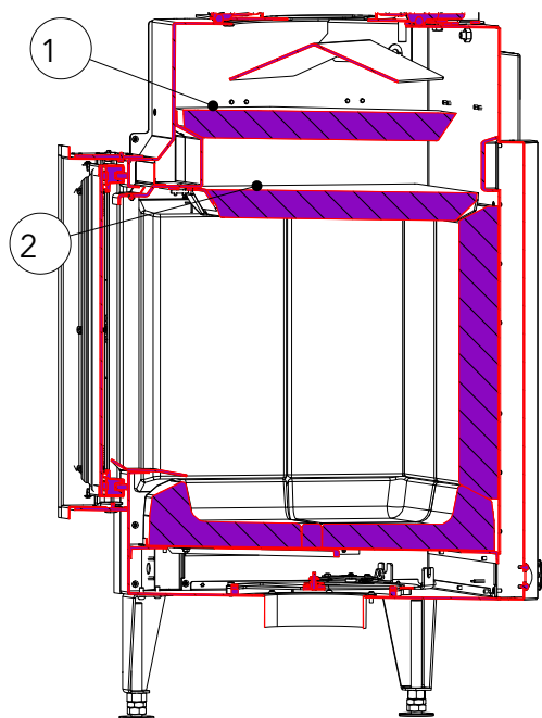
Fig. 18: Déflecteurs pour 38x38x57
