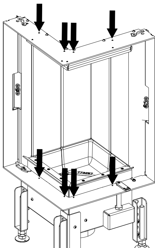
Fig. 55: Dévisser les vis
