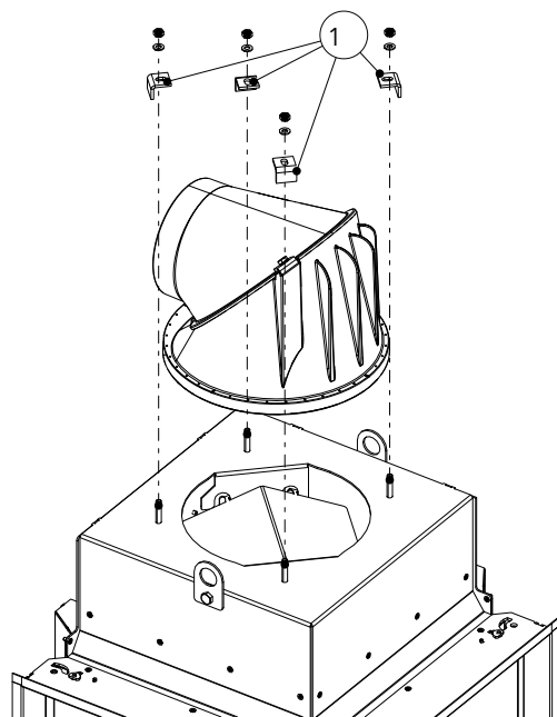
Fig. 43: Déposer l'avaloir de fumées
