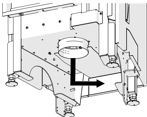
Fig. 5: Buse d'entrée d'air de combustion
