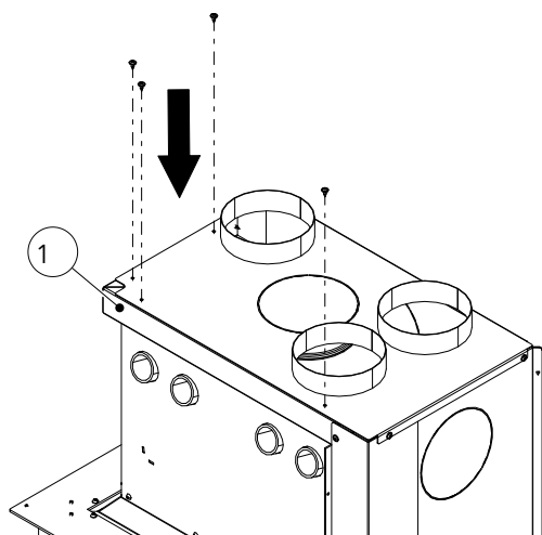
Fig. 54: Installer l'avant du kit de convection
