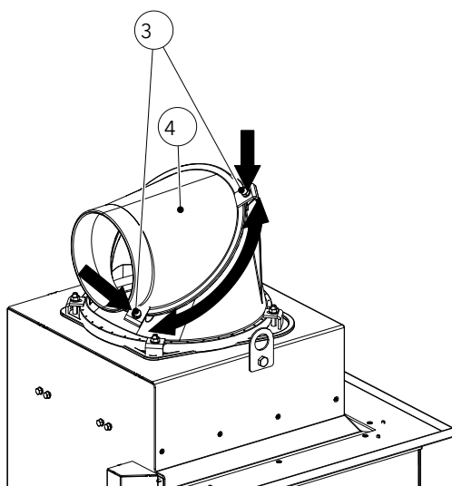
Fig. 61: Régler la buse de l'avaloir de fumées
