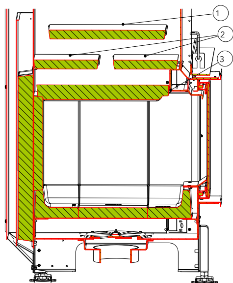
Fig. 20: Plaque déflectrice 63x40x42
