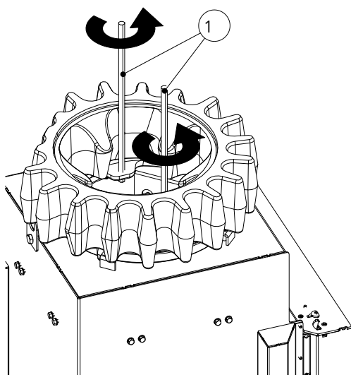
Fig. 47: Installer les tiges filetées
