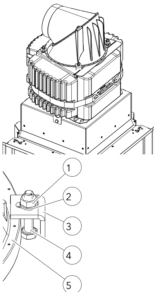
Fig. 39: Installer l'avaloir de fumées
