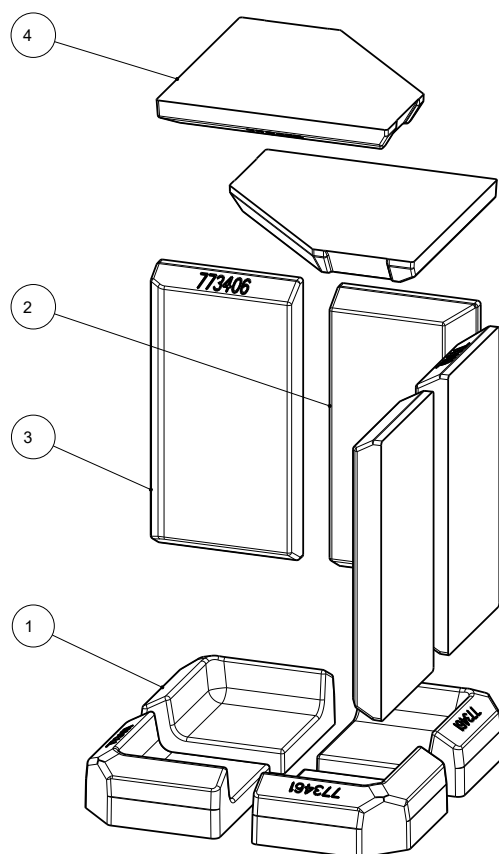
Fig. 22: Keramott 55x55x
