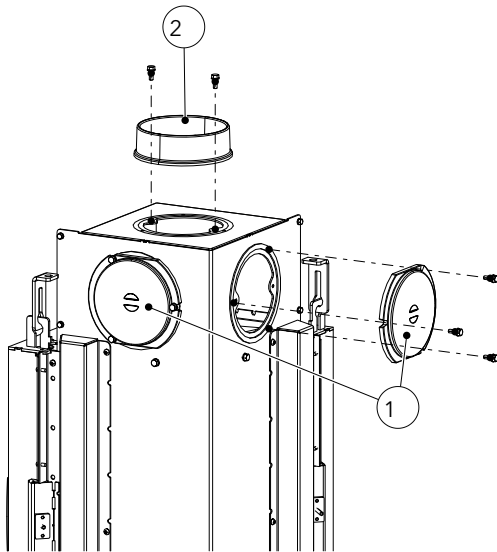
Fig. 31: Démontez le recouvrement et la tubulure de fumées
