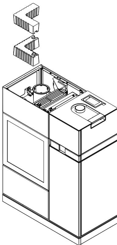
Abb. 2: HMS-Steine anbringen
