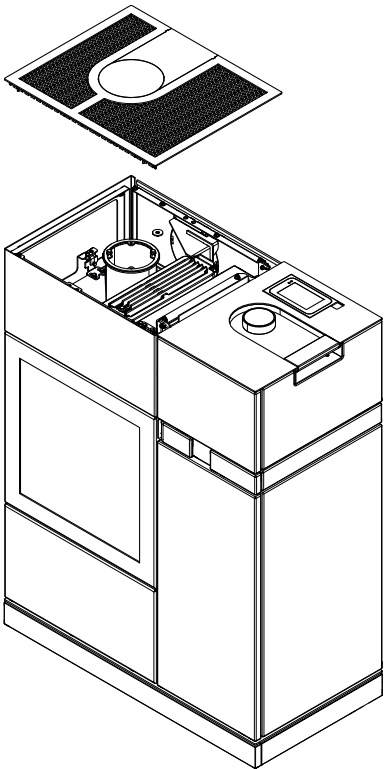
Abb. 1: Deckel abnehmen
