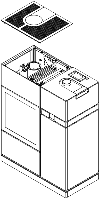
Fig. 1: Enlever le couvercle.
