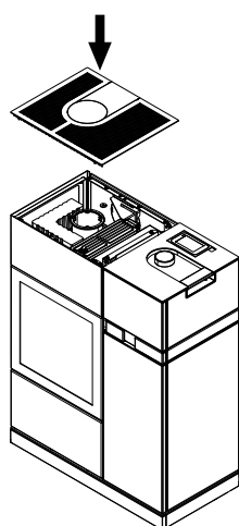
Fig. 3: Poser le couvercle
