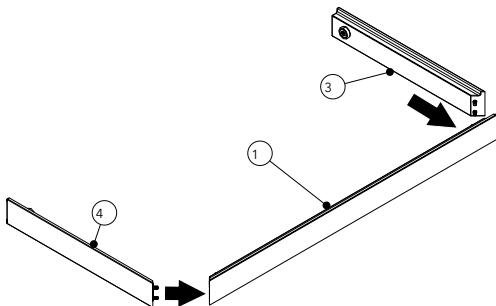
Fig. 9: Assemblare il basamento in legno
