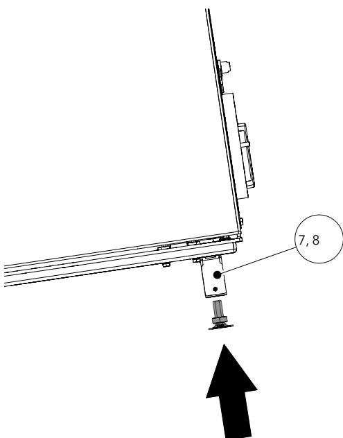
Fig. 4: Installer les pieds de distance
