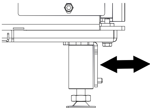
Fig. 8: Régler l'équerre
