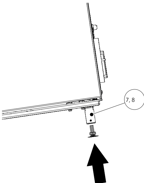
Fig. 4: Montare i piedini regolabili.
