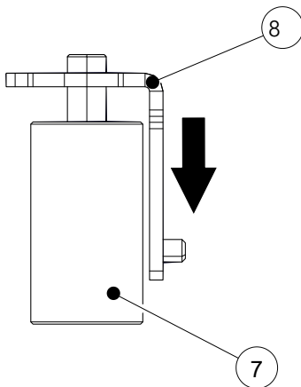
Abb. 3: Winkel und Distanzfuß montieren
