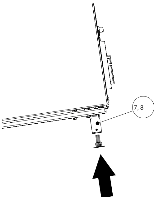
Fig. 7: Montare i piedini regolabili.
