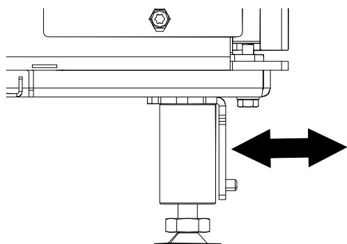
Fig. 5: Régler l'équerre
