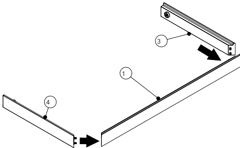
Abb. 9: Holzsockel zusammenstecken
