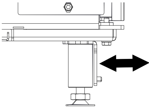
Abb. 8: Winkel einstellen
