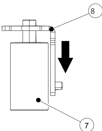
Fig. 3: Installer équerre et le pied de distance
