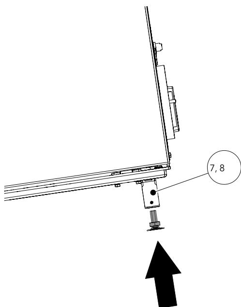
Fig. 7: Installer les pieds de distance
