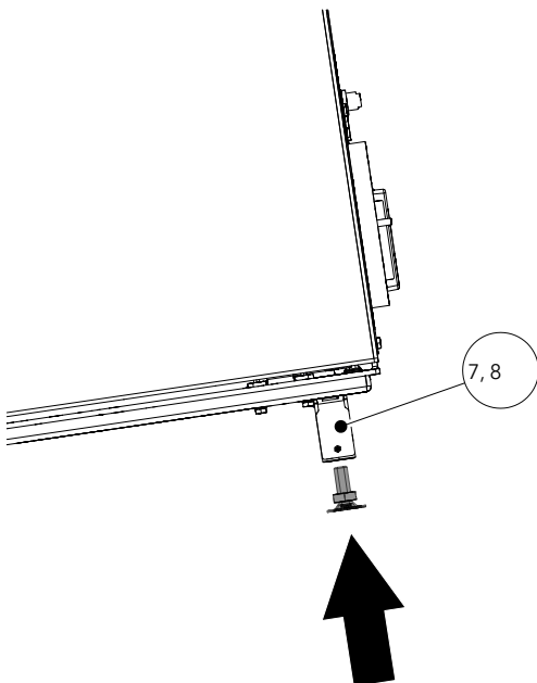
Abb. 4: Stellfüße montieren
