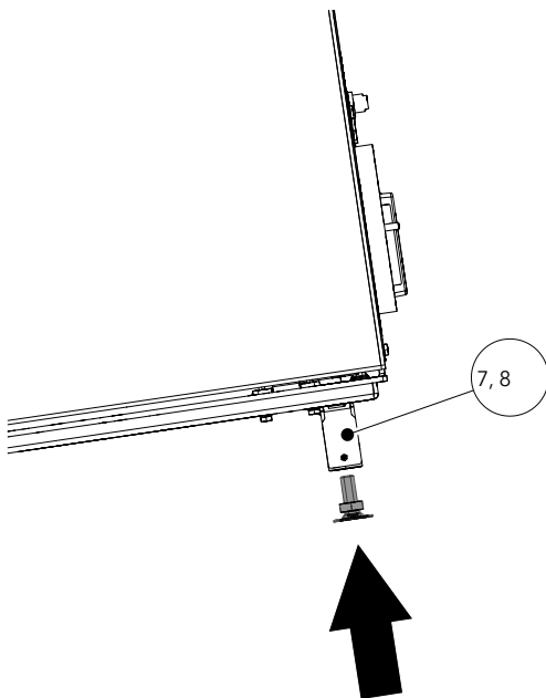
Abb. 7: Stellfüße montieren
