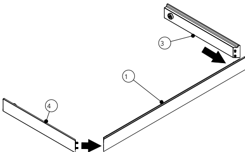
Fig. 9: Assembler le socle en bois
