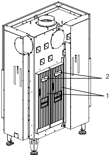
Abb. 1: HMS montieren
