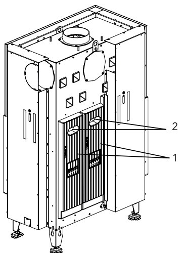
Fig. 1: Montaggio dell'HMS
