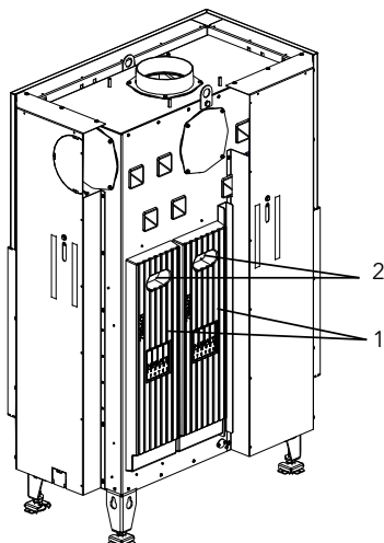
Fig. 1: Installer l'HMS
