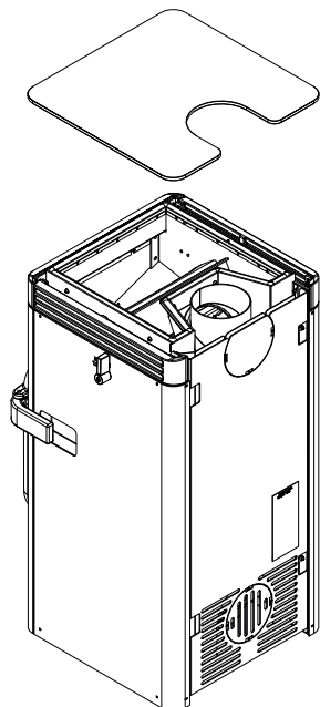
Abb. 1: Herdplatte anbringen
