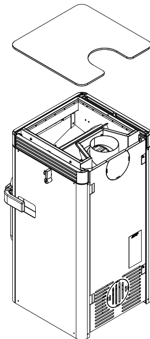
Fig. 1: Collocazione del piano cottura
