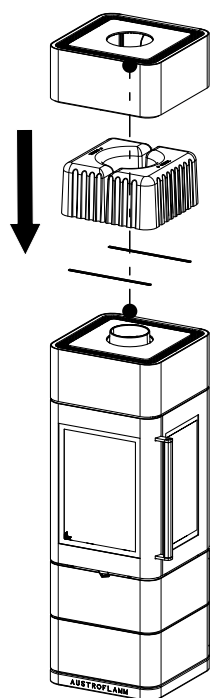
Fig. 1: Montaggio dell'HMS
