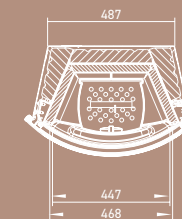
Abb. rechts: Fynn Xtra mit Keramikverkleidung in Turmaline
