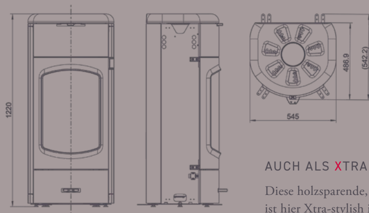
Zeichnung: Meron Xtra
