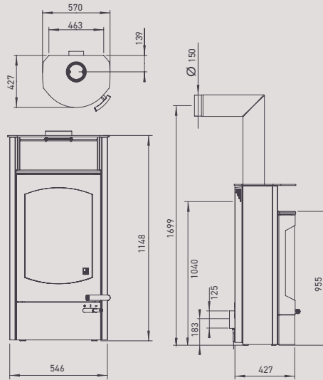
Koko 2.0 avec compartiment chauffe-plat en pierre ollaire
