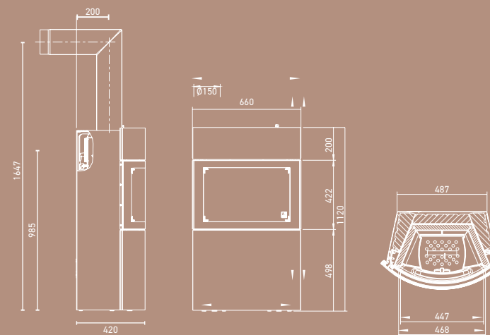
Fig. de droite : Fynn Xtra avec revêtement en céramique tourmaline
