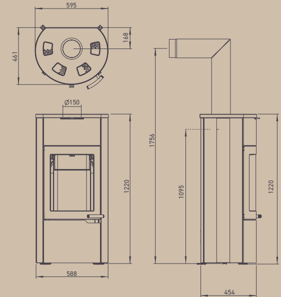
Le Uno Xtra avec enveloppe et couvercle en pierre ollaire et ses ouvertures de convection réglables.
