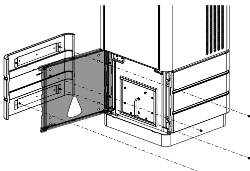
Abb. 13: vordere Keramikverkleidung montieren
