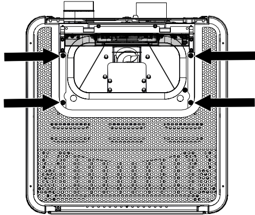
Abb. 9: Schrauben lösen
