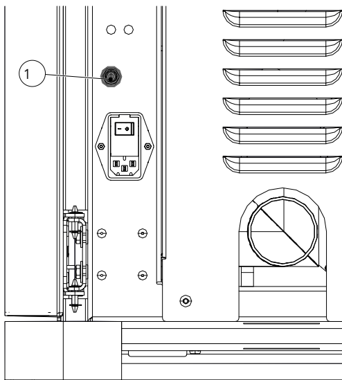
Abb. 78: Sicherheitstemperaturbegrenzer
