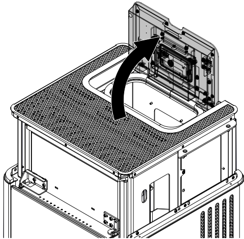
Abb. 8: Tank öffnen
