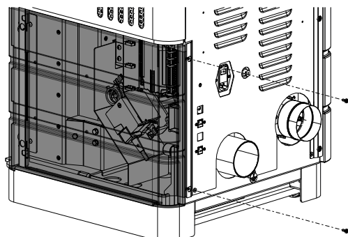
Abb. 12: Seitenteile befestigen
