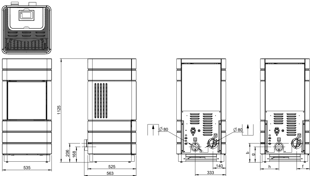
Abb. 2: Abmessungen
