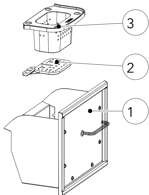
Abb. 65: Kipprost reinigen
