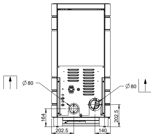
Abb. 28: Abmessungen
