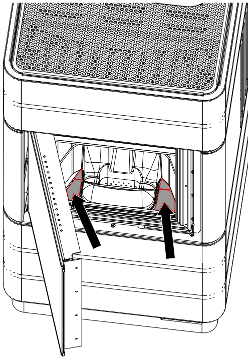
Abb. 71: Feuerraum reinigen
