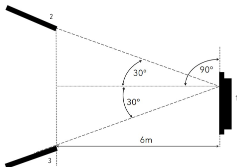
Abb. 38: Betriebswinkel
