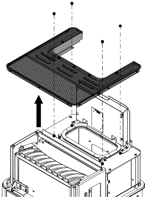
Abb. 10: Deckel abnehmen
