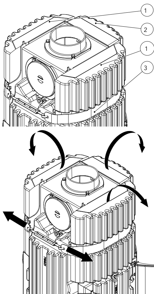
Fig. 48: Rimozione della cinghia di fissaggio e delle pietre HMS superiori
