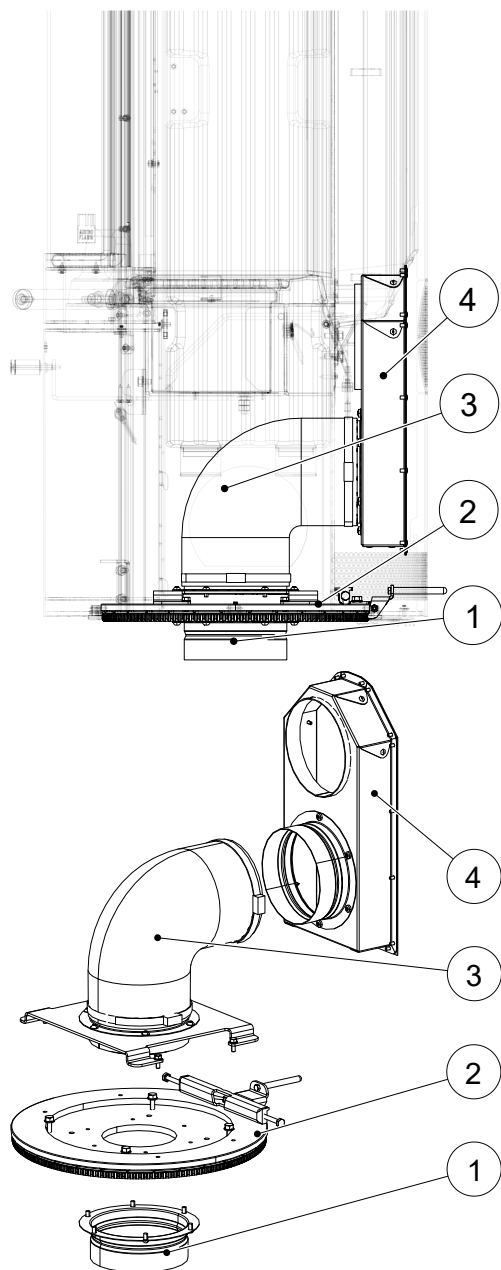
Fig. 36: Montaggio della connessione dell'aria esterna nella parte inferiore
