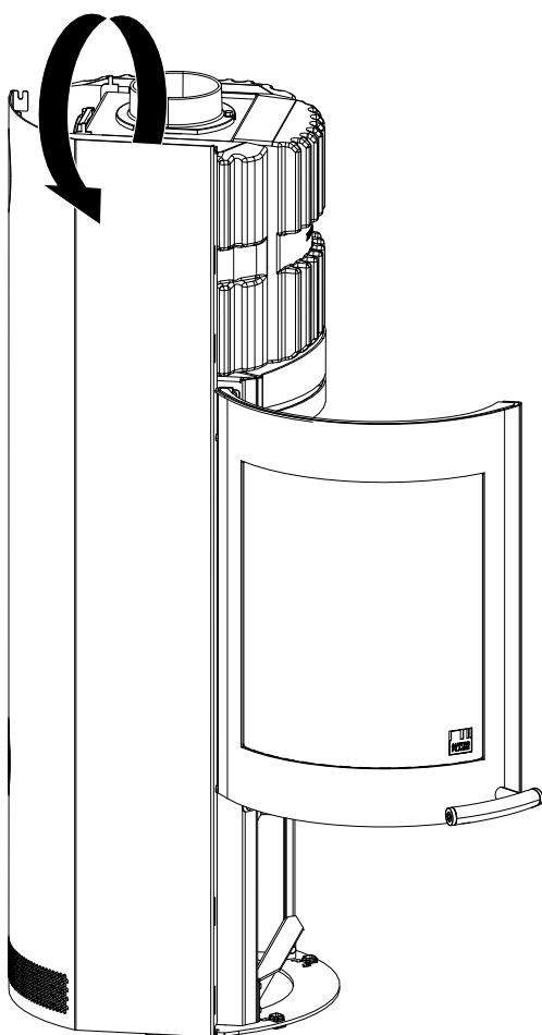
Fig. 20: Rimozione del rivestimento laterale sinistro
