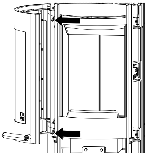
Fig. 19: Svitamento delle viti della porta
