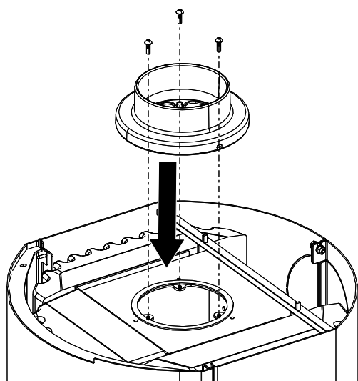
Fig. 34: Montaggio del giunto girevole
